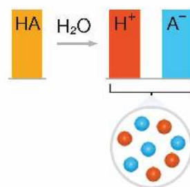
Rys. 60. Dysocjacja mocnego kwasu jednoprotowego.
