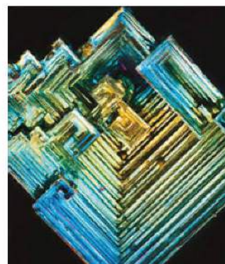
Fot. 151. Bizmut.
