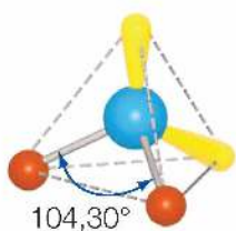
Rys. 43. Przestrzenna budowa cząsteczki wody.
