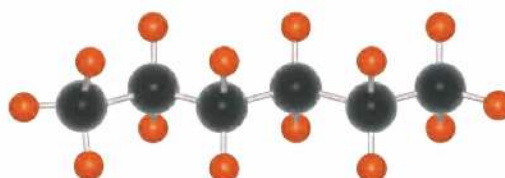
heksan
