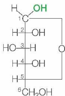
wzór Fischera
