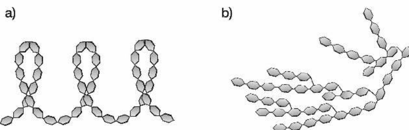
Rys. 18. Schemat budowy cząsteczek: a) amylozy, b) amylopektyny.
