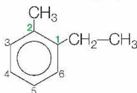
1-etylo-2-metylobenzen
