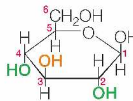
wzór Hawortha
