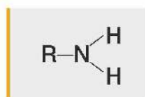
amina pierwszorzędowa
