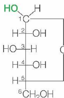
wzór Fischera
