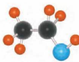
etan ol
