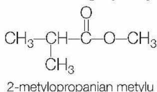
łańcuch rozgałęziony
