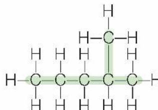
łańcuch rozgałęziony
