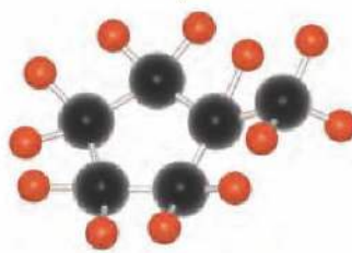
metylocyklopentan
