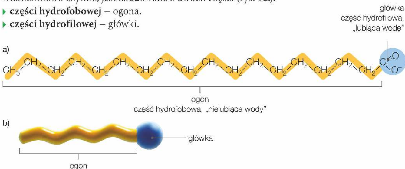
Rys. 12. Jon stearynianowy: a) wzór półstrukturalny, b) model.
