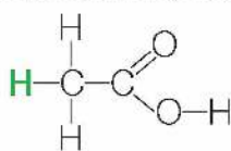
kwas karboksylowy
