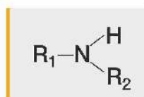
amina drugorzędowa
