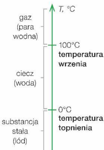
Rys. 3. Stany skupienia wody w zależności od temperatury.
