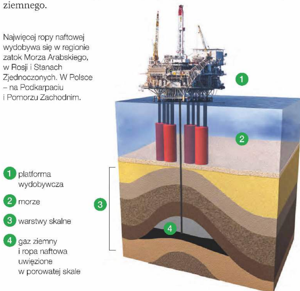
Rys. 6. Ropę naftową wydobywa się z pokładów znajdujących się na głębokości kilku kilometrów pod powierzchnią lądu lub dna morskiego.
