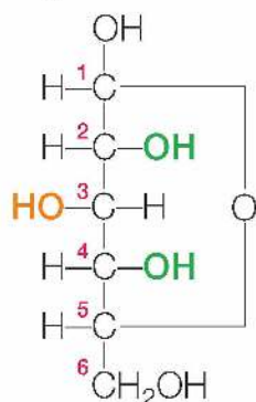
wzór pierścieniowy
