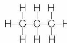
wzór strukturalny propanu
