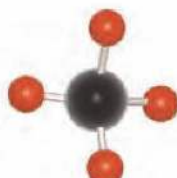
metan
