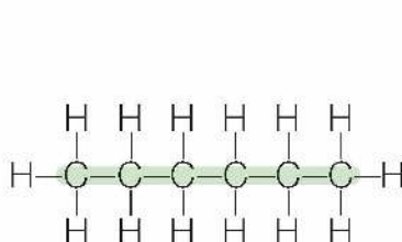
łańcuch prosty
