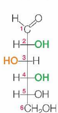
wzór Fischera
