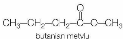
łańcuch prosty
