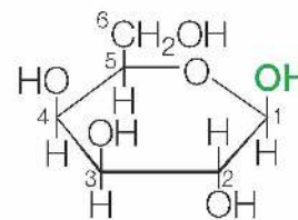
wzór Hawortha
