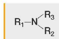
amina trzeciorzędowa
