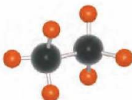
etan
