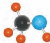
metan ol
