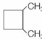
1,2-dimetylocyklobutan
