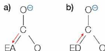
Rys. 43. Kierunek przemieszczania się elektronów w anionie karboksylanowym podstawionym: a) stabilizującą grupą elektronoakceptorową, b) destabilizującą grupą elektronodonorową.
