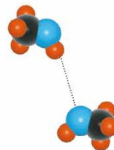
Rys. 35. Model wiązania wodorowego między polarnymi cząsteczkami metanolu.
