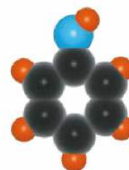
Rys. 38. Model cząsteczki najprostszego fenolu – benzenolu.
