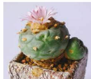
Fot. 122. Meskalina – związek chemiczny, który znajduje się w tej roślinie – jest trująca.
