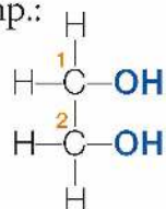
etano-1,2-diol
