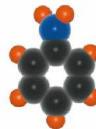
Modele atomów:
