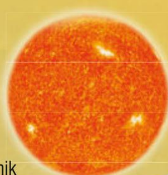
powierzchnia Słońca
