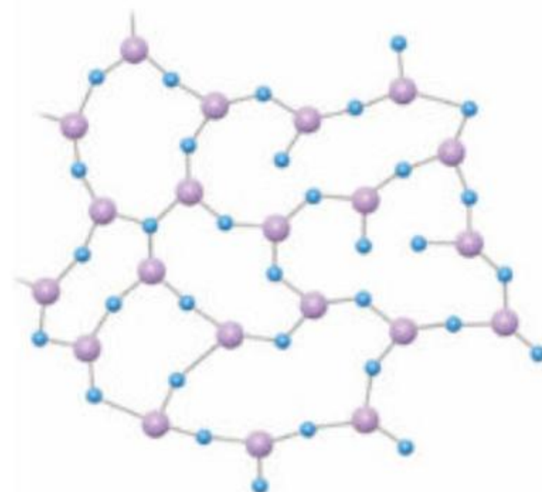
Cząsteczki szkła.
