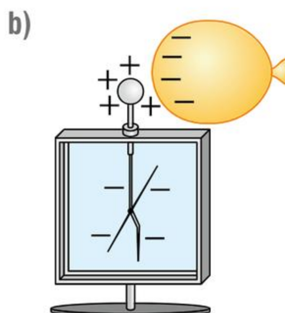
Do kulki elektroskopu zbliżamy ciało naelektryzowane ujemnie.
