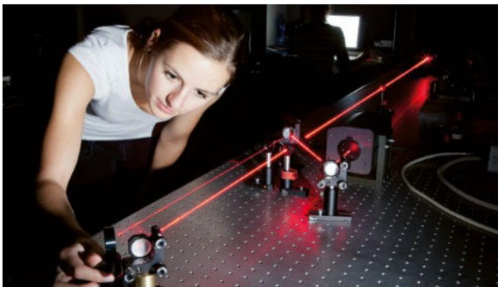
Laser jest źródłem światła wytwarzającym cienką, równoległą wiązkę.
