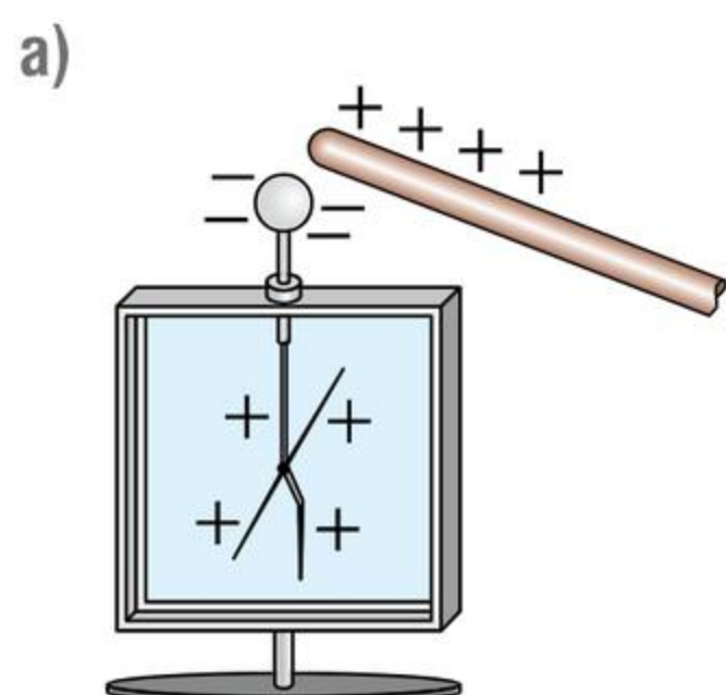
Do kulki elektroskopu zbliżamy ciało naelektryzowane dodatnio.
