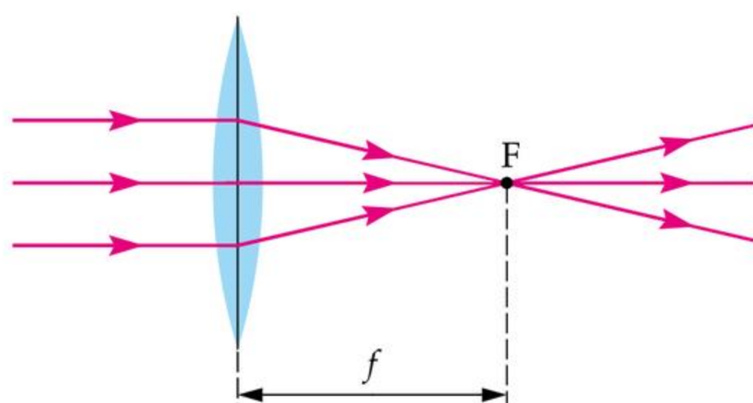
F – ognisko (punkt), f – ogniskowa (odległość)
