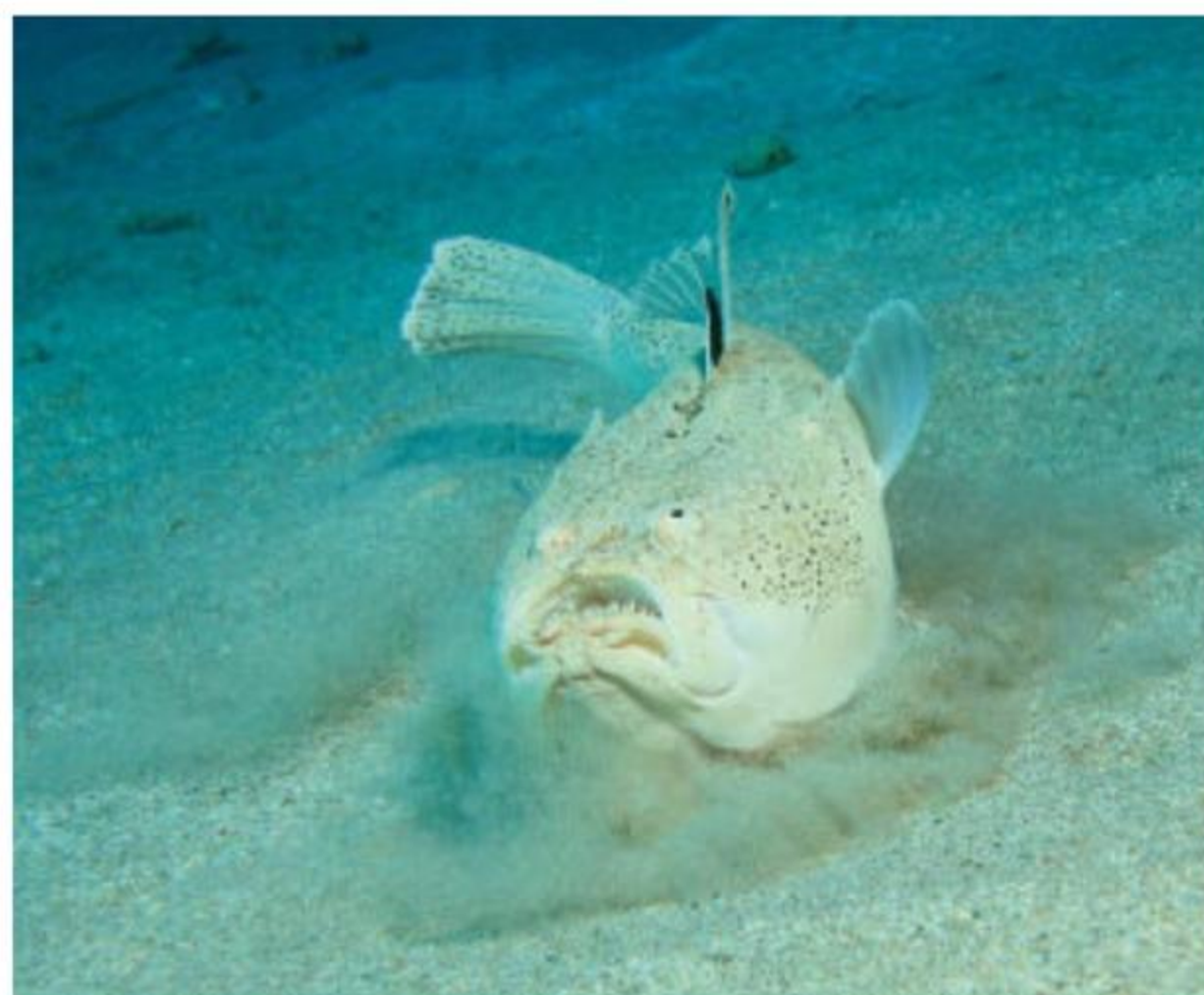
Niektóre skarabierowate są w stanie porazić ofiarę prądem o napięciu dochodzącym do 50 V. Organy elektryczne ryby zlokalizowane są w głowie.
