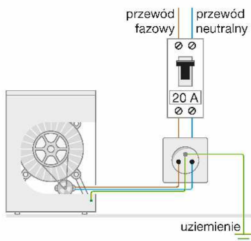
Rys. 15.14. Przewody w gniazdku sieciowym
