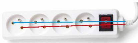
Rys. 13.28. Gniazdka w przedłużaczu – a w konsekwencji podłączone do nich odbiorniki energii – są połączone równoległe
