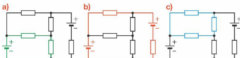
Rys. 13.55. W skomplikowanym obwodzie elektrycznym można wyróżnić wiele oczek
