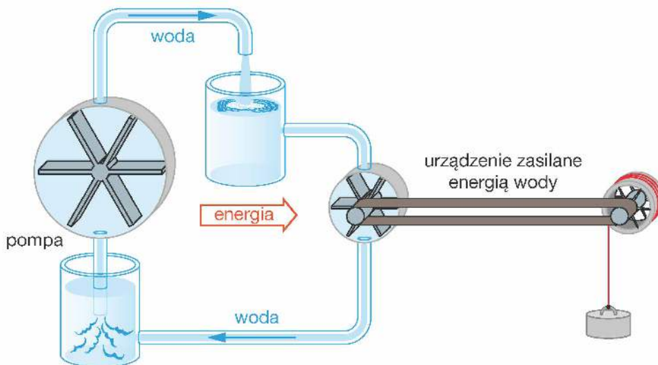
Rys. 13.12. Hydrauliczny odpowiednik obwodu elektrycznego
