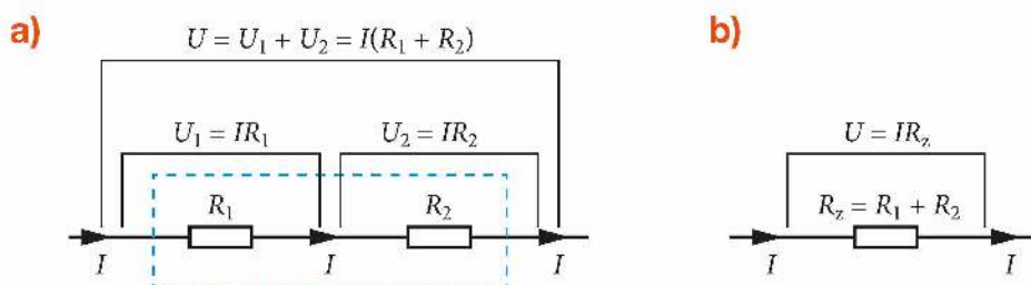
Rys. 13.37. Wyznaczanie oporu zastępczego oporników połączonych szeregowo
