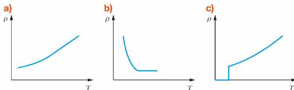
Rys. 13.45. Schematyczny wykres zależności oporu właściwego od temperatury dla: a) przewodnika, b) półprzewodnika, c) nadprzewodnika
