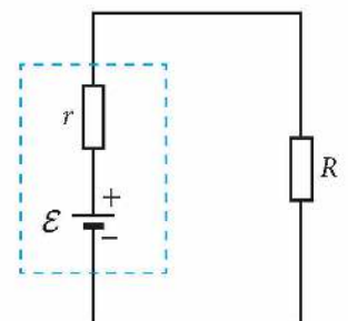
Rys. 13.53. Schemat obwodu z uwzględnieniem oporu wewnętrznego
