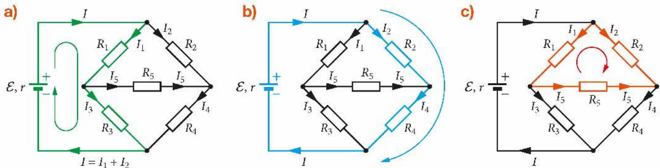
Rys. 13.60. Trzy oczka obwodu wybrane do obliczeń
