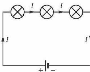
Rys. 13.23. Przy połączeniu szeregowym natężenie prądu I jest takie samo w każdym punkcie obwodu. Takie samo natężenie ma prąd wewnątrz każdej z żarówek i wewnątrz baterii
