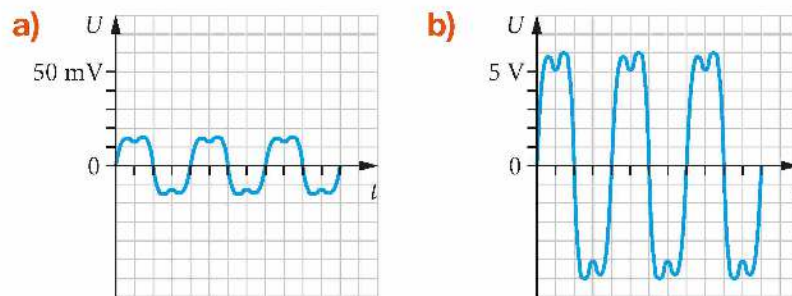
Rys. 15.38. Działanie wzmacniacza: a) sygnał wejściowy, b) sygnał wyjściowy
