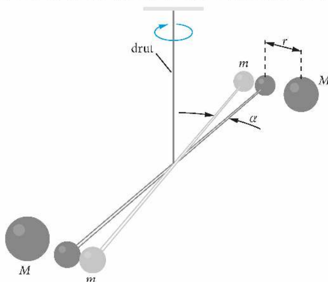
Rys. 11.29. Schemat pomiaru stałej grawitacji w doświadczeniu Cavendisha
