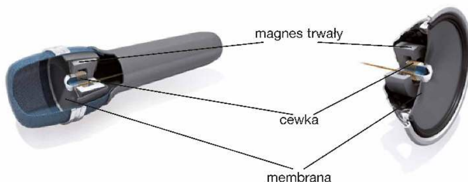
Rys. 15.5. Budowa mikrofonu i głośnika – oba urządzenia mają podobną konstrukcję
