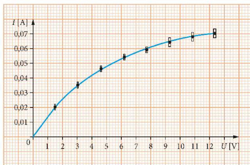
Rys. 13.43. Wykres zależności natężenia prądu od napięcia, sporządzony na podstawie danych z tabeli 13.6
