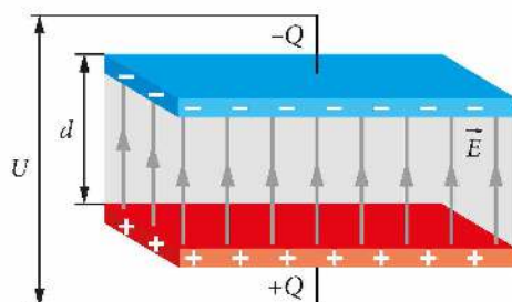
Rys. 12.44. Schemat kondensatora płaskiego
