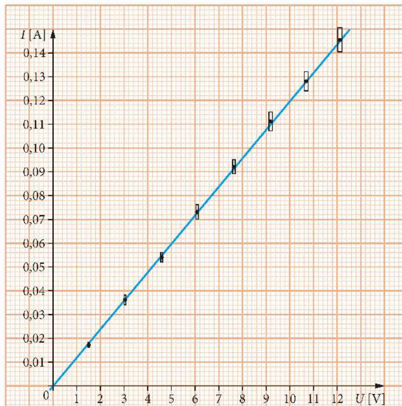
Rys. 13.30. Wykres zależności I(U) na podstawie danych z tabeli 13.4
