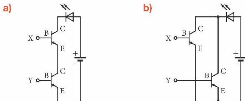
Rys. 15.48. Tranzystory połączone tak, aby dioda świeciła, gdy napięcie pojawi się: a) jednocześnie między wejściem X i ujemnym biegunem baterii oraz między wejściem Y i ujemnym biegunem baterii, b) między co najmniej jednym z wejść X lub Y oraz ujemnym biegunem baterii
