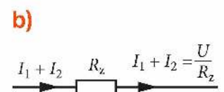
Rys. 13.38. Wyznaczanie oporu zastępczego oporników połączonych równoległe
