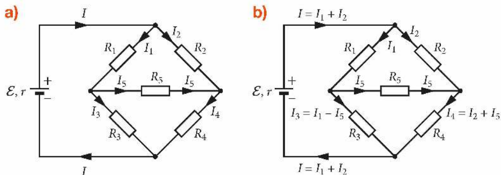
Rys. 13.59. Obwód z zaznaczonymi kierunkami przepływu prądu
