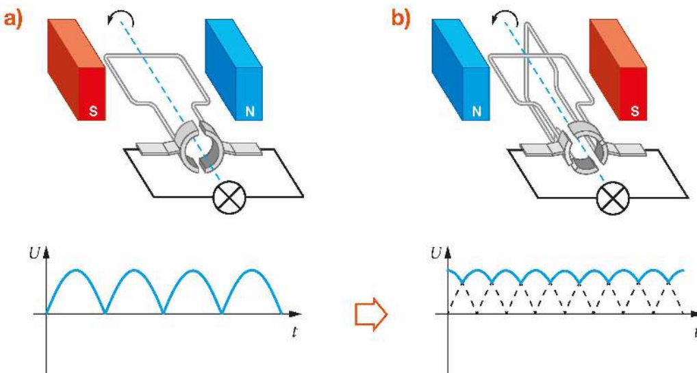
Rys. 15.29. Prądnica prądu stałego z komutatorem 2-segmentowym (a) i 4-segmentowym (b)
