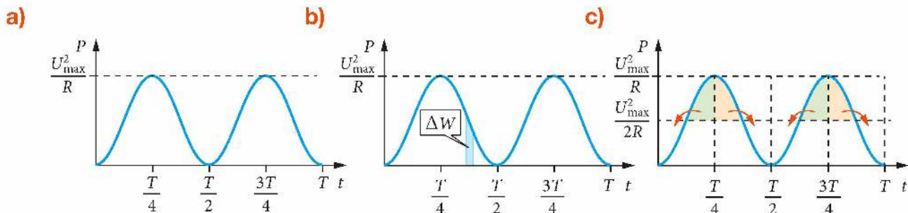
Rys. 15.13. Pracę prądu można wyznaczyć jako pole pod wykresem P(t) . a) Wykres P(t) , b) przybliżenie pracy przez schodki na wykresie, c) geometryczne wyznaczanie pola pod wykresem
