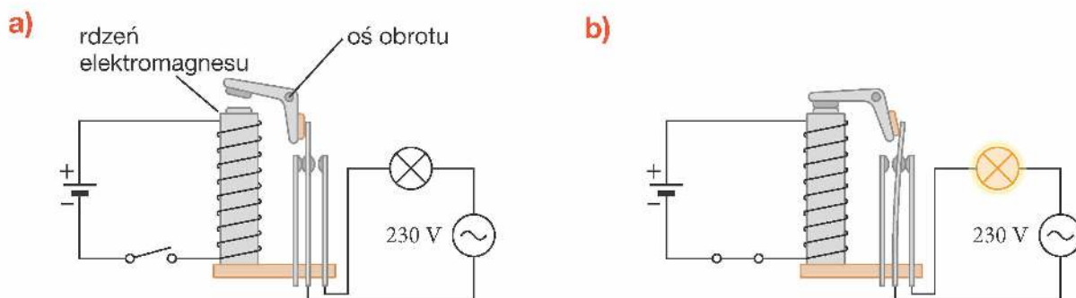
Rys. 15.47. Przekaznik może służyć do sterowania żarówką sieciową za pomocą obwodu niskiego napięcia: a) prąd z baterii nie płynie, obwód napięcia 230 V jest otwarty, żarówka nie świeci, b) prąd z baterii płynie, elektromagnes powoduje zamknięcie obwodu napięcia 230 V, żarówka świeci
