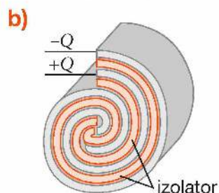
Rys. 12.39. Budowa kondensatora a) płaskiego, b) zwijanego
