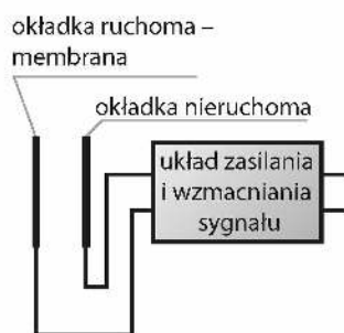
Rys. 12.47. Schemat mikrofonu pojemnościowego
