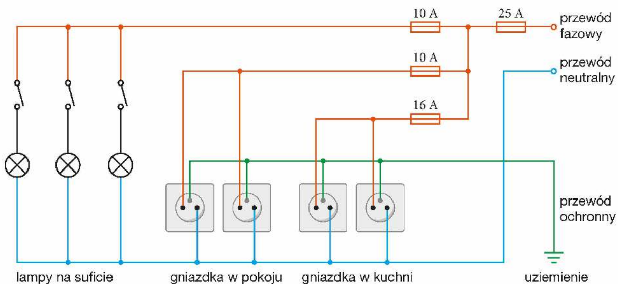
Rys. 15.17. Przykład użycia bezpieczników w sieci domowej
