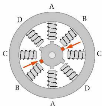
Rys. 15.27. Schemat silnika krokowego
