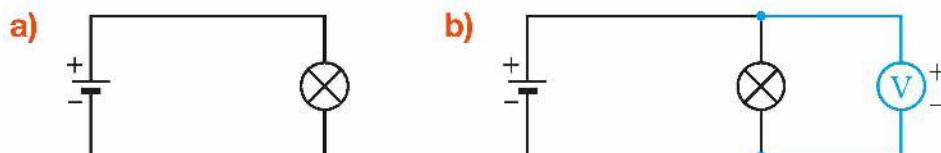
Rys. 13.14. Pomiar napięcia na żarówce: a) wyjściowy obwód, b) obwód z podłączonym woltomierzem
