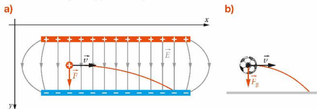
Rys. 12.38. a) ruch ciała naładowanego dodatnio: w jednorodnym polu elektrycznym, z prędkością początkową \vec{v} prostopadłą do kierunku wektora natężenia pola, b) rzut poziomy
