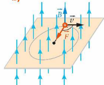
Rys. 14.22. Siła Lorentza działająca na ładunek poruszający się: a) wzdłuż linii pola, b) prostopadłe do linii pola
