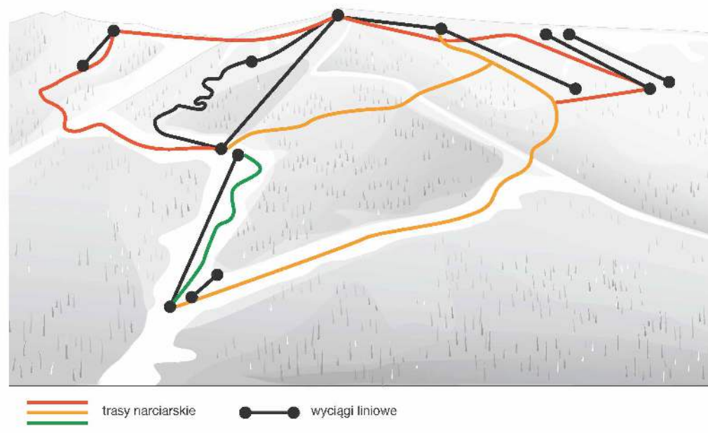
Rys. 13.57. Zmiany energii ładunku w obwodzie elektrycznym można porównać do zmian energii potencjalnej narciarza przemieszczającego się w obrębie stacji narciarskiej
