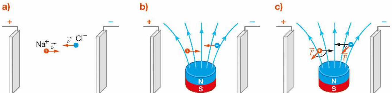
Rys. 14.18. Schemat działania siły Lorentza \vec{F} na jony w polu magnetycznym
