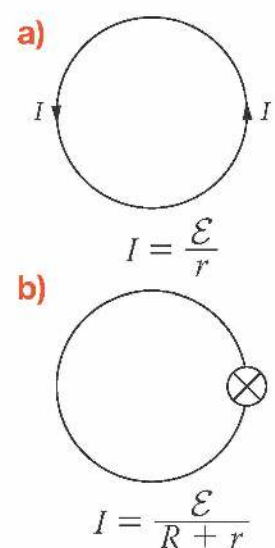
Rys. 15.10. Natężenie prądu indukcyjnego płynącego w: a) pętli, b) pętli z odbiornikiem energii (żarówką)
