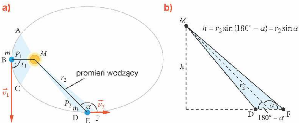
Rys. 11.36. Pola zakreślonych obszarów są równe. Dwa fragmenty elipsy między punktami A i C oraz D i F planeta pokonuje w jednakowych przedziałach czasu. Prędkość planety między punktami A i C jest większa niż między punktami D i F ( v_1 > v_2 )
