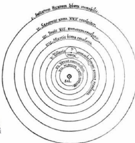
Rys. 11.39. Rycina z dzieła Kopernika O obrotach sfer niebieskich . Przy orbitach kolejnych planet podano ich okres obiegu (tłumaczenie znajduje się obok ilustracji)
