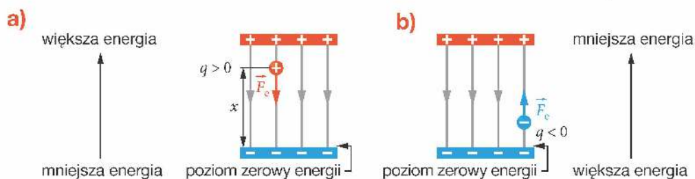
Rys. 12.26. Energia ładunku dodatniego rośnie (a), a ujemnego maleje (b) podczas odsuwania go od ujemnie naładowanej płytki
