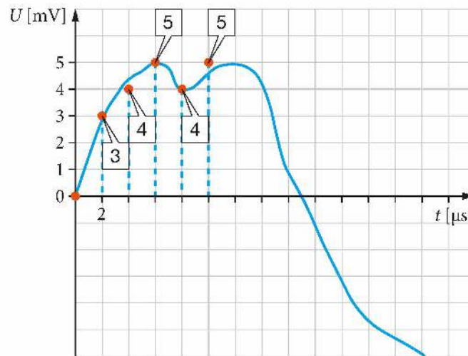
Rys. 15.46. Dźwięk można zapisać za pomocą serii liczb oznaczających napięcie wytwarzane przez mikrofon w równych odstępach czasu: 0, 3, 4, 5, 4, 5, ...
