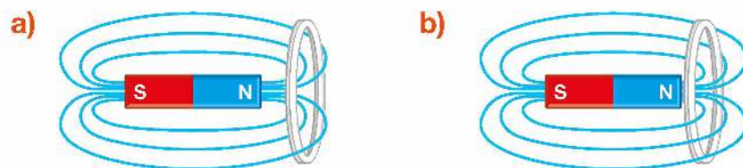
Rys. 15.3. Liczba linii pola przechodzących przez pętlę zależy od położenia magnesu względem pętli
