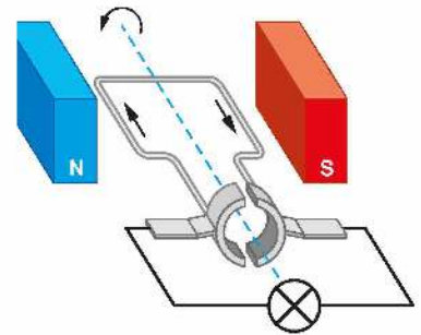
Rys. 15.28. Silnik może działać jak prądnica
