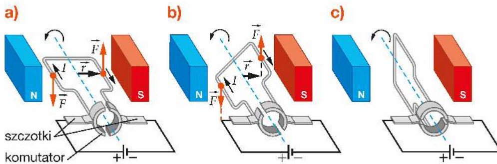
Rys. 15.24. Pojedyncza ramka to najprostszy model silnika elektrycznego
