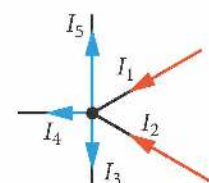
Rys. 13.22. Pierwsze prawo Kirchhoffa dla pojedynczego węzła
