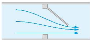
Rys. 15.35. Zawór, który przepuszcza wodę w jedną stronę (a), natomiast zamyka jej przepływ w przeciwnym kierunku (b). Jego odpowiednikiem dla prądu elektrycznego jest dioda
