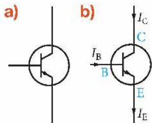
Rys. 15.43. Symbol tranzystora bipolarnego npn (a) z zaznaczonymi końcówkami i kierunkiem przepływu prądu (b)
