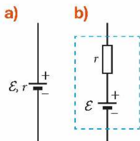
Rys. 13.51. Rzeczywiste źródło napięcia (a) i jego schemat zastępczy (b)
