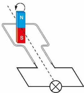
Rys. 15.30. Prądnica prądu przemiennego
