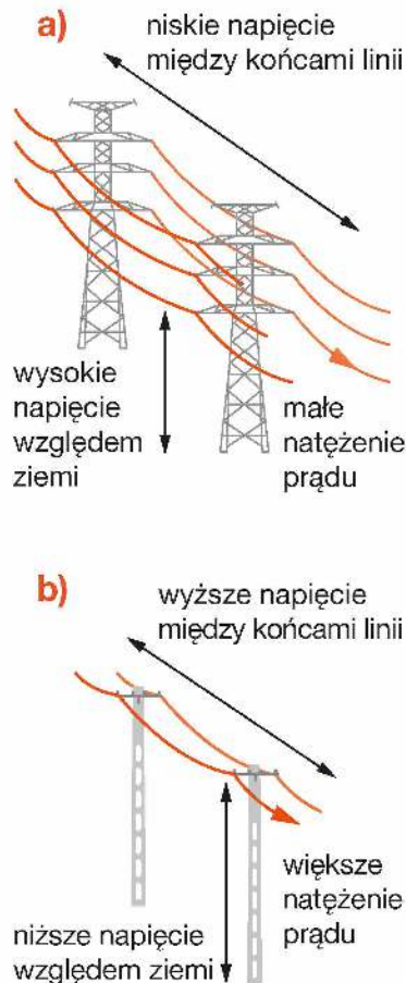
Rys. 15.32. Przesyłanie energii elektrycznej
