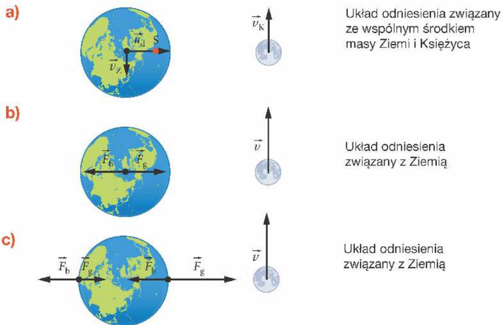
Rys. 11.48. Powstawanie sił pływowych
