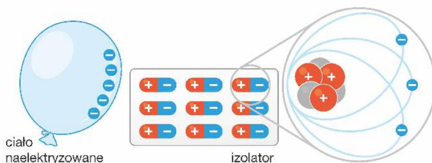
Rys. 12.9. Przesunięcie powłok elektronowych względem jądra atomu powoduje polaryzację cząsteczki. Spolaryzowane cząsteczki są przyciągane przez naelektryzowane ciało
