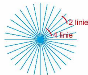
Rys. 12.15. Na płaszczyźnie dwukrotne zwiększenie odległości powoduje dwukrotne zmniejszenie zagęszczenia linii, ale w rzeczywistości – czterokrotne
