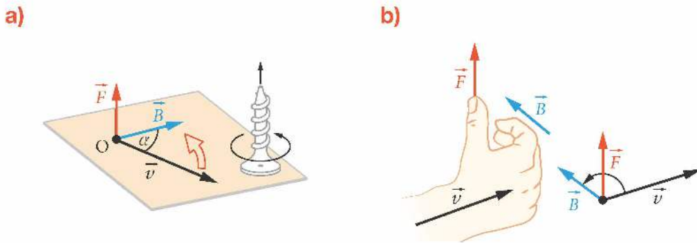
Rys. 14.20. Wyznaczanie zwrotu siły Lorentza za pomocą reguły śruby prawoskrętnej (a) i reguły prawej ręki (b)
