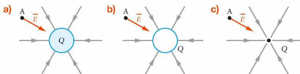
Rys. 12.22. Ciało sferycznie symetryczne o równomiernie rozmieszczonym ładunku – zarówno kula (a), jak i sfera (b) – wytwarza na zewnątrz takie pole jak ładunek punktowy (c) umieszczony w jego środku. Natężenie pola w punkcie A w każdym przypadku będzie takie samo
