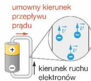
Rys. 13.6. Porównanie umownego kierunku prądu z rzeczywistym kierunkiem uporządkowanego ruchu elektronów
