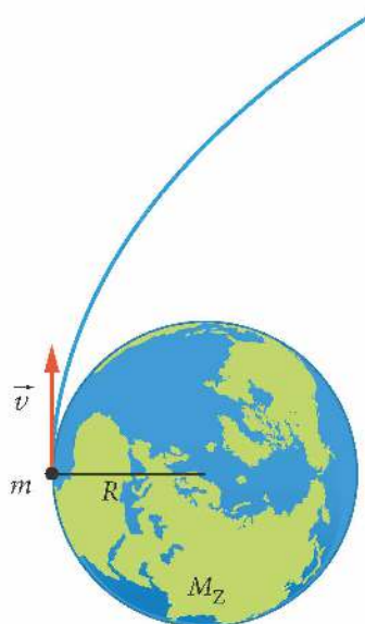
Rys. 11.45. Całkowita energia ciała wyrzuconego z Ziemi z drugą prędkością kosmiczną jest podczas ruchu stała i równa zero
