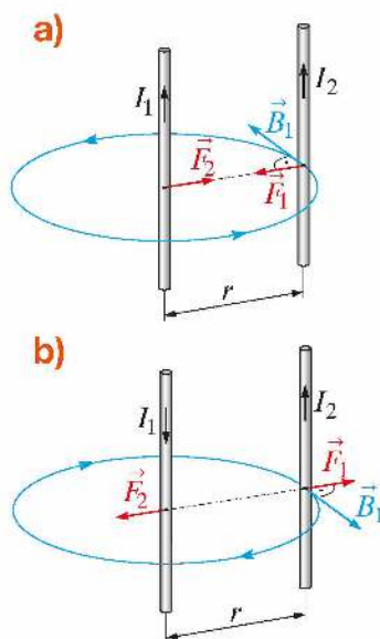
Rys. 14.31. Siły działające między przewodnikami, w których prąd płynie: a) w tę samą stronę – przyciąganie, b) w przeciwnie strony – odpychanie
