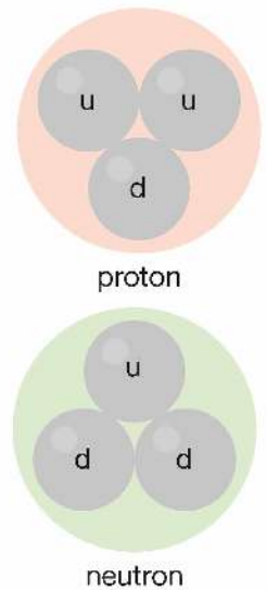
Rys. 12.2. Protony i neutrony są zbudowane z kwarków górnych ( u ) i dolnych ( d )
