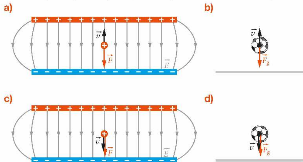
Rys. 12.37. Porównanie ruchu odbywającego się równoległe do linii jednorodnego pola elektrycznego (a, c) i rzutu pionowego (b, d)
