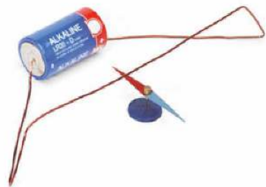
Rys. 14.8. Odchylenie igły magnetycznej pod wpływem przepływu prądu świadczy o tym, że ruch ładunków jest źródłem pola magnetycznego
