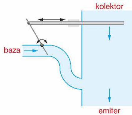
Rys. 15.42. Wodny model tranzystora: woda płynąca cienką rurką z bazy popycha kłapkę, która porusza zasuwkę regulującą przepływ wody z szerokiego kolektora
