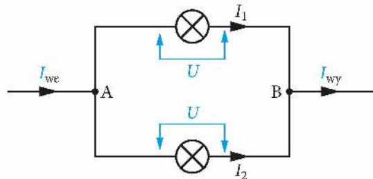
Rys. 13.20. Napięcia na dwóch żarówkach połączonych równoległe są takie same
