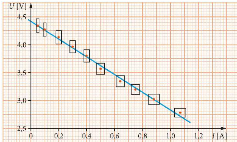
Rys. 13.54. Wykres zależności U(I) na podstawie danych z tabeli 13.8
