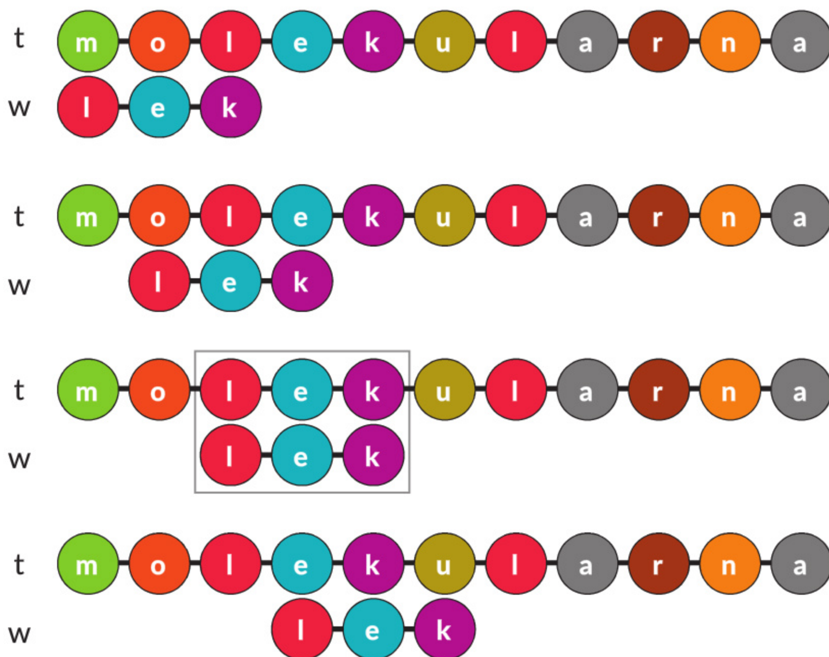
Rys. 5. Cztery z dziewięciu etapów procesu wyszukiwania wzorca w słowie molekularna
