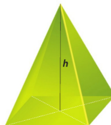
Ostrosłup
