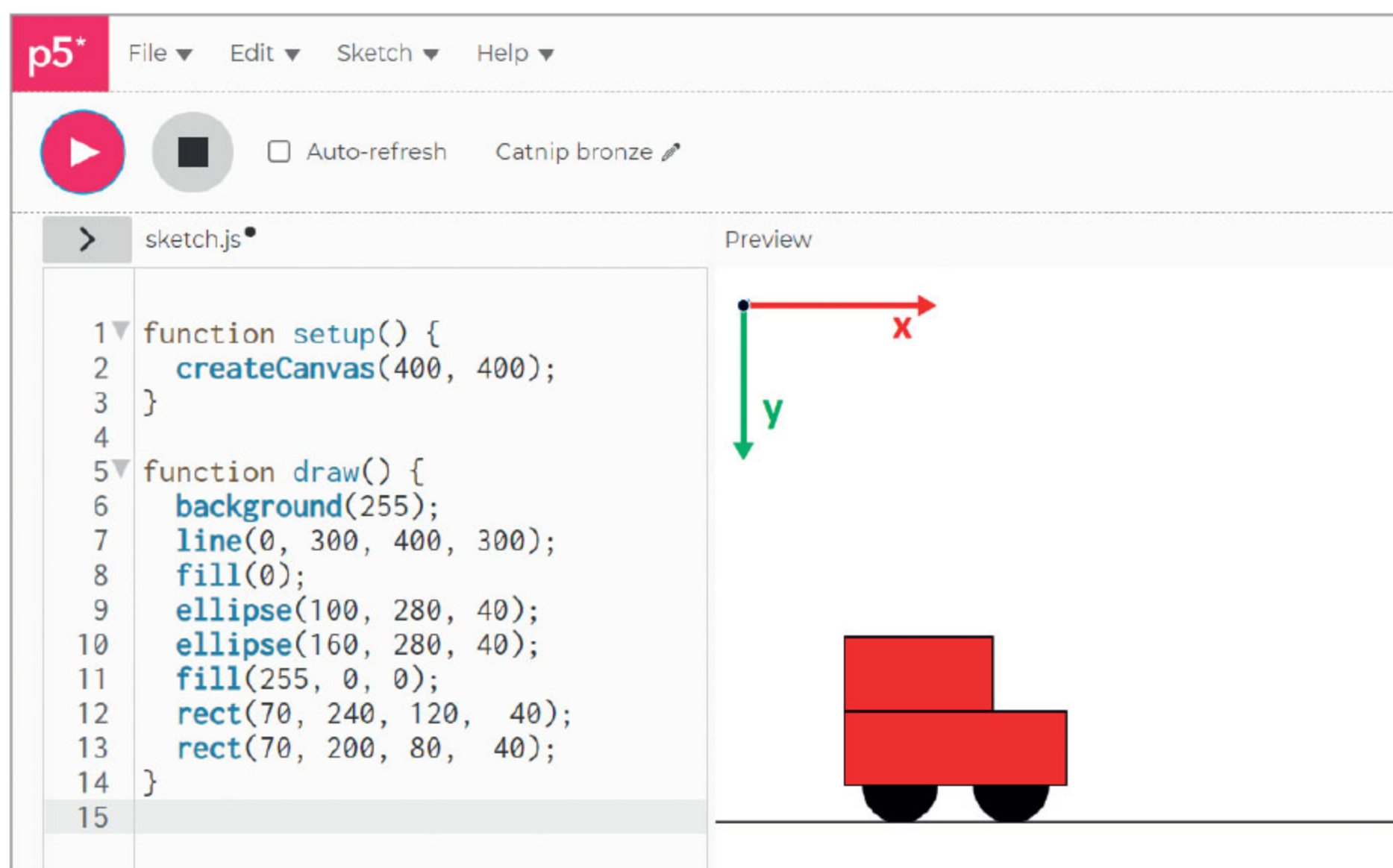
Rys. 8. Przykładowy kod odpowiadający za narysowanie samochodu. Początek układu współrzędnych znajduje się w lewym górnym rogu, przy czym x rośnie w prawo, a y – w dół
