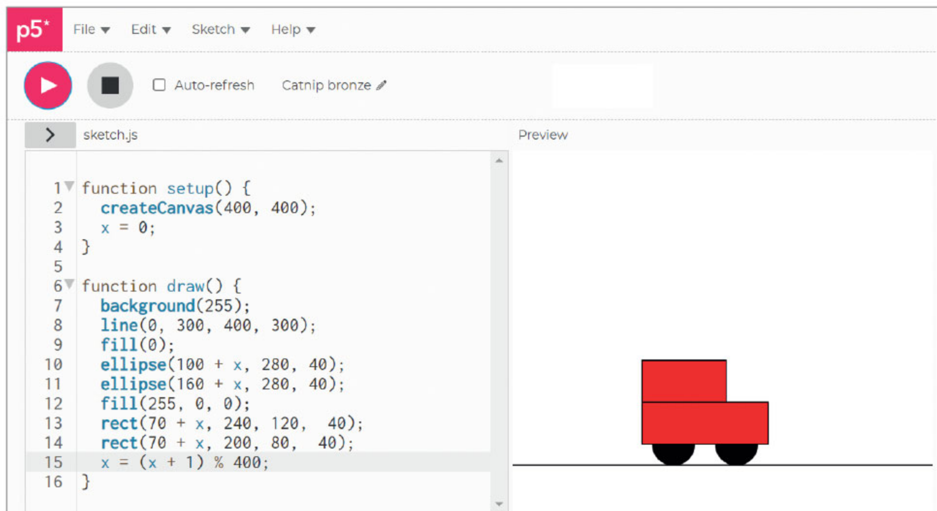
Rys. 10. Zmodyfikowany kod odpowiadający za narysowanie i poruszanie się samochodu
