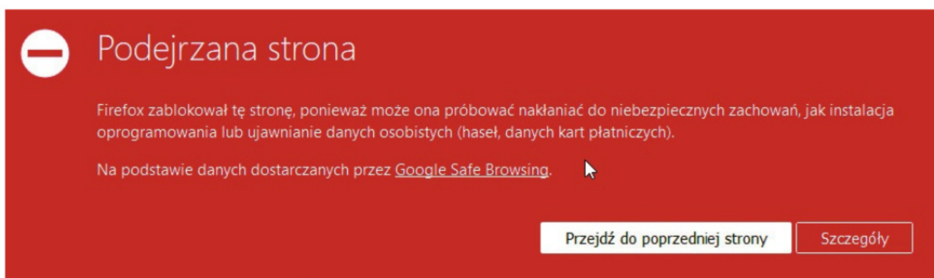
Rys. 1. Przykład phishingu
