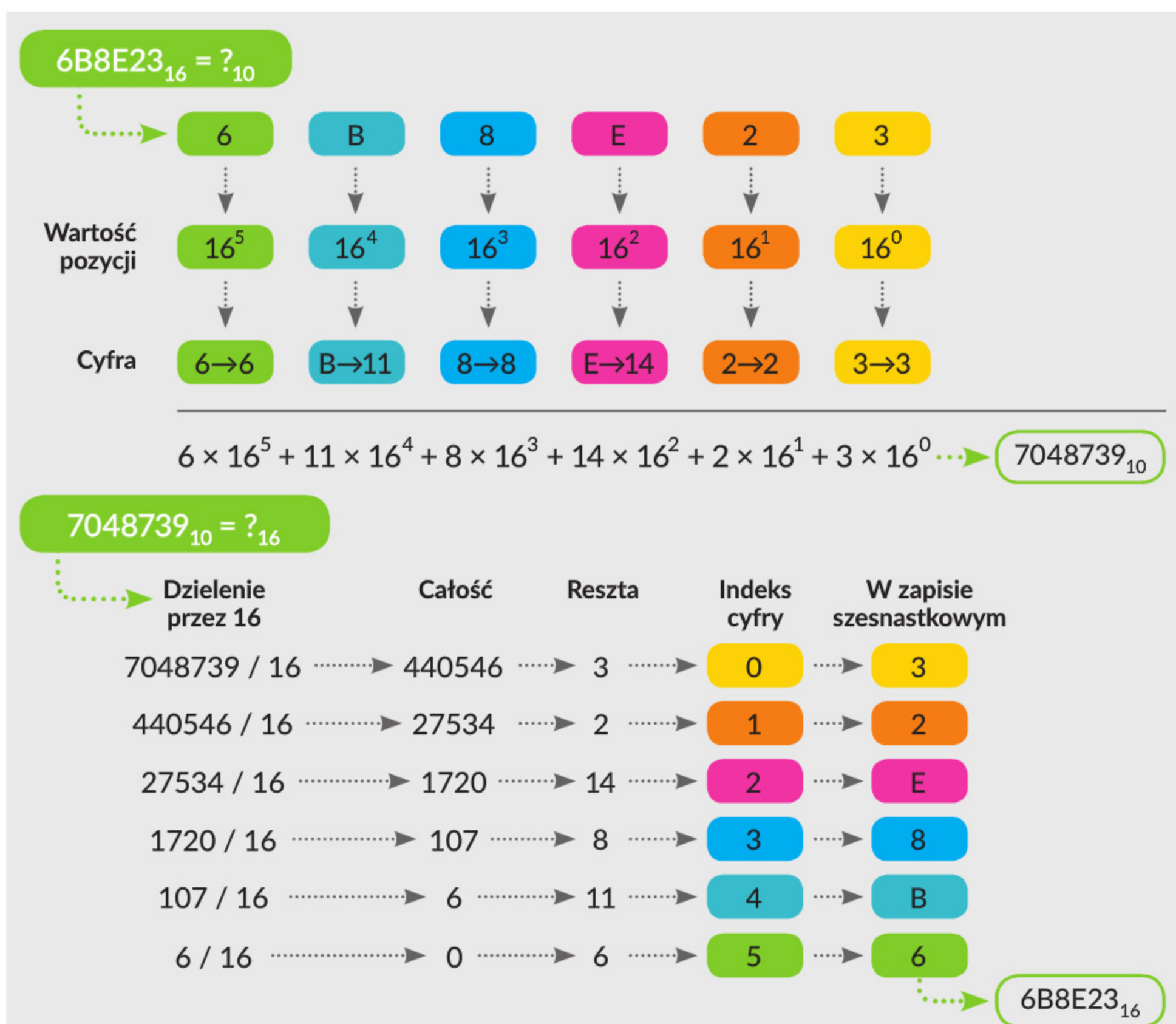
Rys. 7. Zamiana liczby szesnastkowej na dziesiętkową i odwrotnie
