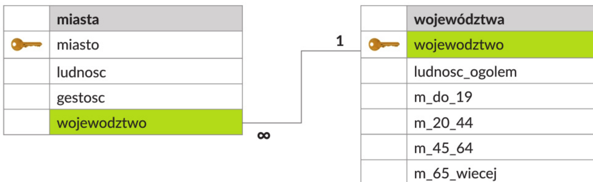
Rys. 4. Relacja 1: ∞ – jednemu rekordowi w tabeli województwa odpowiada co najmniej jeden rekord w tabeli miasta
