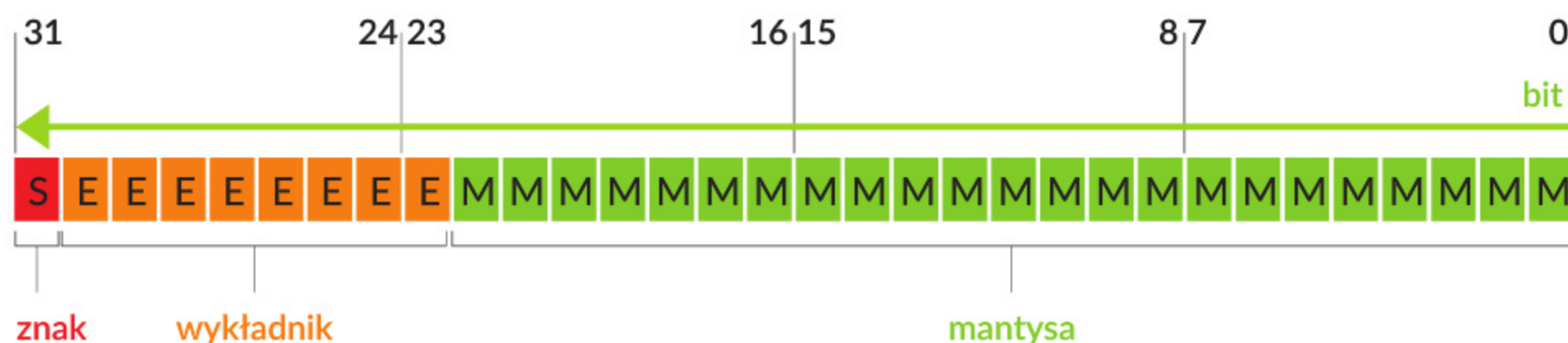
Rys. 6. Reprezentacja liczb zmiennoprzecinkowych w komputerze
