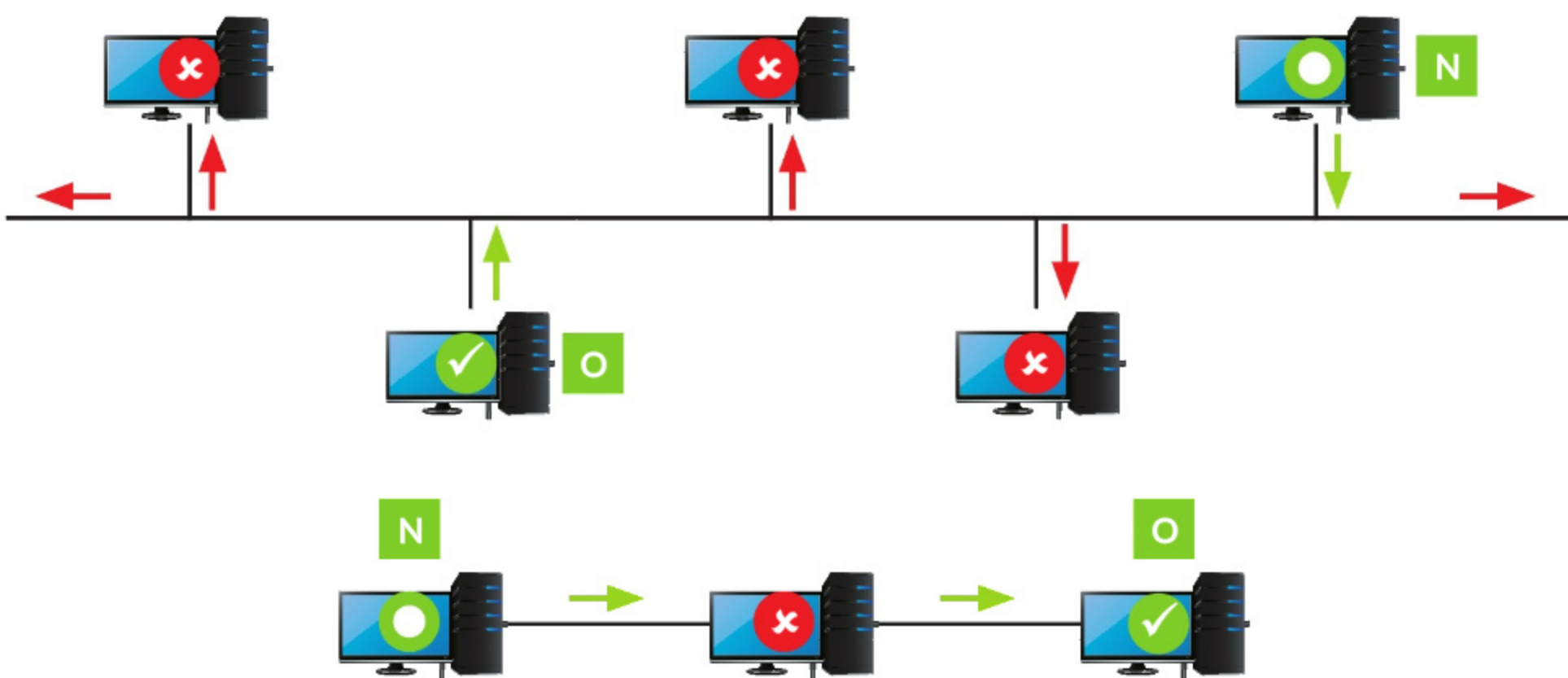
Rys. 2. Model magistrali (na górze) i jego odmiana – model liniowy
