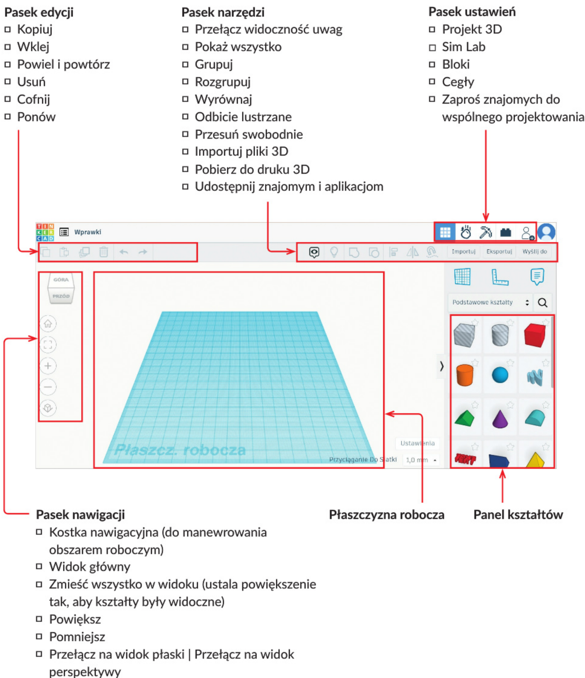
Rys. 2. Okno programu Tinkercad
