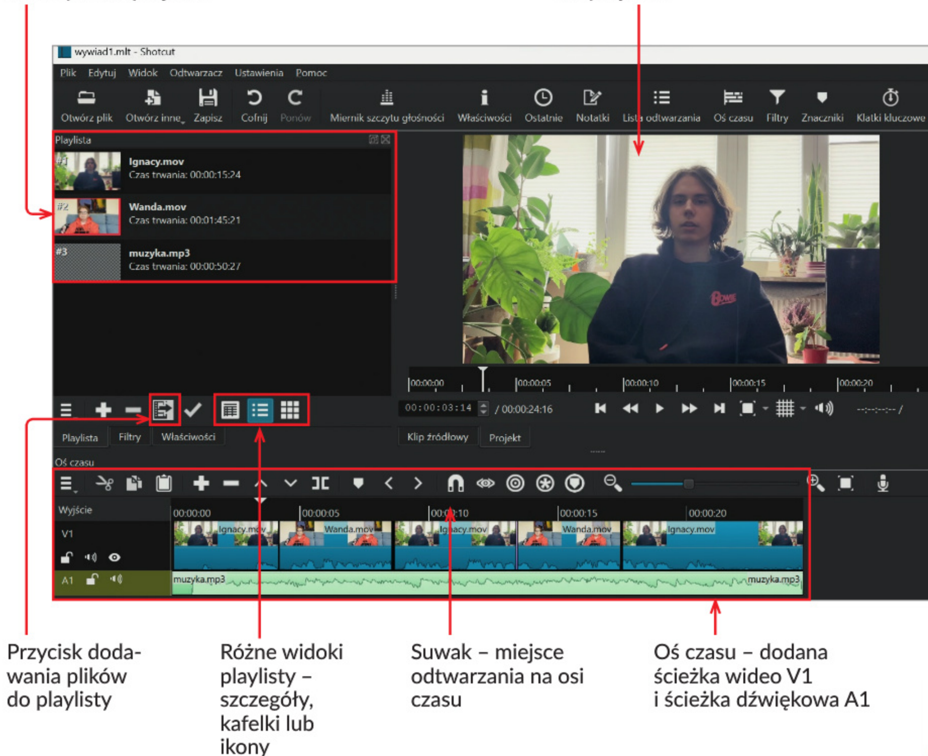
Rys. 1. Okno programu Shotcut
