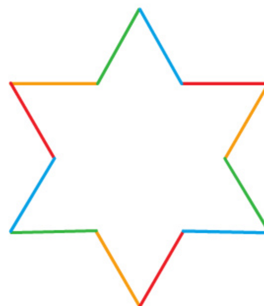
płatek Kocha stopnia 1.
