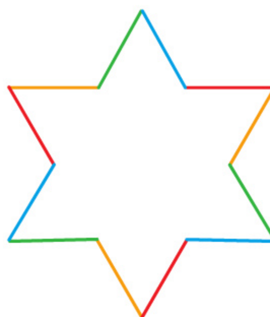
płatek Kocha stopnia 1.
