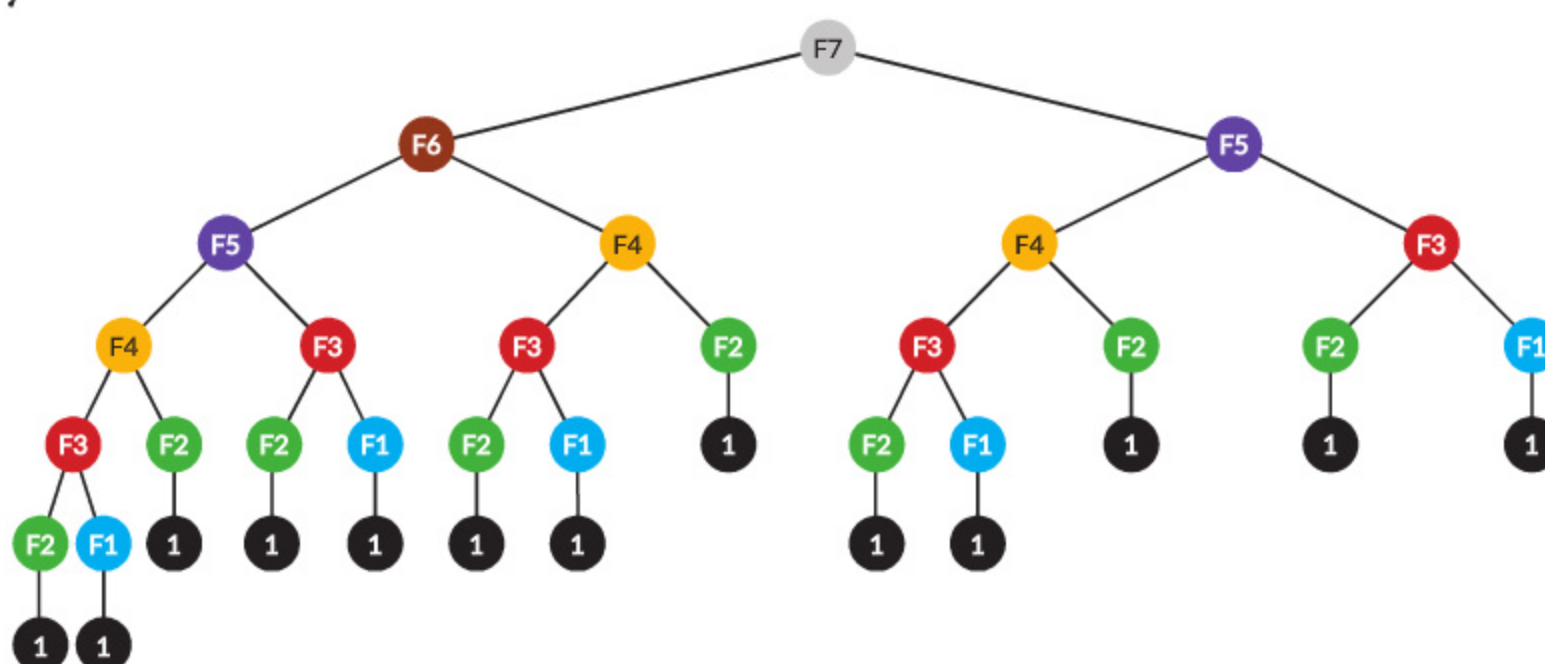
Rys. 2. Obliczanie siódmej liczby Fibonacciego – dla n = 7 wartość funkcji F5 obliczana jest dwa razy, F4 trzy razy, F3 pięć razy, ...
