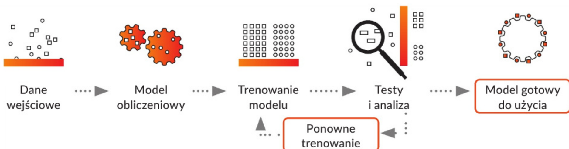
Rys. 2. Proces uczenia maszynowego
