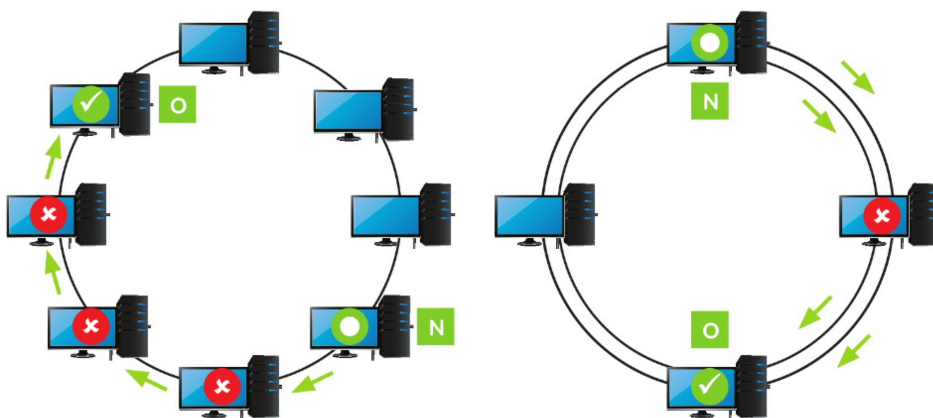
Rys. 3. Modele pierścienia (z lewej) i jego odmiana – model podwójnego pierścienia
