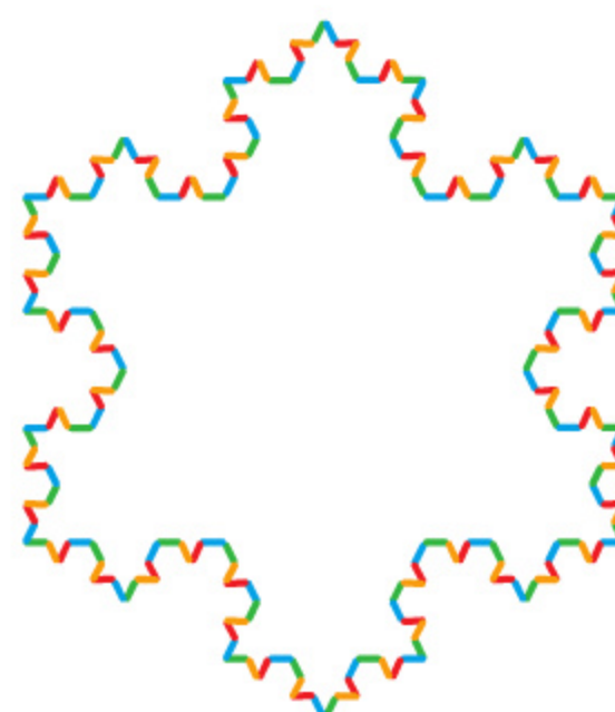
płatek Kocha stopnia 3.
