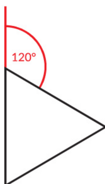
Rys. 2. Trójkąt z zaznaczonym kątem obrotu
