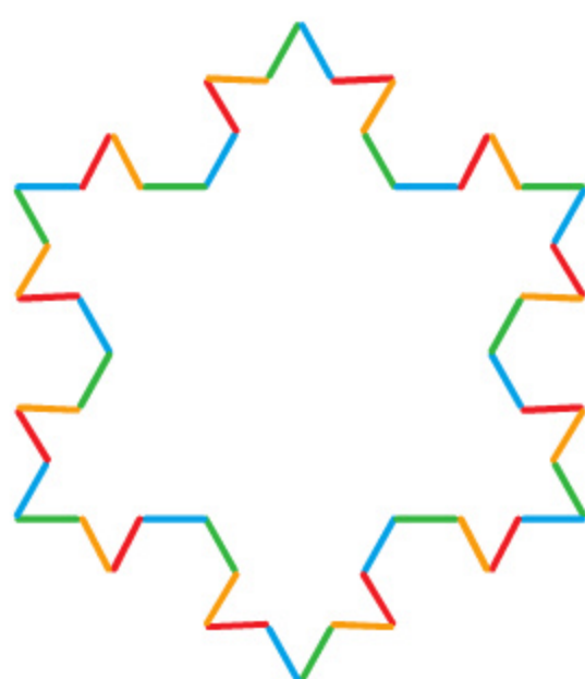
płatek Kocha stopnia 2.
