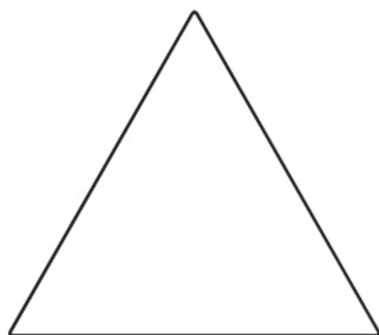
płatek Kocha stopnia 0.
