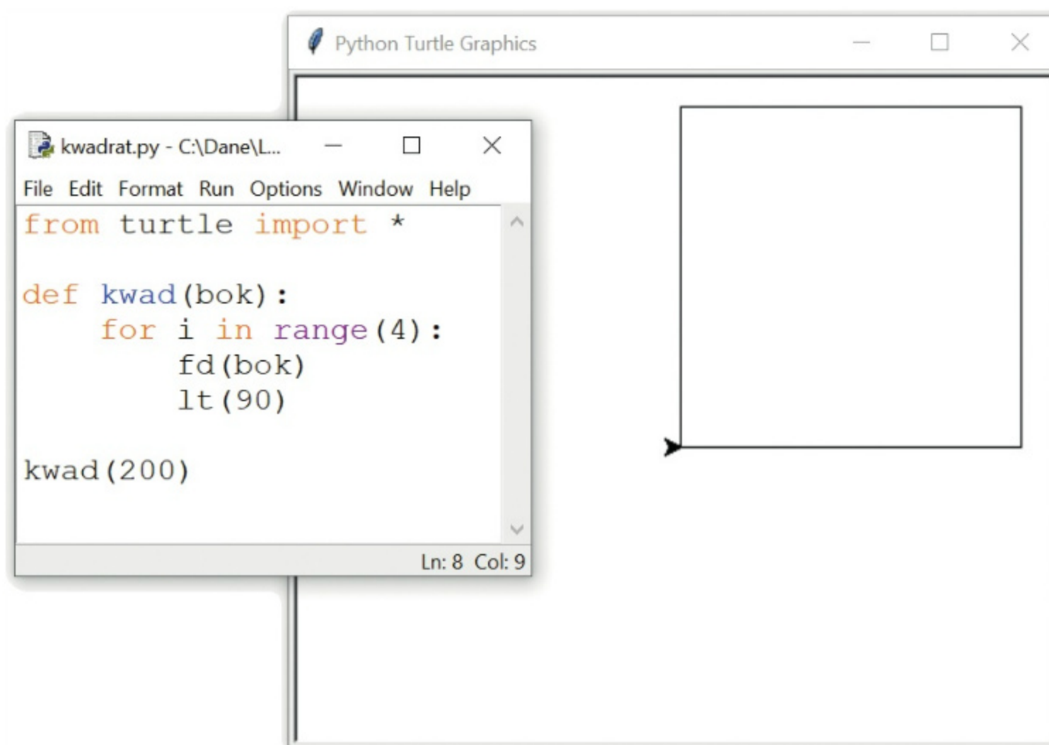
Rys. 2. Rysowanie kwadratu z wykorzystaniem modułu turtle
