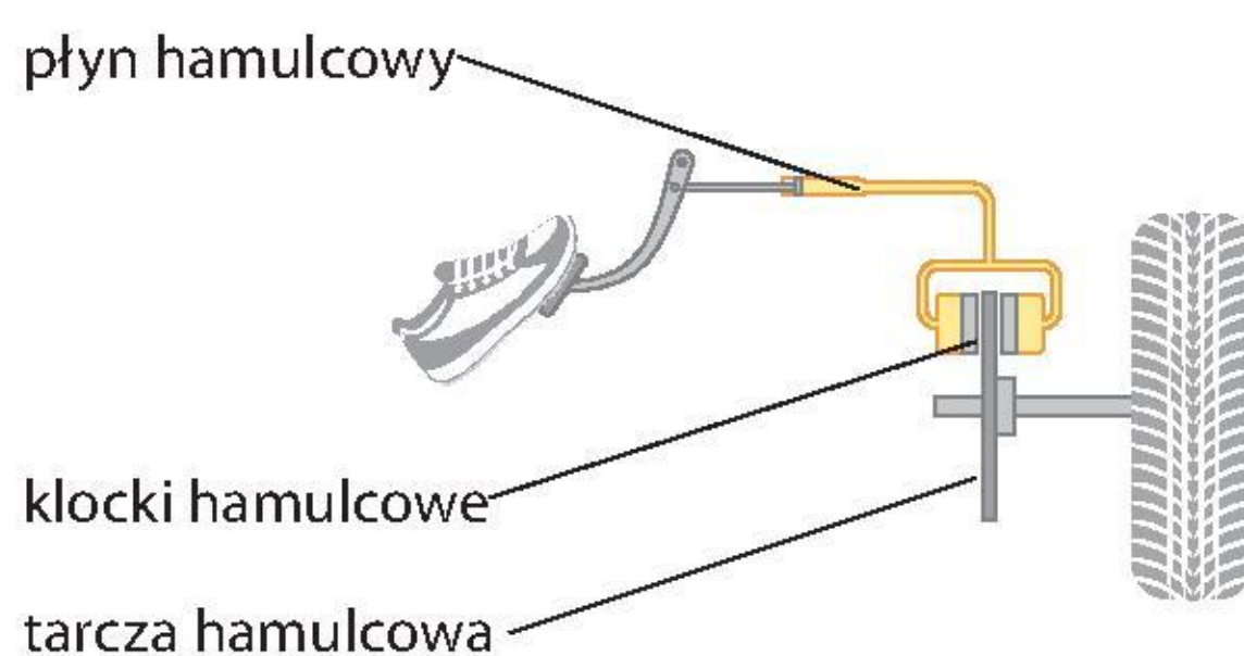
Schemat zasady działania hamulca hydraulicznego.
