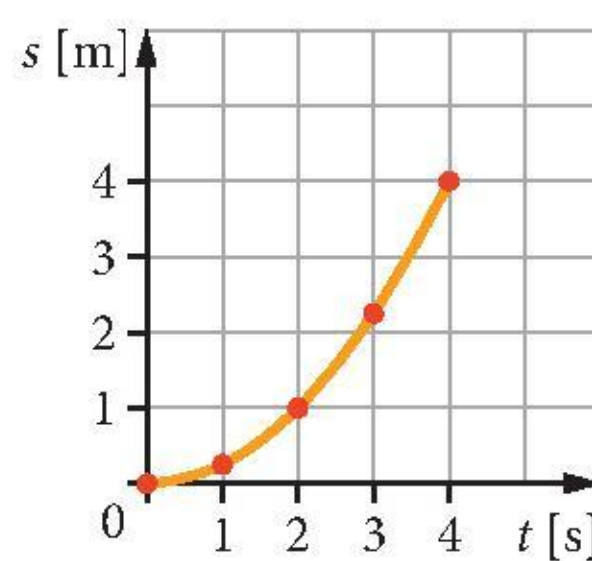
Wykres zależności drogi od czasu dla pociągu poruszającego się z przyspieszeniem 0,5 \frac{\text{m}}{\text{s}^2} .
