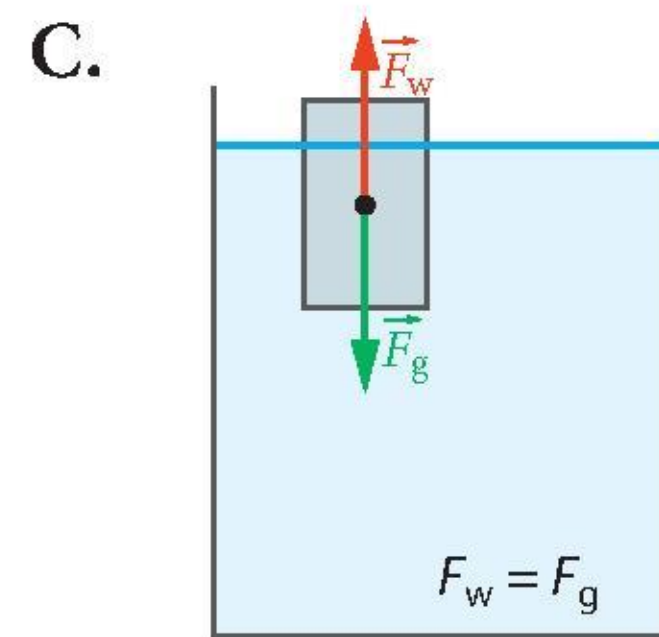
Ciało częściowo zanurzone.
