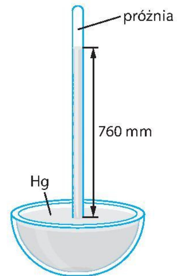
Schemat doświadczenia Torricellego.
