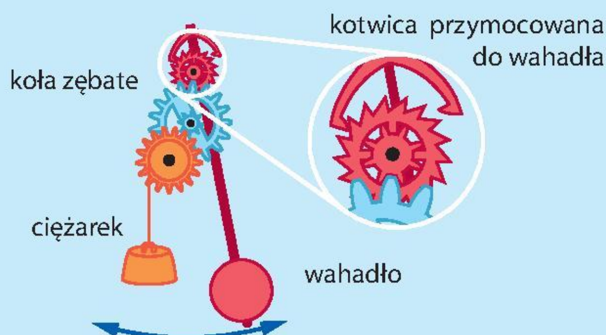
Uproszczony mechanizm działania zegara wahadłowego.
