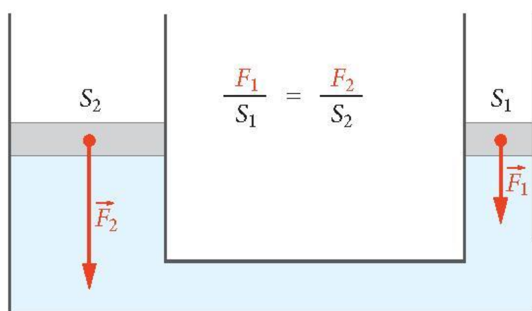
Schemat prasy hydraulicznej.
