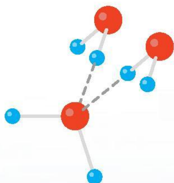
Wiązania wodorowe (zaznaczone linią przerywaną)
