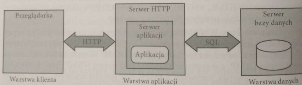
Rysunek 2.2. Programowalne warstwy aplikacji internetowej
