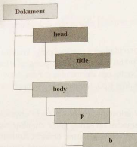
Rysunek 3.5. Hierarchia obiektów przykładowej strony internetowej
