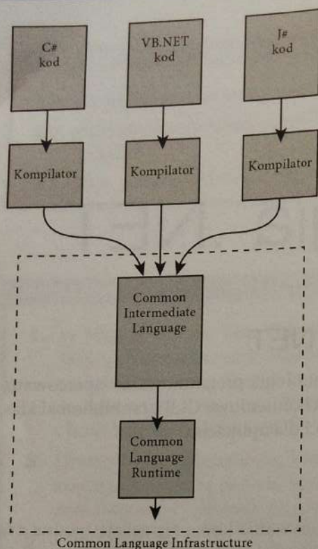
Rysunek 8.1. Sposób wykonania kodu platformy .NET
