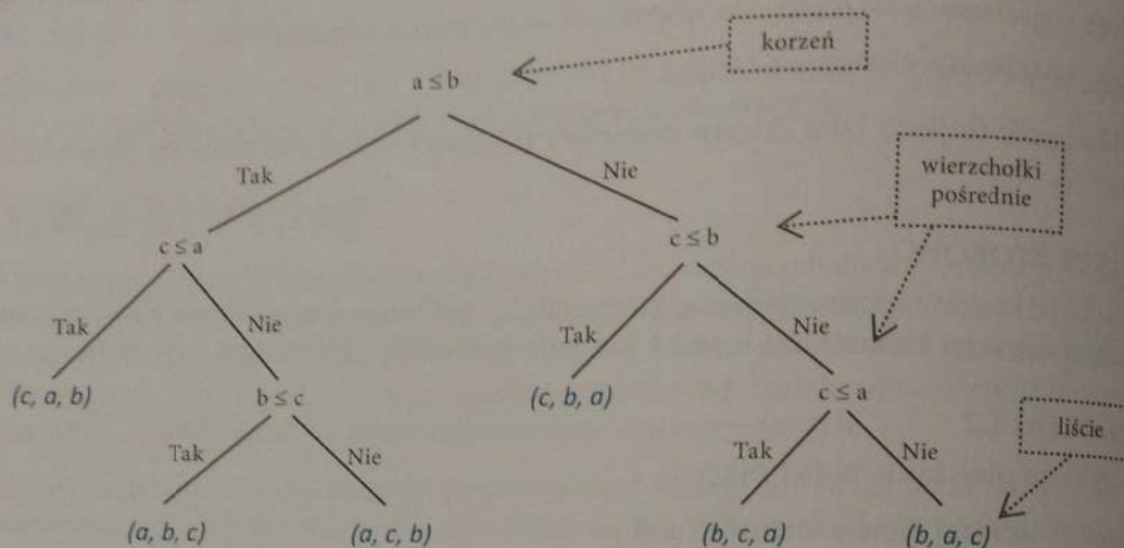
Rysunek 1.1. Przykładowe drzewo algorytmu
