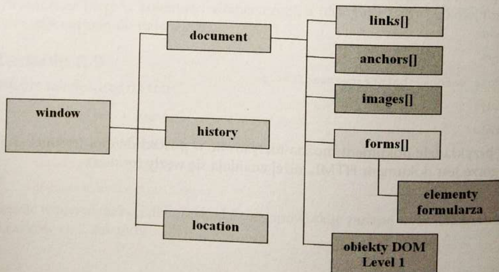
Rysunek 3.6. Hierarchia obiektów DOM
