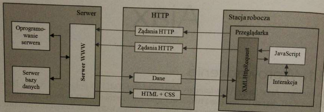
Rysunek 5.1. Struktura komunikacji między serwerem a użytkownikiem w technologii Ajax
