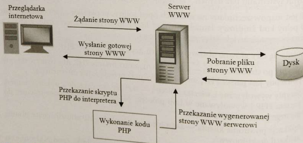
Rysunek 7.1. Proces przetwarzania kodu PHP
