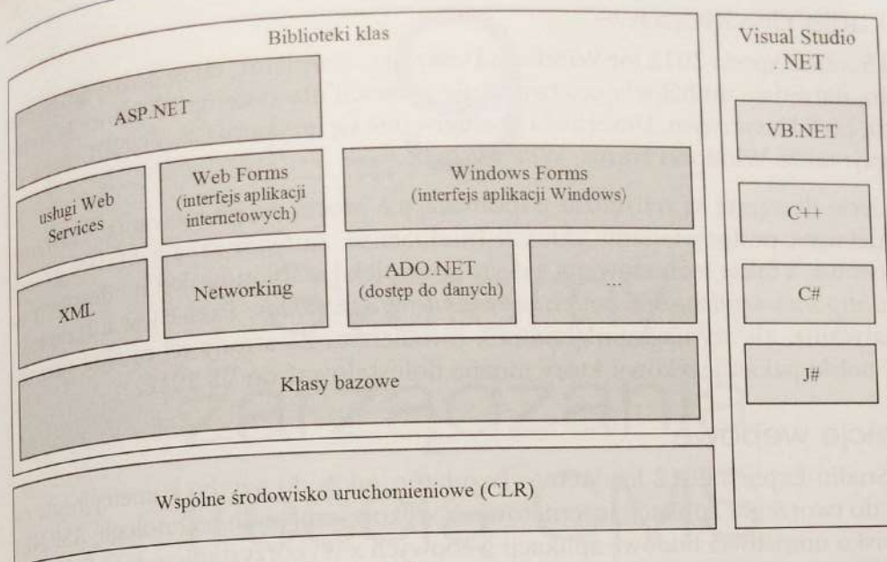
Rysunek 8.2. Struktura platformy .NET
