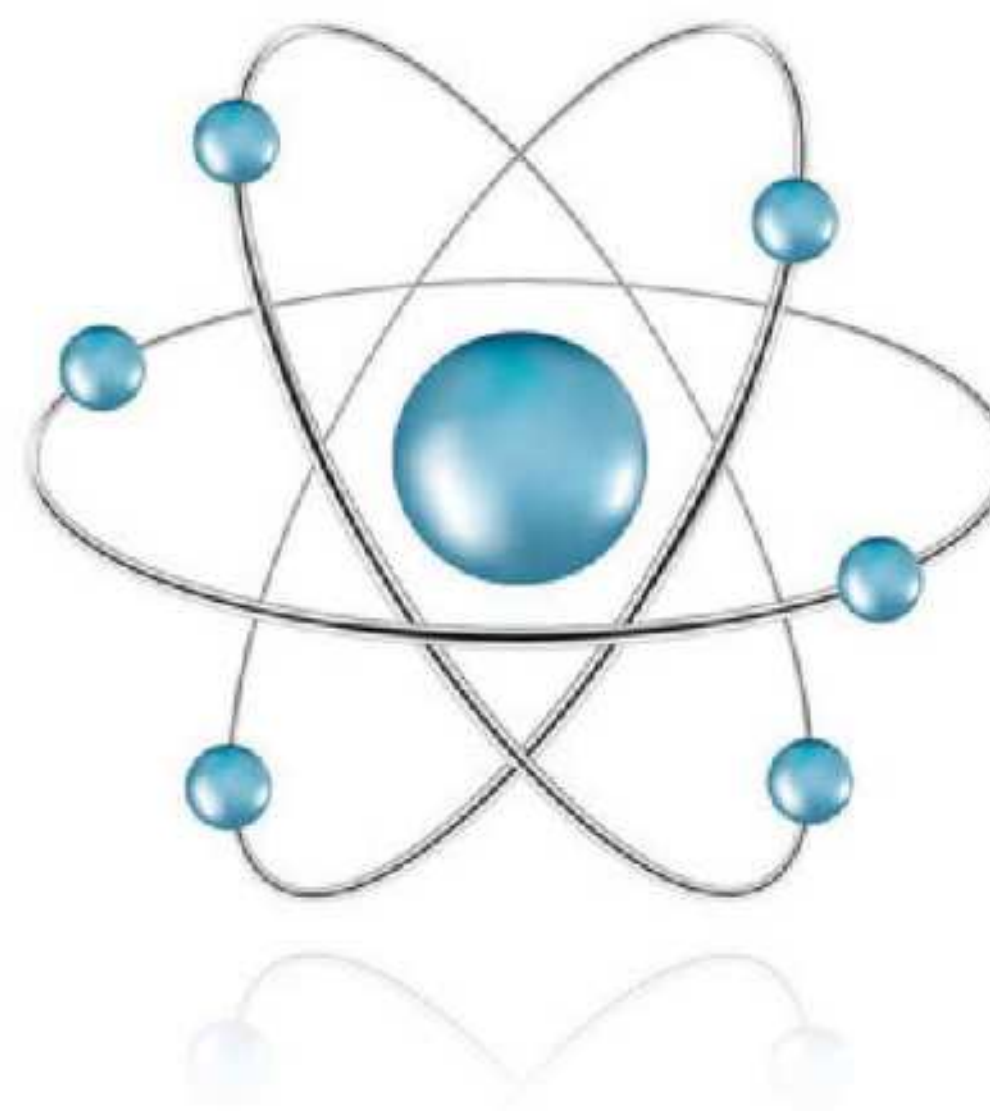
XX-wieczny model atomu Nielsa Bohra [czyt.: nilsa bora]
