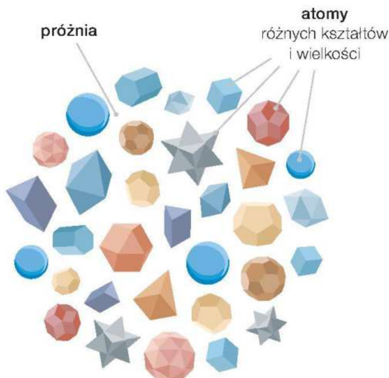
Różnorodność atomów według Demokryta
