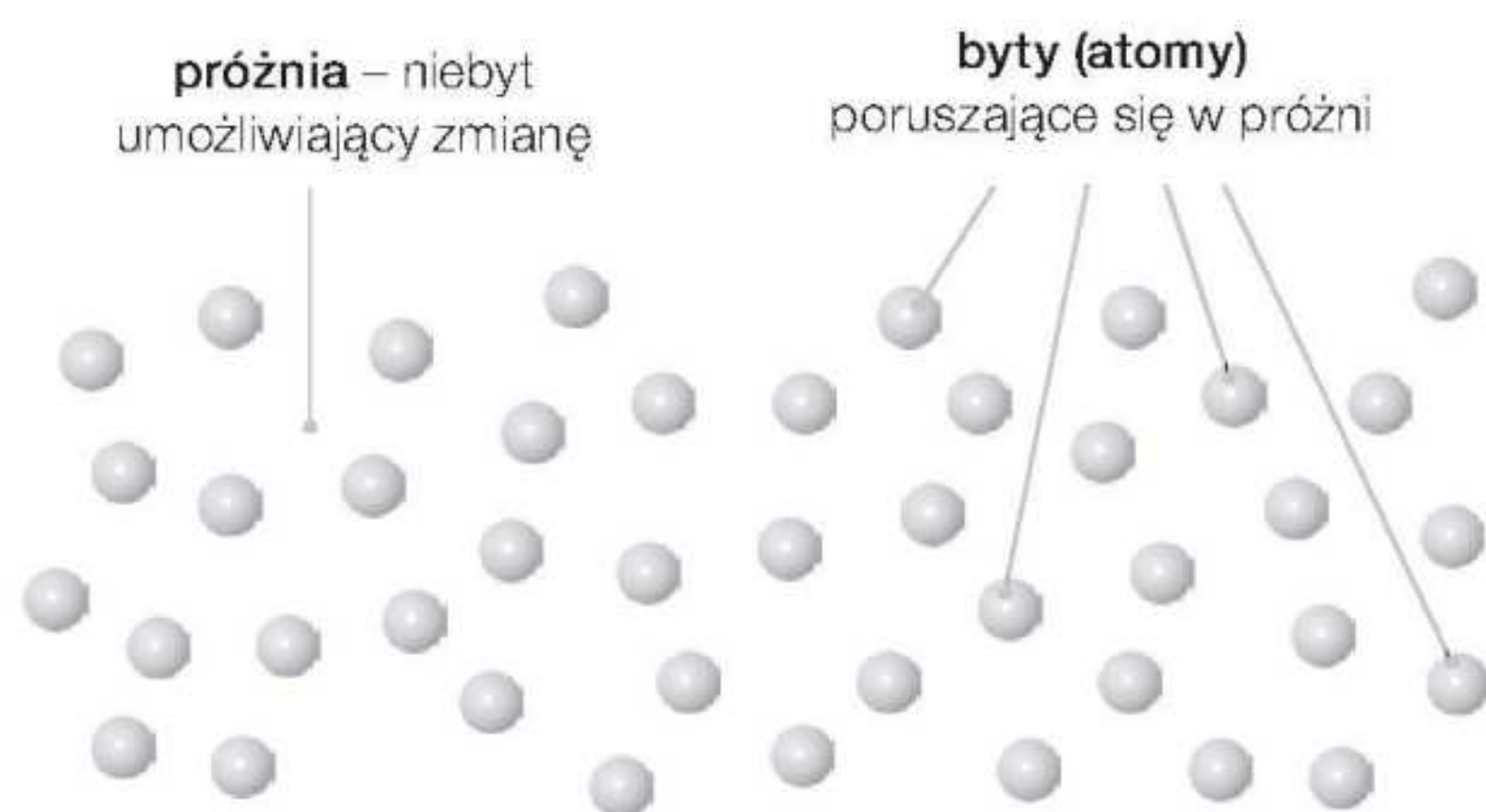
Budowa świata według Leucypa
