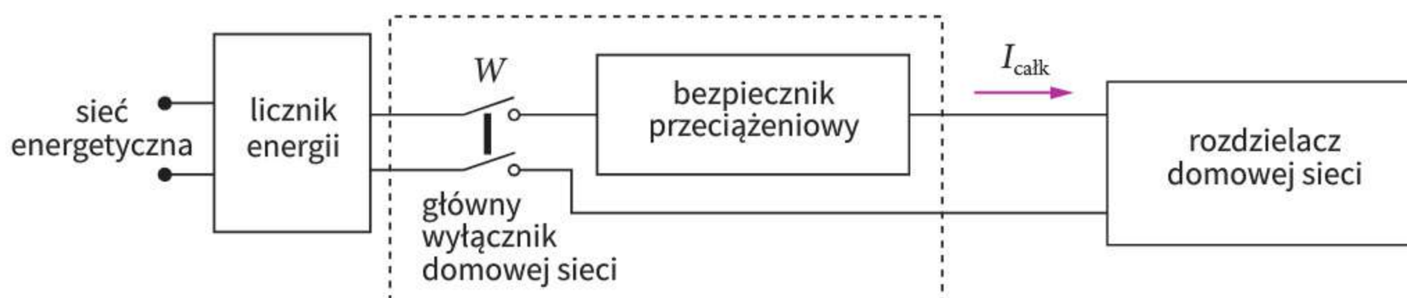
Ryc. 13.1. Elementy przyłączeniowe domowej sieci elektrycznej
