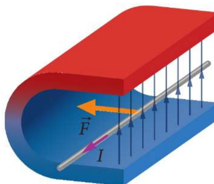
Ryc. 16.1. Prostoliniowy przewód z prądem w polu magnetycznym, ustawiony prostopadle do linii pola. Zwrot siły zależy od zwrotu linii pola i kierunku prądu
