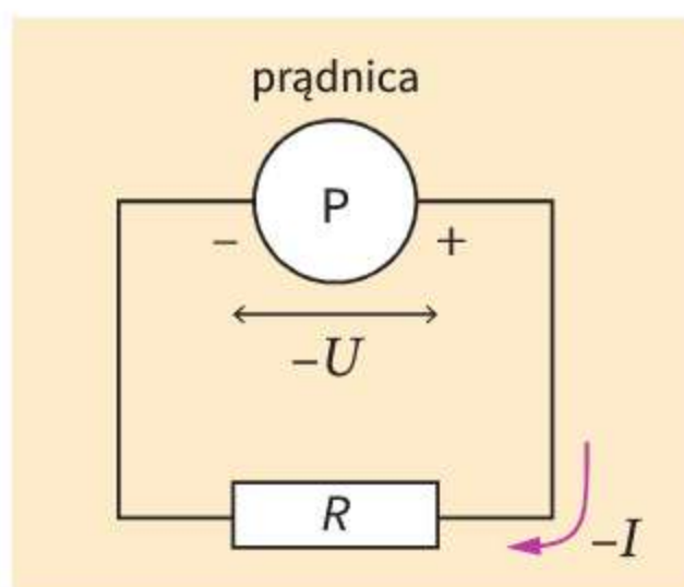
Ryc. 22.1. Schemat obwodu z prądnicą prądu przemiennego oraz wykresy zależności napięcia na zaciskach prądnicy i natężenia prądu w obwodzie od czasu
