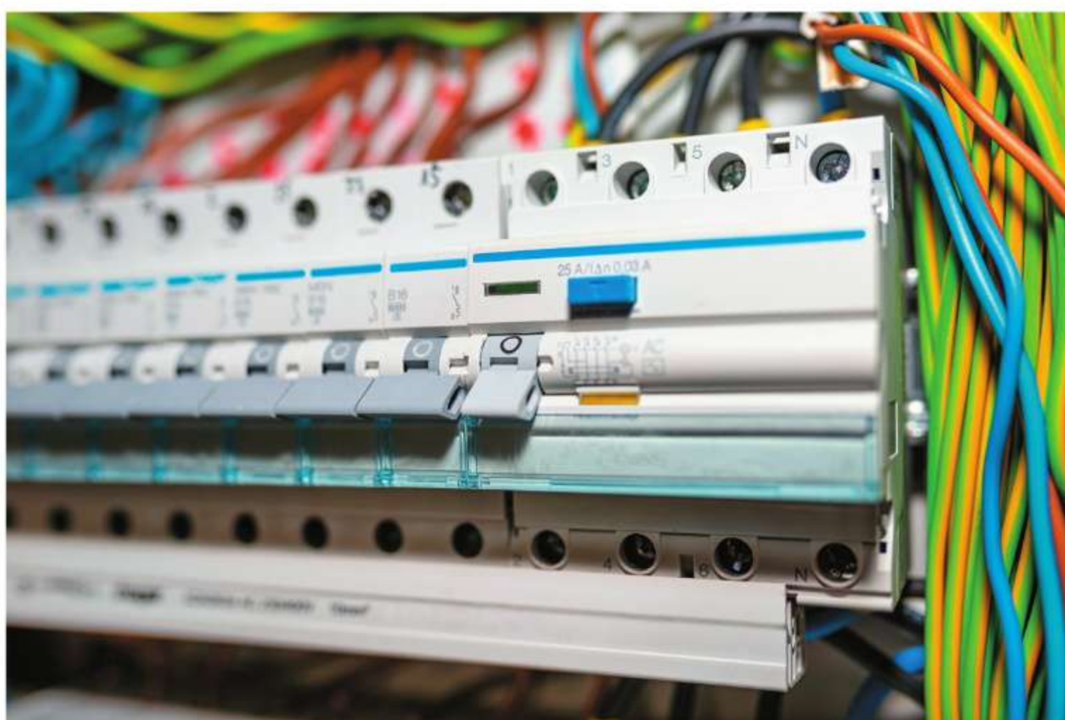
Ryc. 13.5. Bezpieczniki różnicowoprądowe w domowej instalacji elektrycznej
