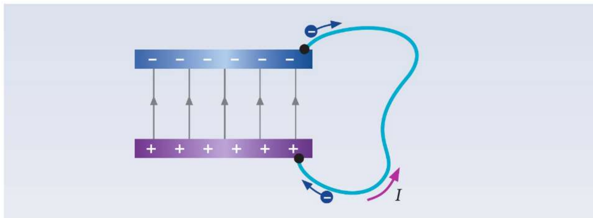
Ryc. 9.1. Prąd płynący w przewodzie rozładowuje kondensator
