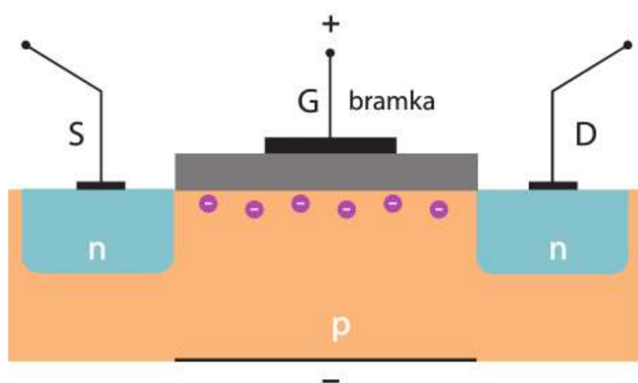
Ryc. 30.4. Bramka tranzystora podłączona do „+” napięcia sterującego przyciąga do kanału elektrony, które mogą tworzyć prąd elektryczny
