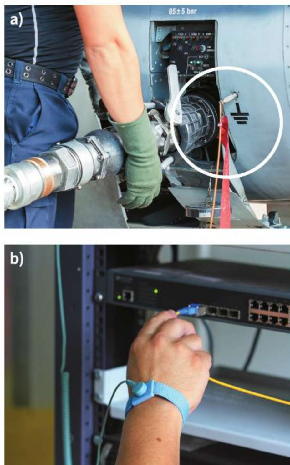
Ryc. 1.8. a) Podczas przepompowywania materiałów łatwopalnych zbiorniki muszą być uziemione. b) Pracownik naprawiający komputer połączony jest przewodem z jego obudową
