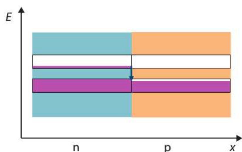
Ryc. 1. Pasma w momencie złączenia półprzewodników typu p i n
