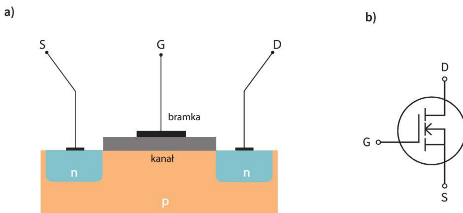
Ryc. 30.2. a) Przekrój tranzystora polowego; b) symbol tego typu tranzystora
