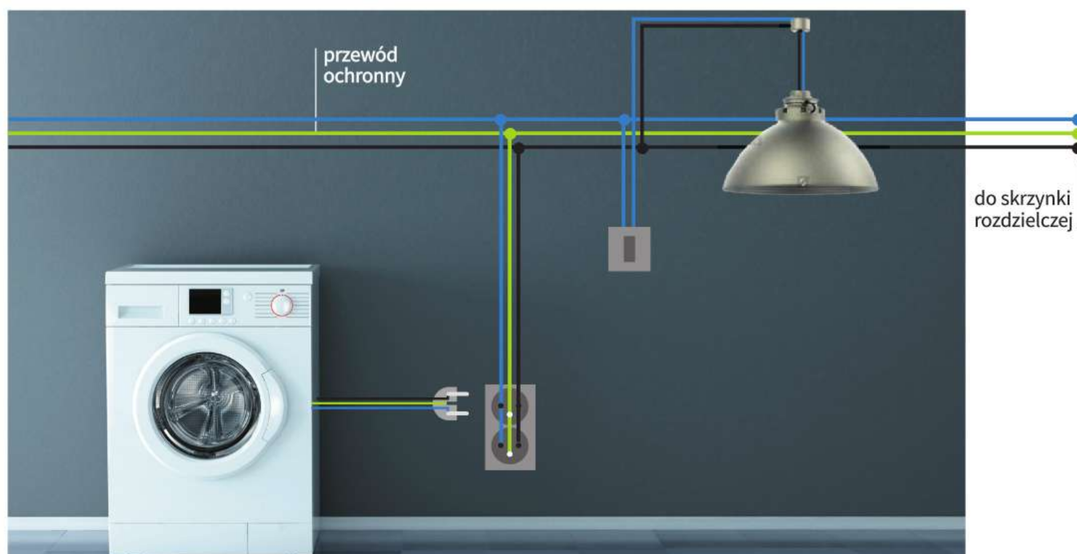
Ryc. 13.2. Schematyczne podłączenie dwóch przykładowych domowych urządzeń elektrycznych
