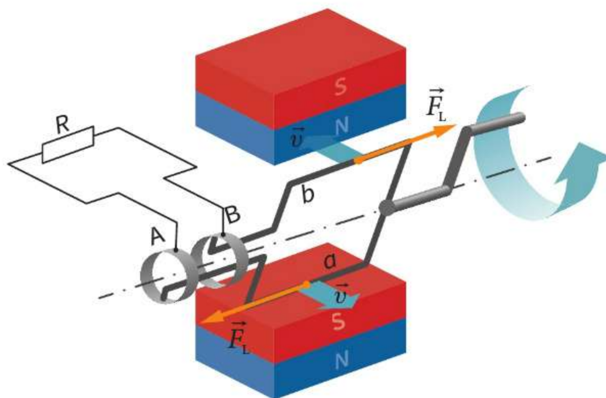
Ryc. 21.2. Model prądnicy
