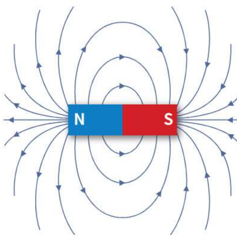
Ryc. 14.1. Układ igieł magnetycznych w pobliżu magnesu sztabkowego (a) i linie pola magnetycznego takiego magnesu (b)
