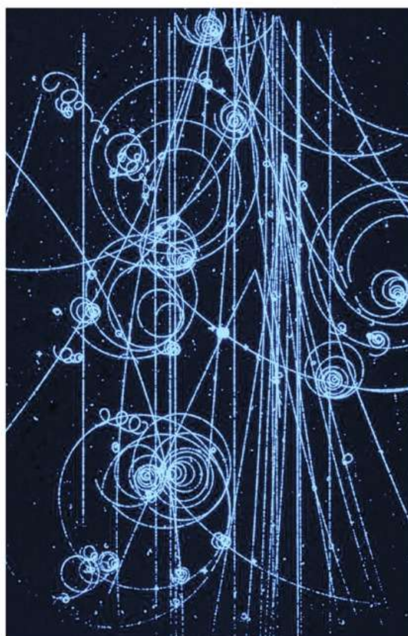
Ryc. 17.4. Ślady cząstek elementarnych w tzw. komorze pęcherzykowej
