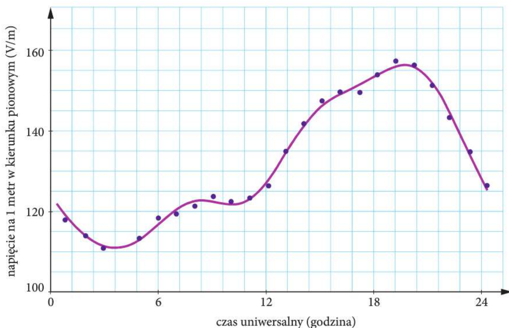
Dobowe zmiany pola elektrycznego wokół Ziemi
