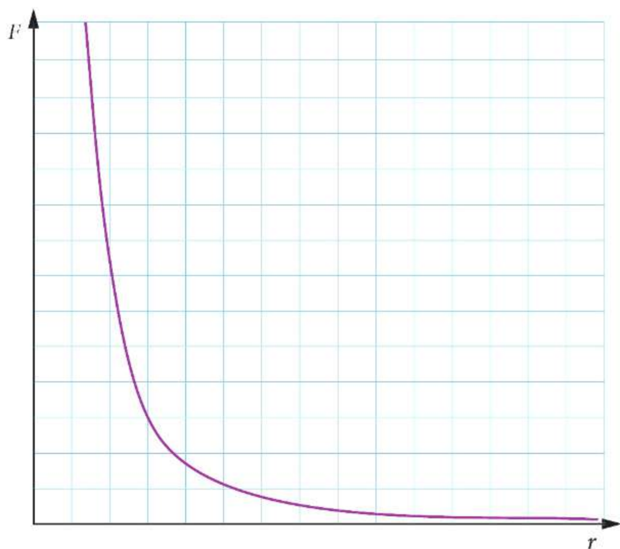
Ryc. 3.3. Wykres zależności wartości siły między dwoma ładunkami od ich wzajemnej odległości
