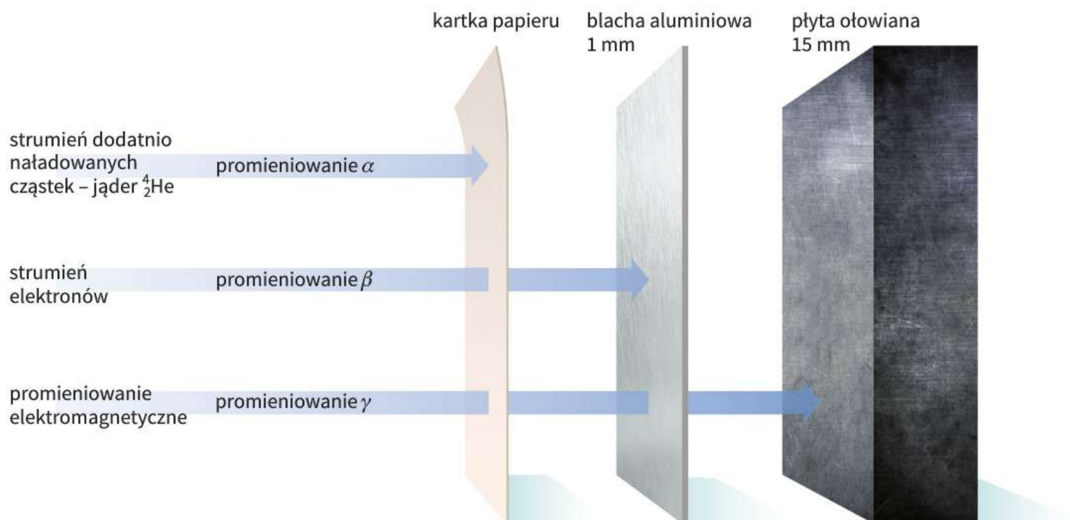
Ryc. 33.4. Przenikliwość promieniowania jądrowego
