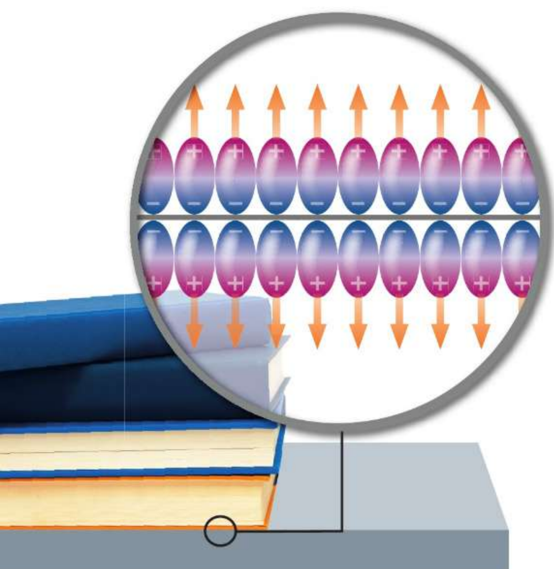
Ryc. 3.5. Wszystkie obiekty na biurku leżą na nim dzięki elektrycznemu odpychaniu się atomów i cząsteczek
