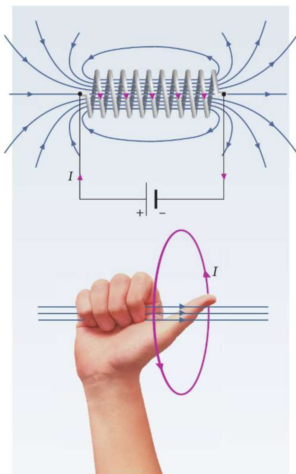
Ryc. 15.4. Kierunek linii pola magnetycznego wewnątrz zwojnicy i kierunek prądu są względem siebie prawoskrętne
