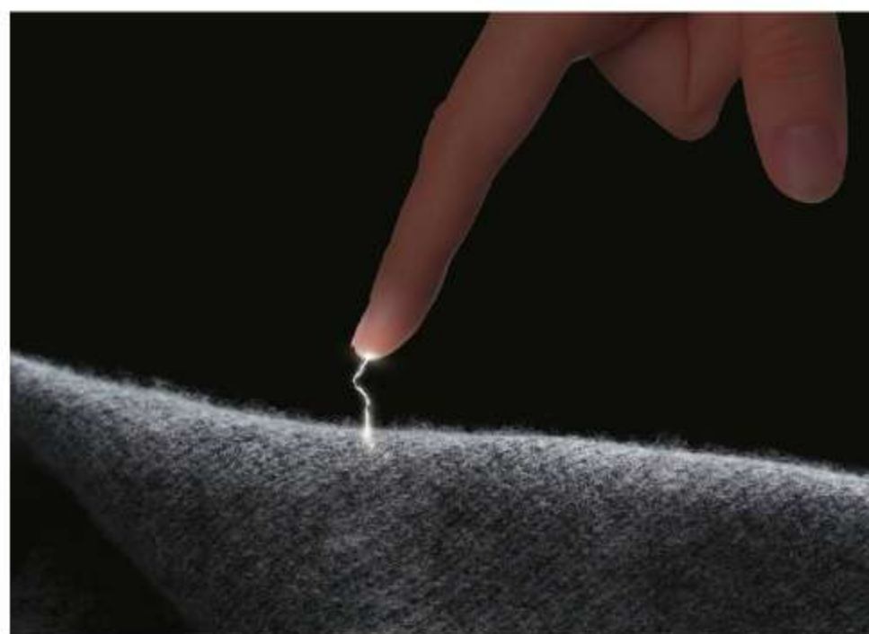
Ryc. 1.7. Odpłynięcie ładunku do Ziemi: przez uziemienie (a) oraz przez iskrę i nasze ciało (b)
