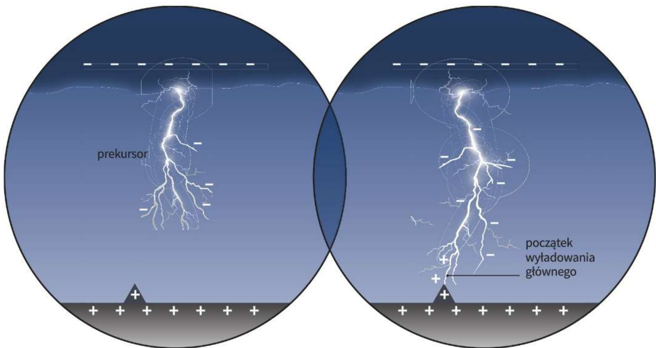
Ryc. 8.6. Schemat powstawania wyładowania wstępnego (prekursora) oraz głównego podczas burzy
