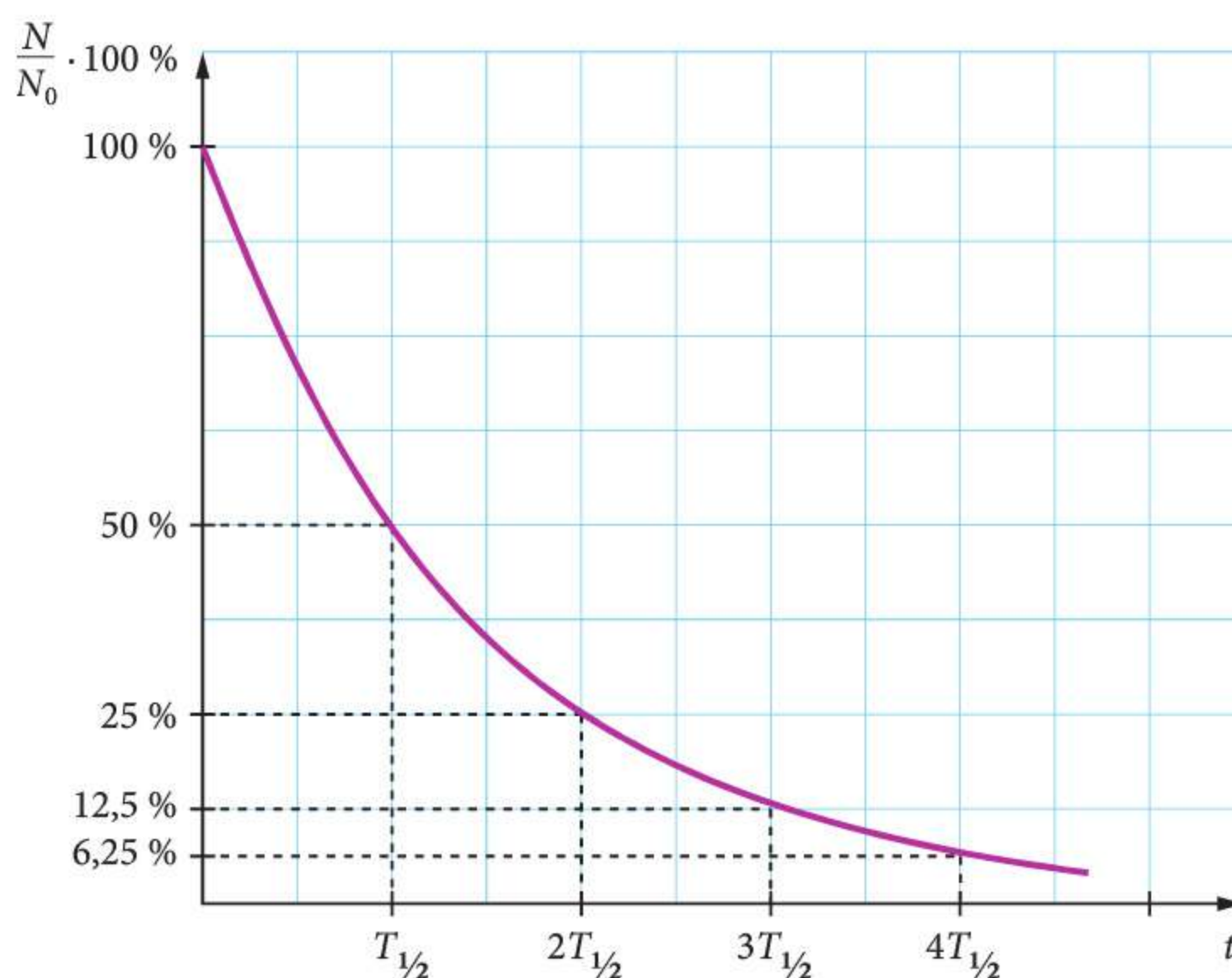
Ryc. 34.4. Zależność procentowej zawartości jąder dowolnego izotopu promieniotwórczego od czasu
