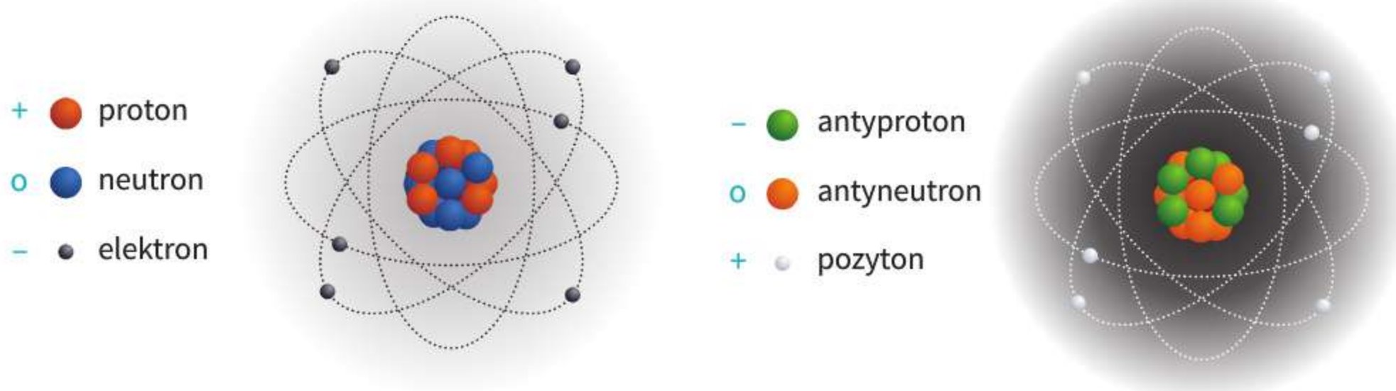
Ryc. 2. Modele atomu materii i atomu antymaterii
