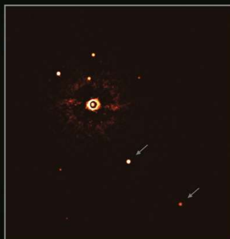
Ryc. 43.4. Zdjęcie gwiazdy TYC 8998-760-1 z dwiema planetami
