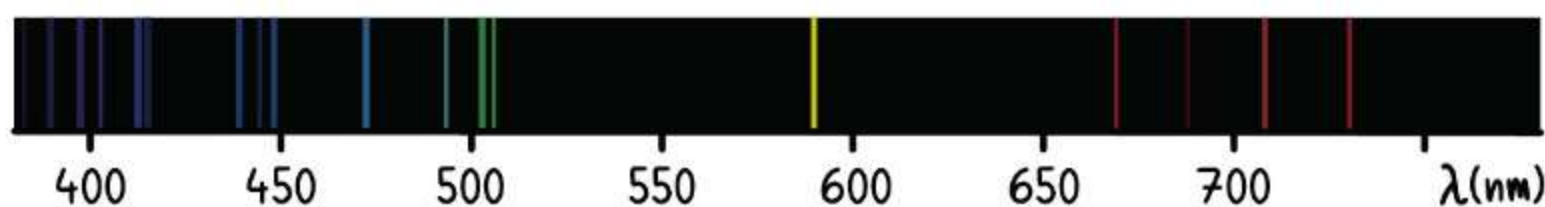
widmo emisyjne helu (przykład widma liniowego)
