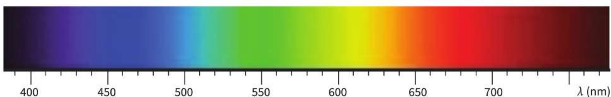
Ryc. 25.2. Widmo ciągłe źródła termicznego z podziałką długości fali
