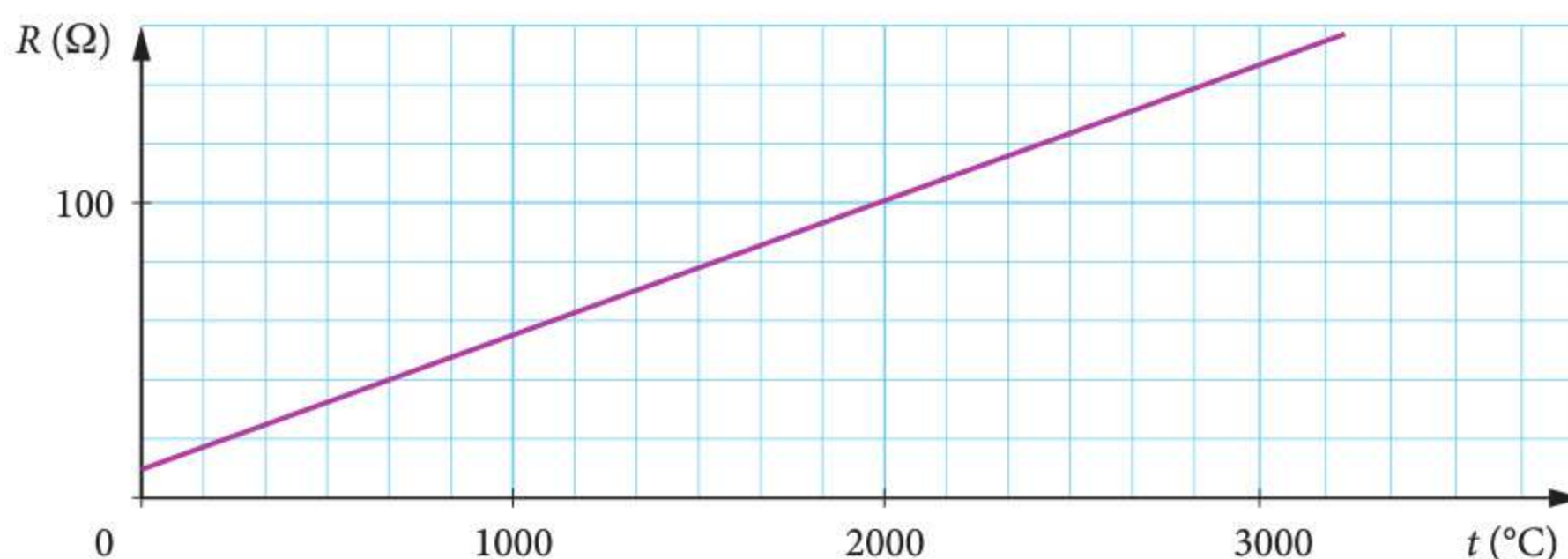
Ryc. 10.6. Zależność oporu drucika wolframowego żarówki od temperatury
