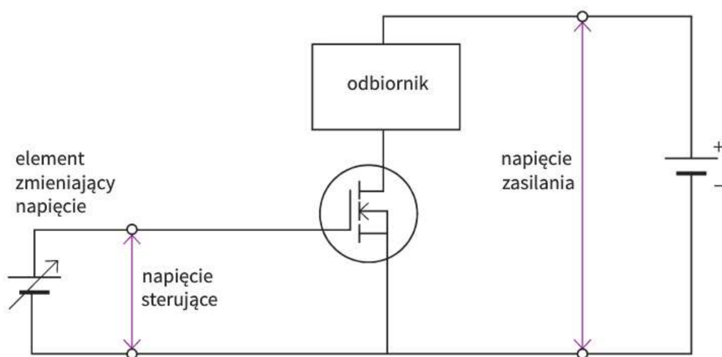
Ryc. 30.3. Podłączenie tranzystora umożliwiające sterowanie prądem płynącym przez odbiornik energii elektrycznej
