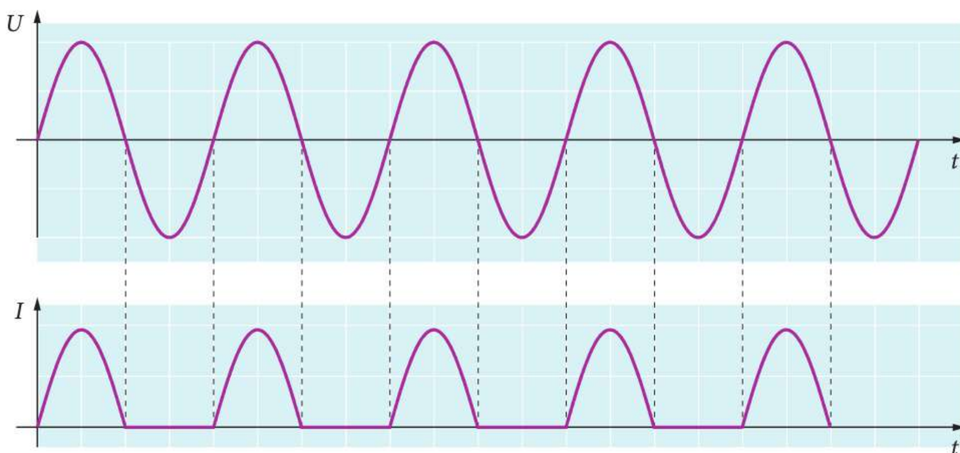
Ryc. 29.5. Napięcie na źródle zasilania i natężenie prądu w obwodzie z diodą w zależności od czasu
