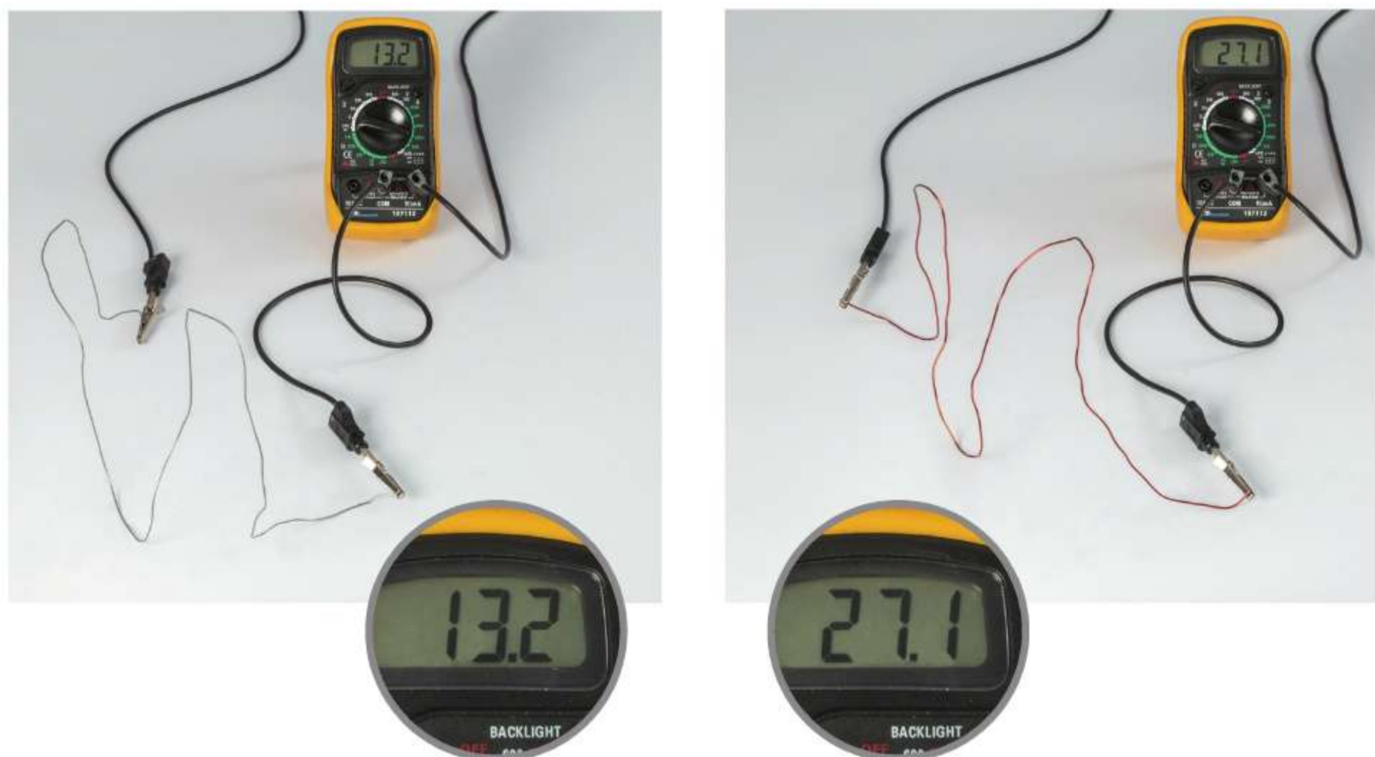
Ryc. 10.1. Pod wpływem tego samego napięcia przez różne przewody płynie prąd o różnym natężeniu
