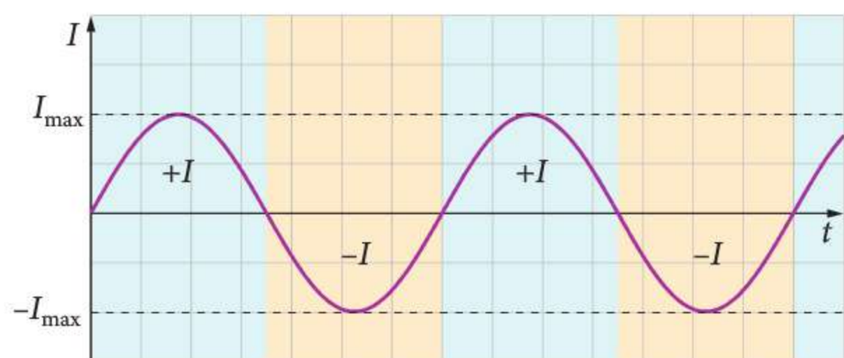
Ryc. 22.1. Schemat obwodu z prądnicą prądu przemiennego oraz wykresy zależności napięcia na zaciskach prądnicy i natężenia prądu w obwodzie od czasu
