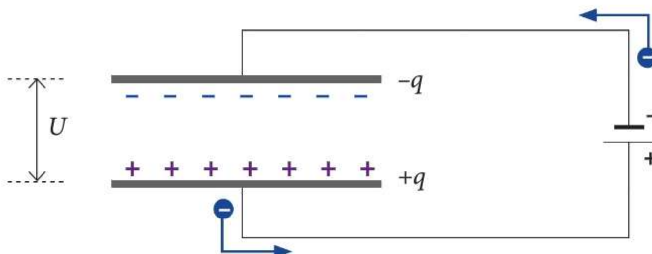
Ryc. 7.3. Podczas ładowania kondensatora źródło napięcia wykonuje pracę równą energii naładowanego kondensatora
