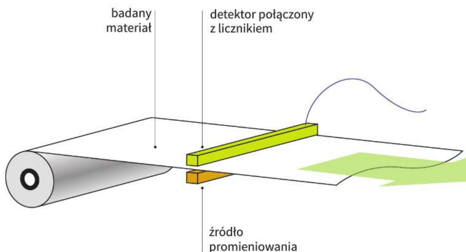
Ryc. 36.4. Detektor promieniowania pozwala na pomiar grubości materiału bez zatrzymywania taśmy
