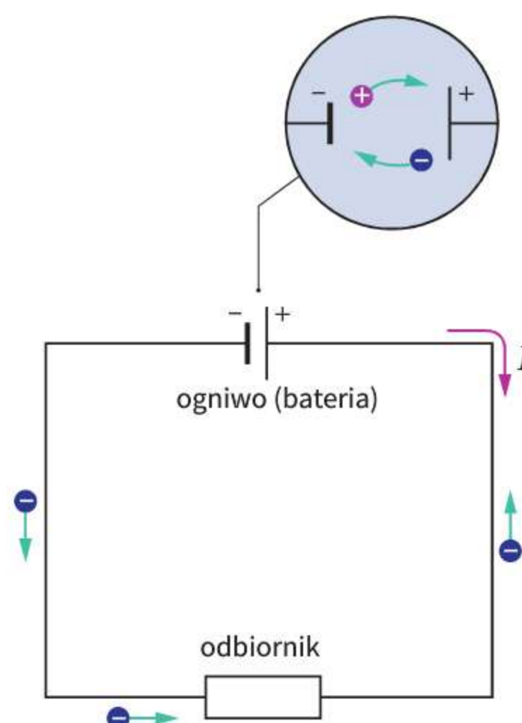
Ryc. 9.3. Ogniwo wymusza przepływ ładunków w obwodzie
