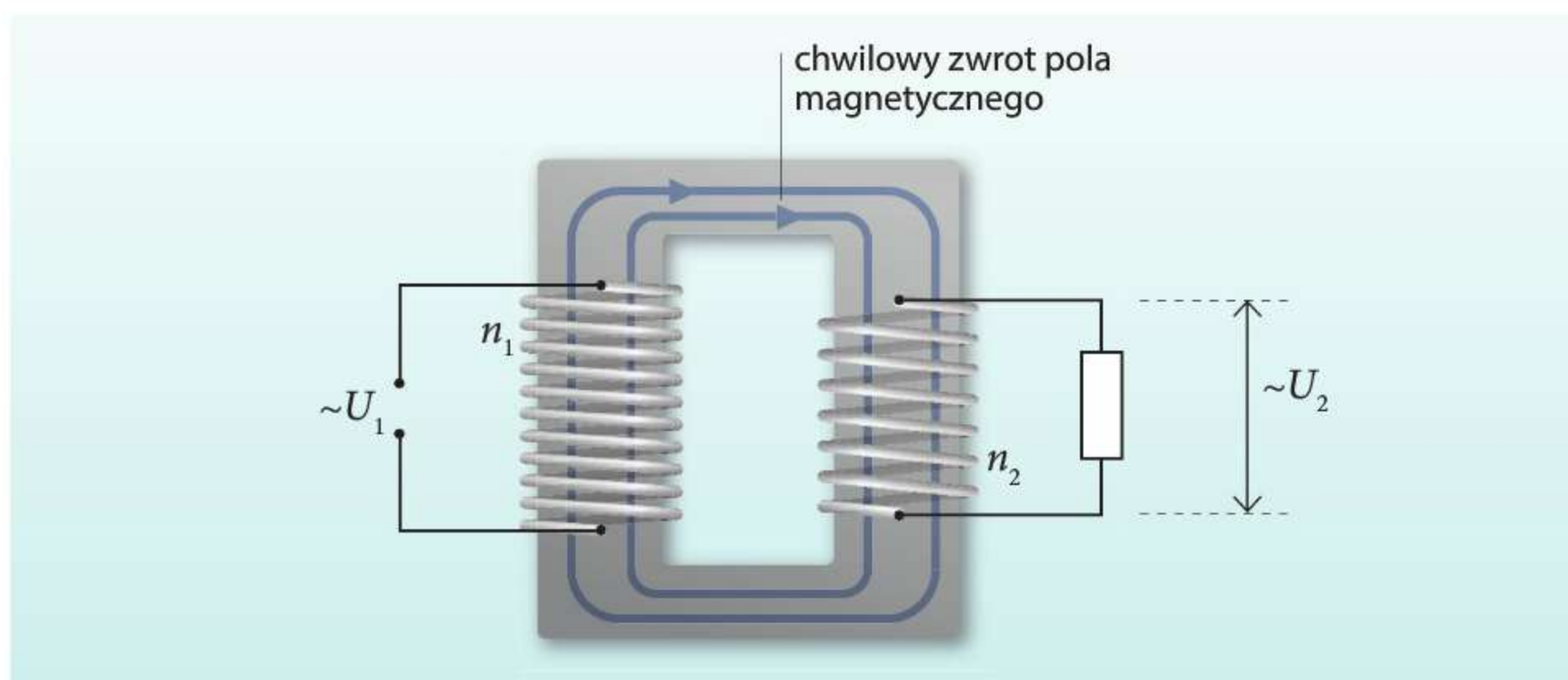
Ryc. 23.2. Schemat działania transformatora, gdzie: U_1 i U_2 – napięcia na uzwojeniu pierwotnym i wtórnym, a n_1 i n_2 – liczba zwojów uzwojenia pierwotnego i wtórnego.
