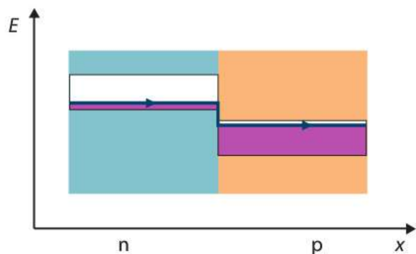
Ryc. 29.3. Kierunek ruchu elektronów tworzących prąd w diodzie
