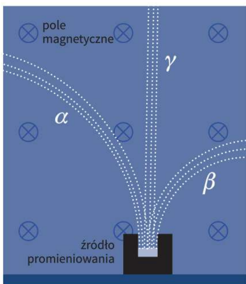
Ryc. 33.1. W polu magnetycznym promieniowanie \alpha i promieniowanie \beta mogą poruszać się po zakrzywionym torze
