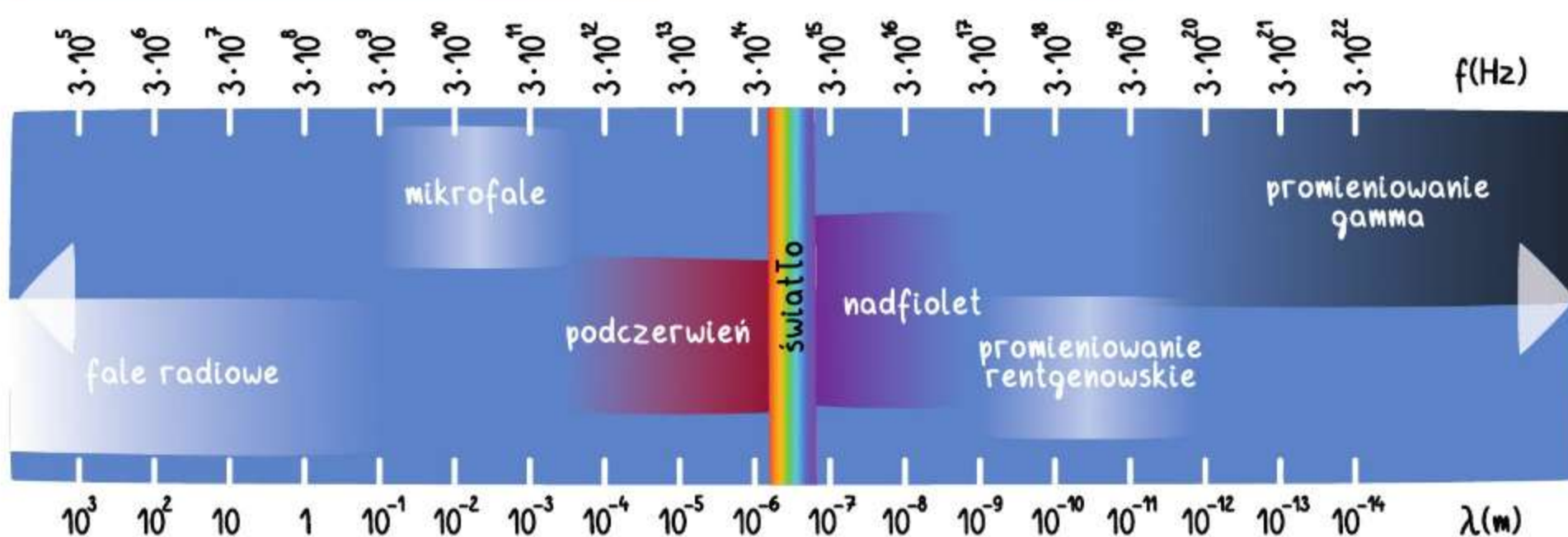
widmo ciągłe światła
