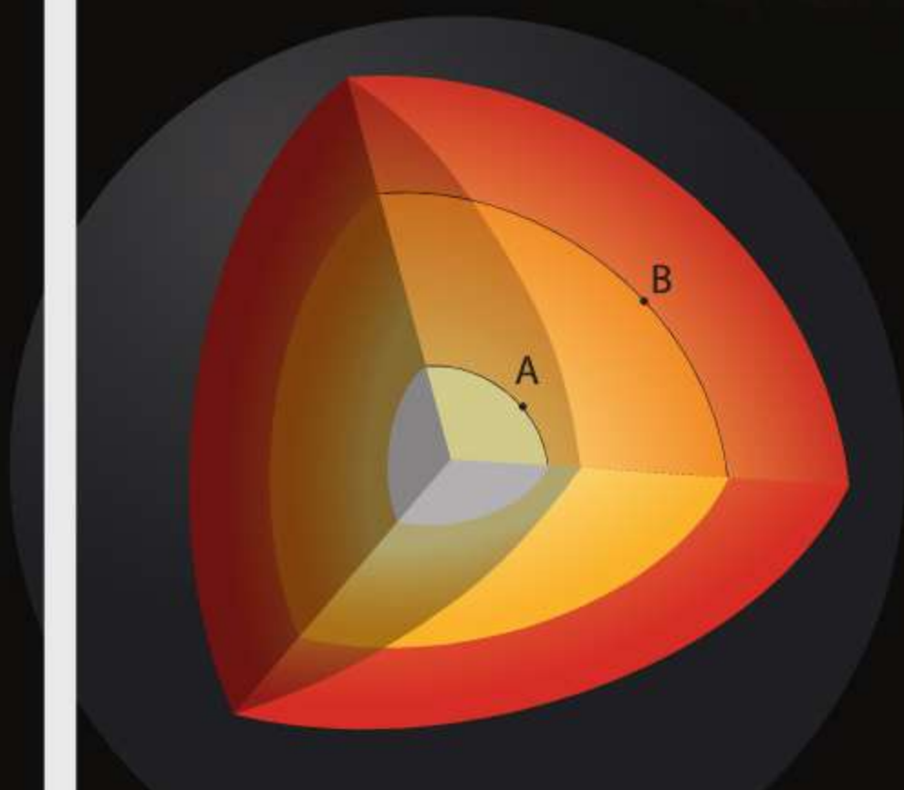
Ryc. 43.6. Ciśnienie na powierzchni B musi zrównoważyć ciężar jednej warstwy (czerwonej), a ciśnienie na powierzchni A musi zrównoważyć ciężar dwóch warstw (czerwonej i pomarańczowej)
