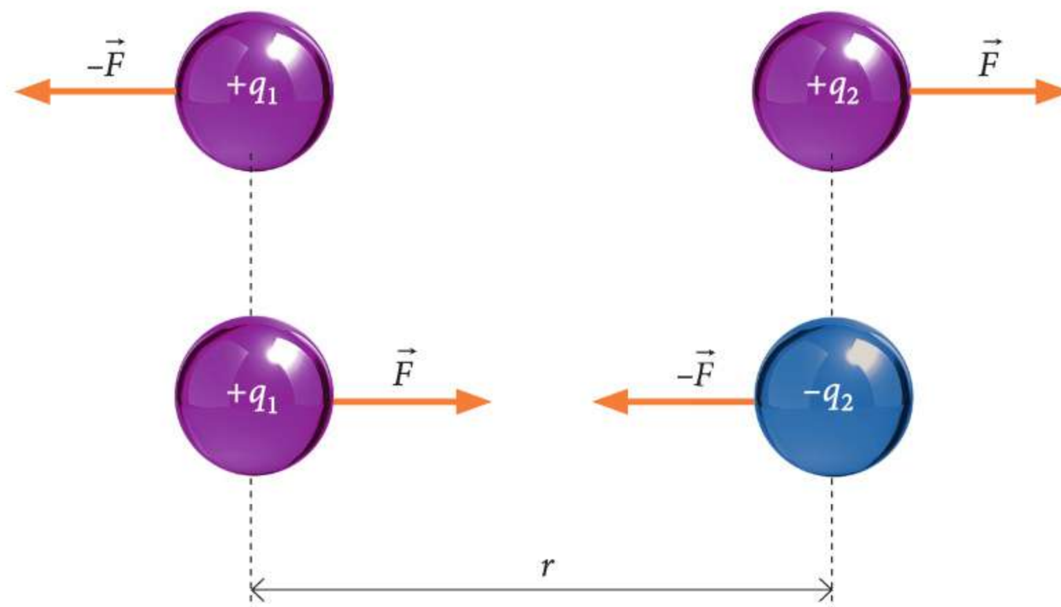
Ryc. 3.1. Oddziaływanie dwóch ładunków
