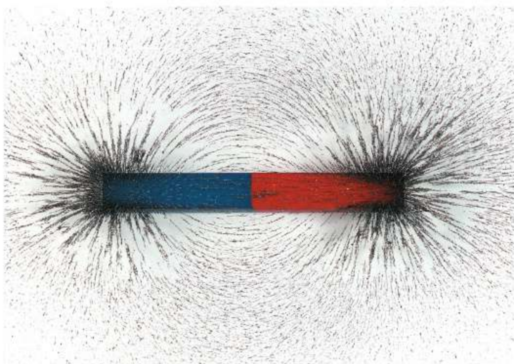
Ryc. 14.5. Pole magnetyczne magnesu zobrażowane za pomocą opiłków żelaza
