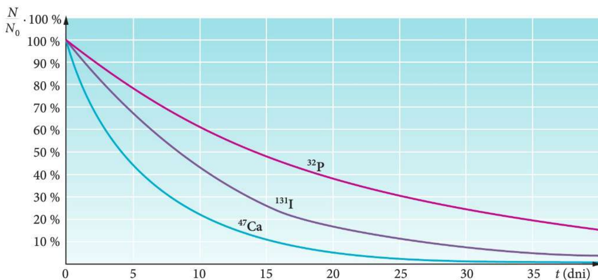
Ryc. 34.2. Wykresy zależności zawartości izotopu promieniotwórczego w próbce od czasu dla trzech różnych izotopów
