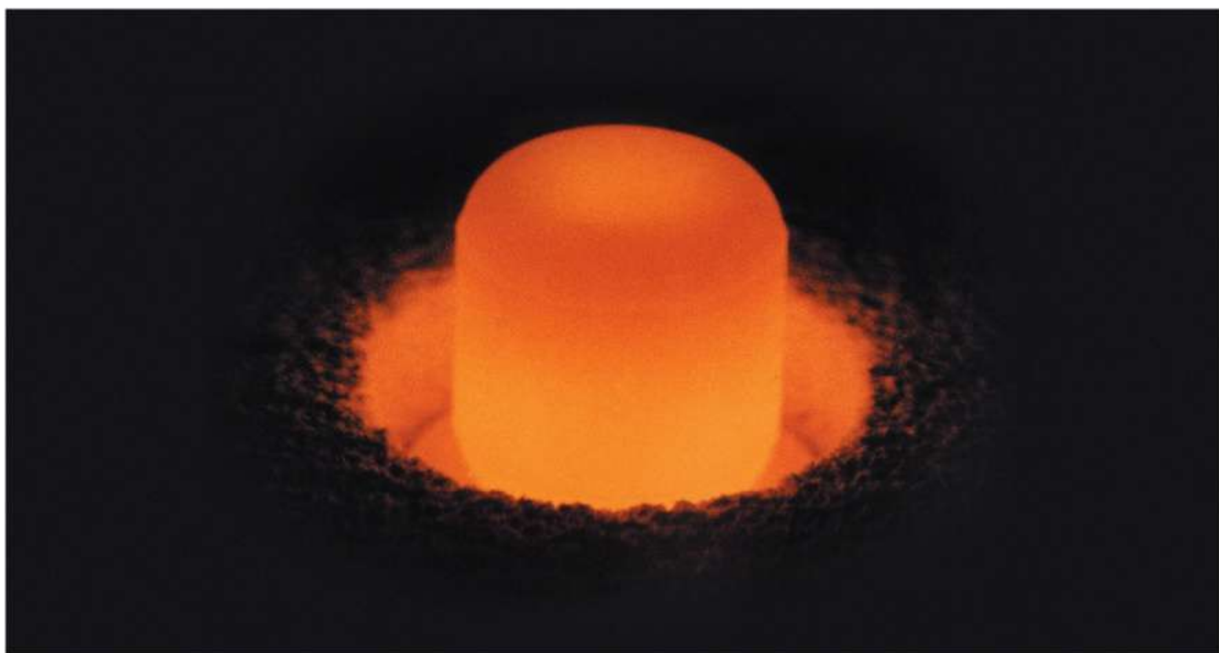
Próbka plutonu rozgrzana w wyniku reakcji rozpadu
