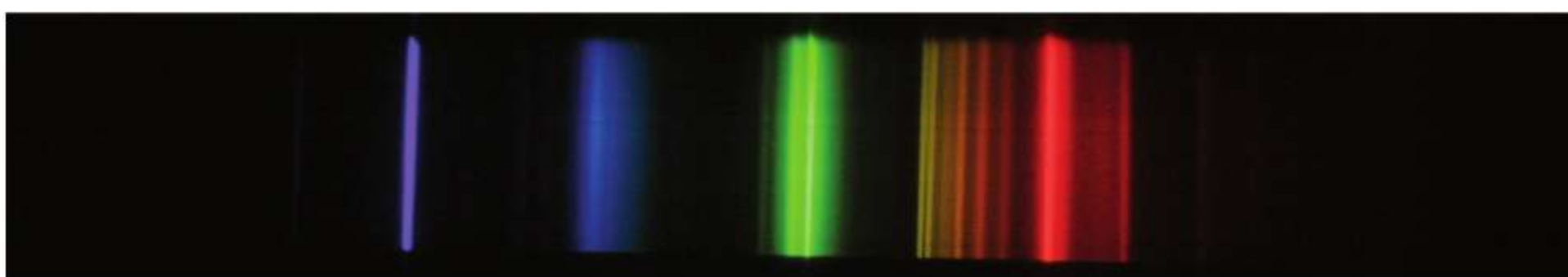
Ryc. 25.5. Widmo świetlówki uzyskane za pomocą spektroskopu zrobionego z płyty CD. Brakuje niektórych barw, więc widmo nazwiemy nieciągłym
