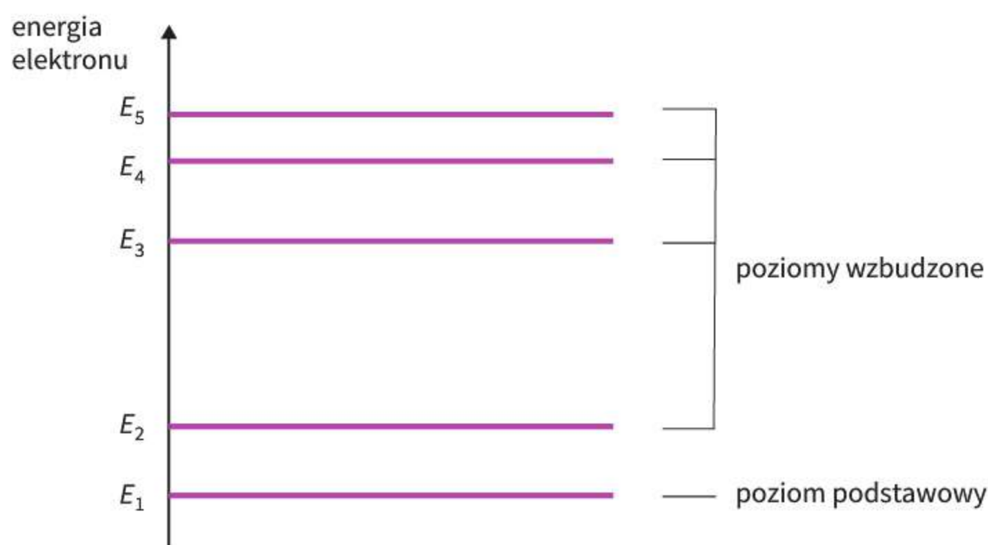
Ryc. 27.4. Poziomy energetyczne atomu – schemat
