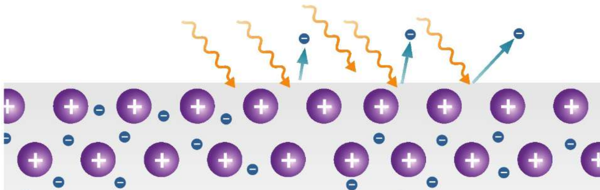
Ryc. 31.1. Podczas zjawiska fotoelektrycznego zewnętrznego elektrony są wybijane z powierzchni metalu
