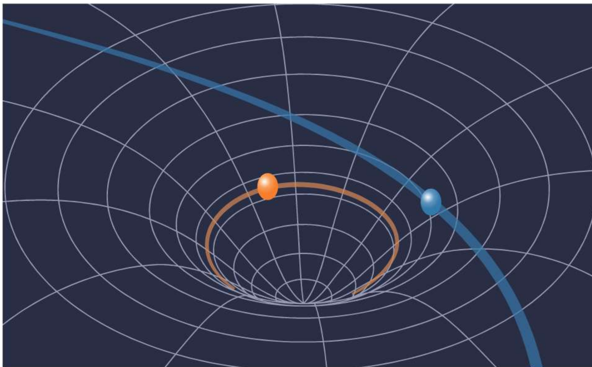
Ryc. 44.6. Gwiazda (w głębi leja) zakrzywia czasoprzestrzeń i powoduje grawitacyjne przyciąganie
