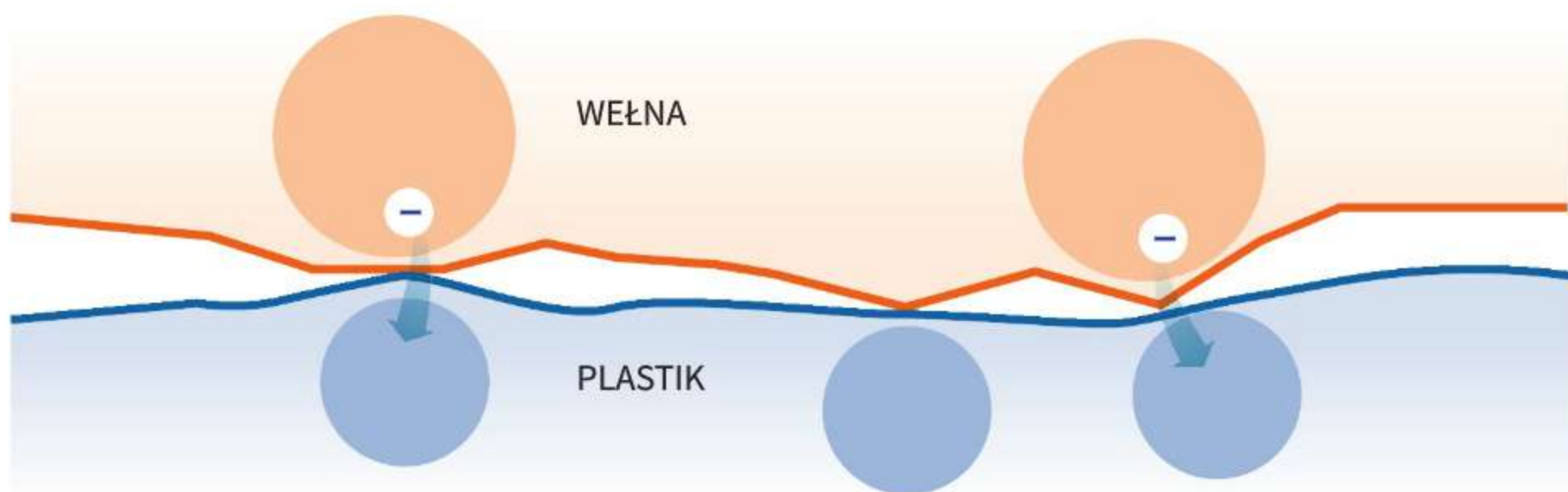
Ryc. 2.1. Elektrony we włóknach wełny są słabiej związane niż elektrony w plastiku. W miejscach bezpośredniego styku cząsteczki tworzące plastik przechwytyują elektrony, zatem plastik elektryzuje się ujemnie, a wełna dodatnio
