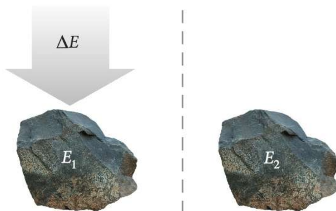
Ryc. 38.1. Przekaz energii zmieniający energię spoczynkową ciała
