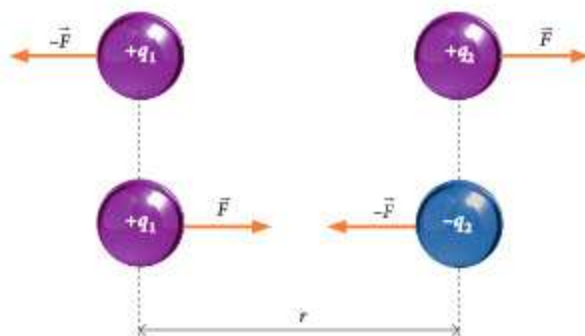
Ryc. 3.1. Oddziaływanie dwóch ładunków
