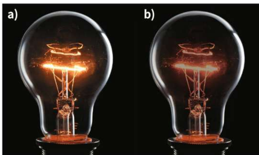
Ryc. 25.3. Dwa widma tej samej żarówki zasilanej wyższym (a) i niższym (b) napięciem. Natężenie koloru niebieskiego w widmie jest wyraźnie słabsze, gdy temperatura włókna żarówki jest niższa
