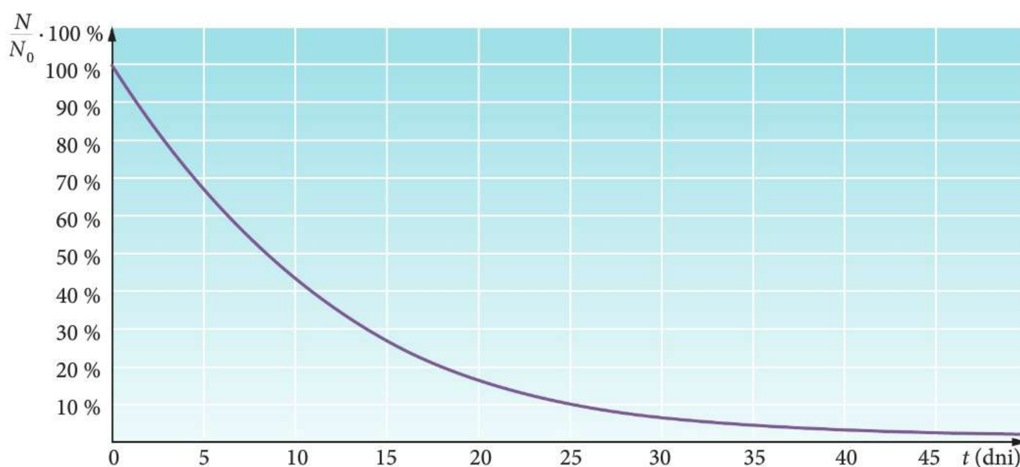
Ryc. 34.3. Wykres zależności zawartości procentowej izotopu jodu ^{131}\text{I} w próbce od czasu
