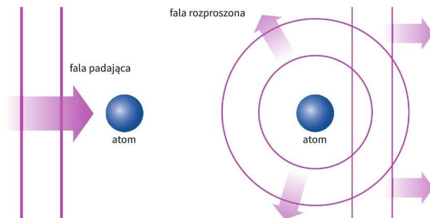
Ryc. 26.2. Fala płaska rozpraszana na atomie
