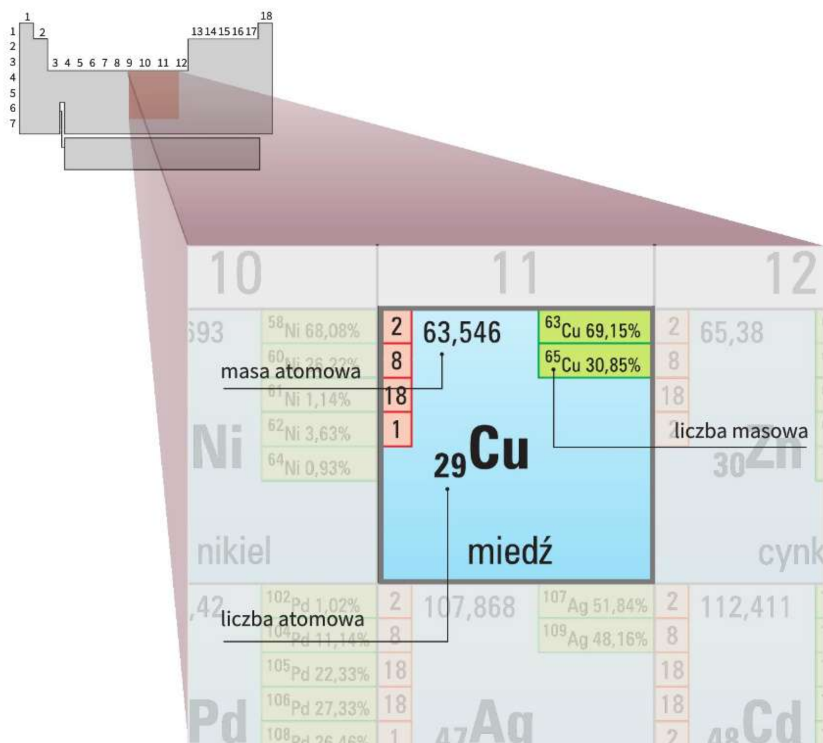
Ryc. 32.2. W układzie okresowym pierwiastków są zawarte informacje o składzie jądra atomowego danego pierwiastka
