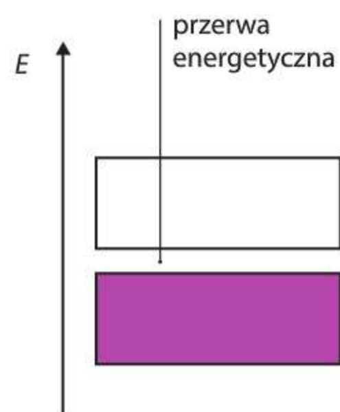
Ryc. 28.6. Pasma energetyczne półprzewodnika
