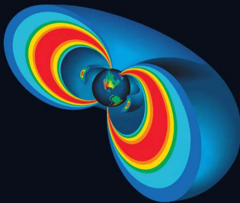
Ryc. 18.4. Cząstki naładowane przechwycone przez ziemskie pole magnetyczne tworzą pasy Van Allena. Kolor czerwony symbolizuje największe zagęszczenie cząstek
