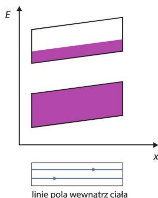
Ryc. 28.4. Dwa najwyższe pasma energetyczne metalu, obsadzone elektronami, w polu elektrycznym
