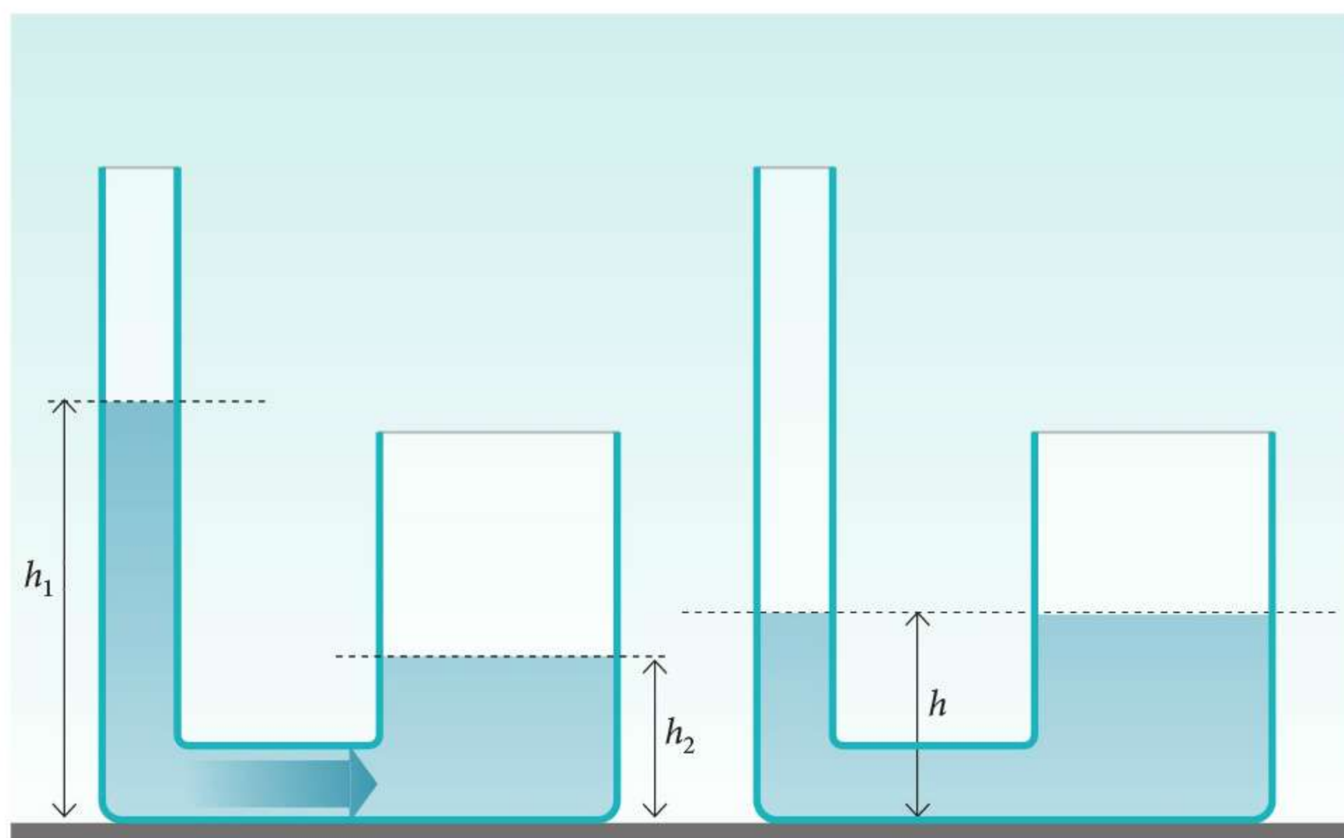
Ryc. 6.7. Przepływ wody trwa do czasu wyrównania jej poziomów
