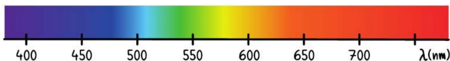
widmo ciągłe światła
