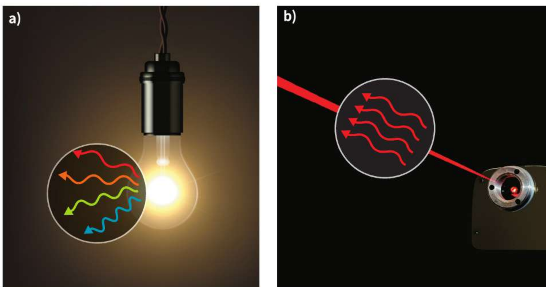
Ryc. 26.5. a) Światło wyemitowane przez żarówkę składa się z fotonów o różnych energiach i kierunkach ruchu. b) Wiązka światła laserowego to wąski strumień identycznych fotonów poruszających się w jedną stronę
