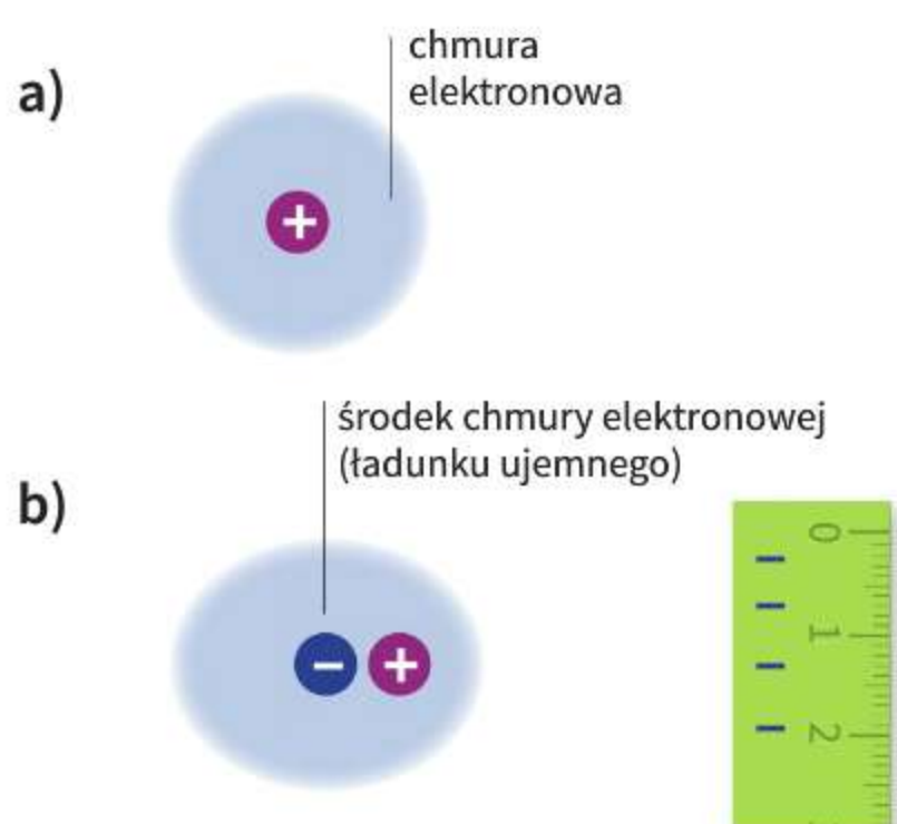
Ryc. 2.5. Rozmieszczenie ładunków w atomie z dala od innych ładunków (a) i w obecności ładunku zewnętrznego (b)
