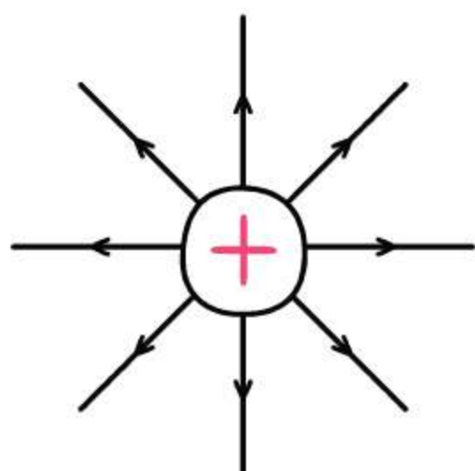
pole elektryczne wokół ładunku dodatniego
