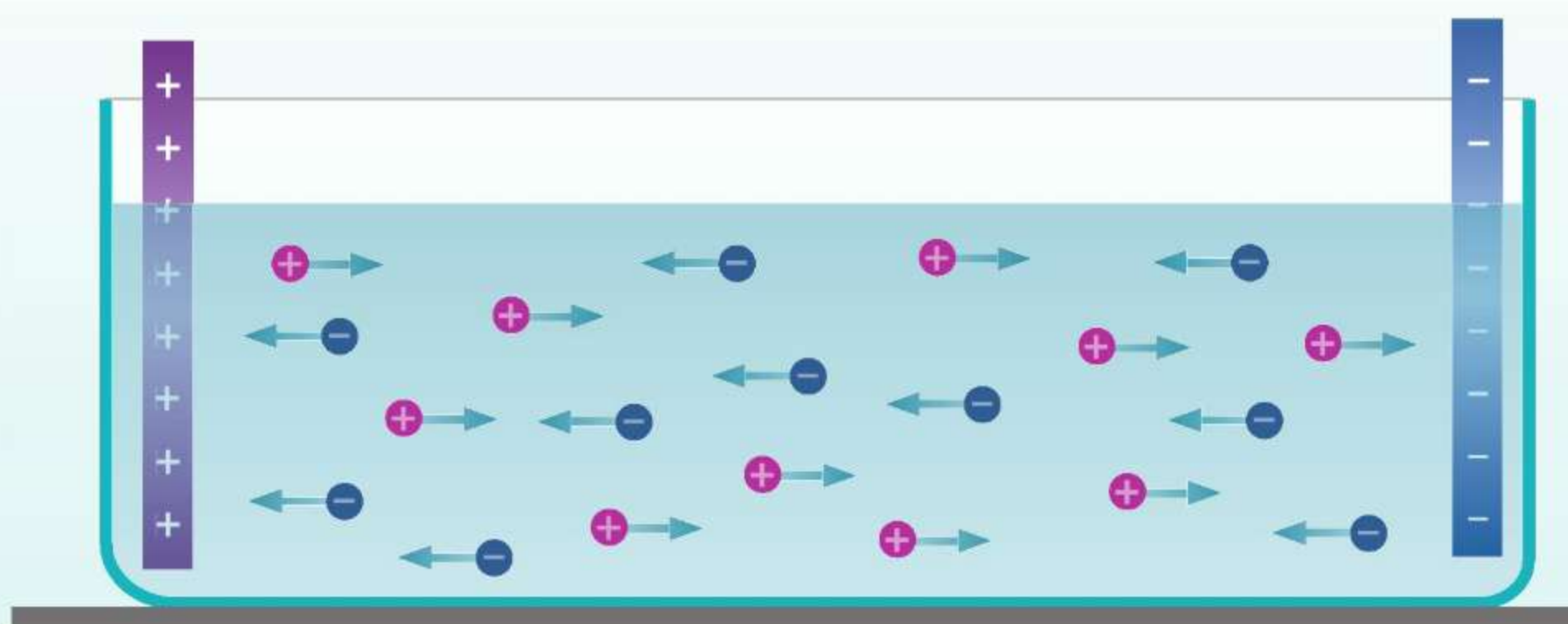
Ryc. 9.8. Prąd w cieczach tworzą jony ujemne i dodatnie
