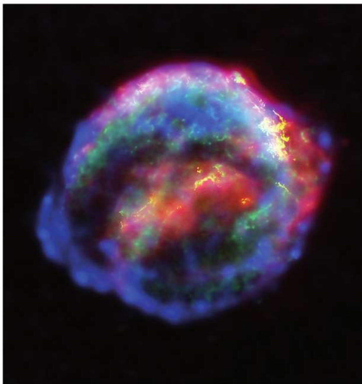
Ryc. 44.4. Pozostałość po supernowej z 1604 roku
