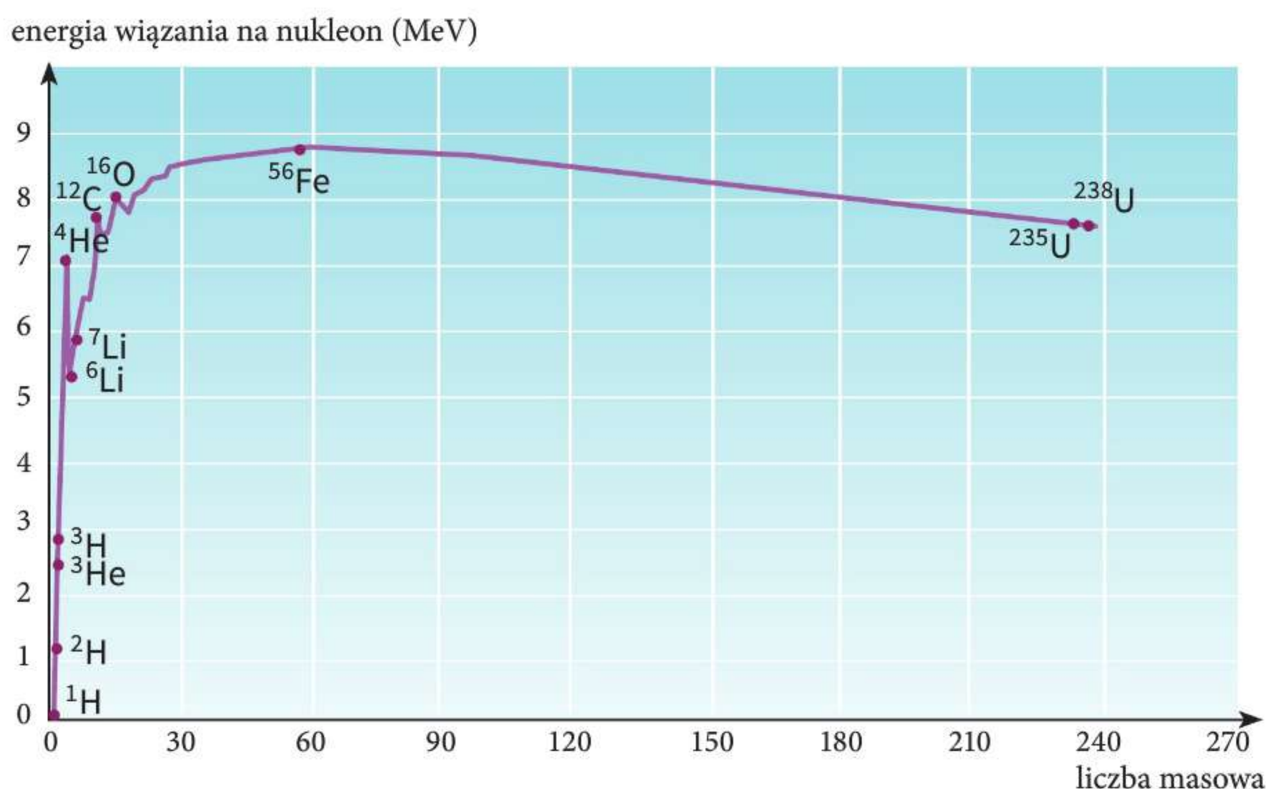
Ryc. 37.2. Zależność energii wiązania na nukleon od liczby masowej
