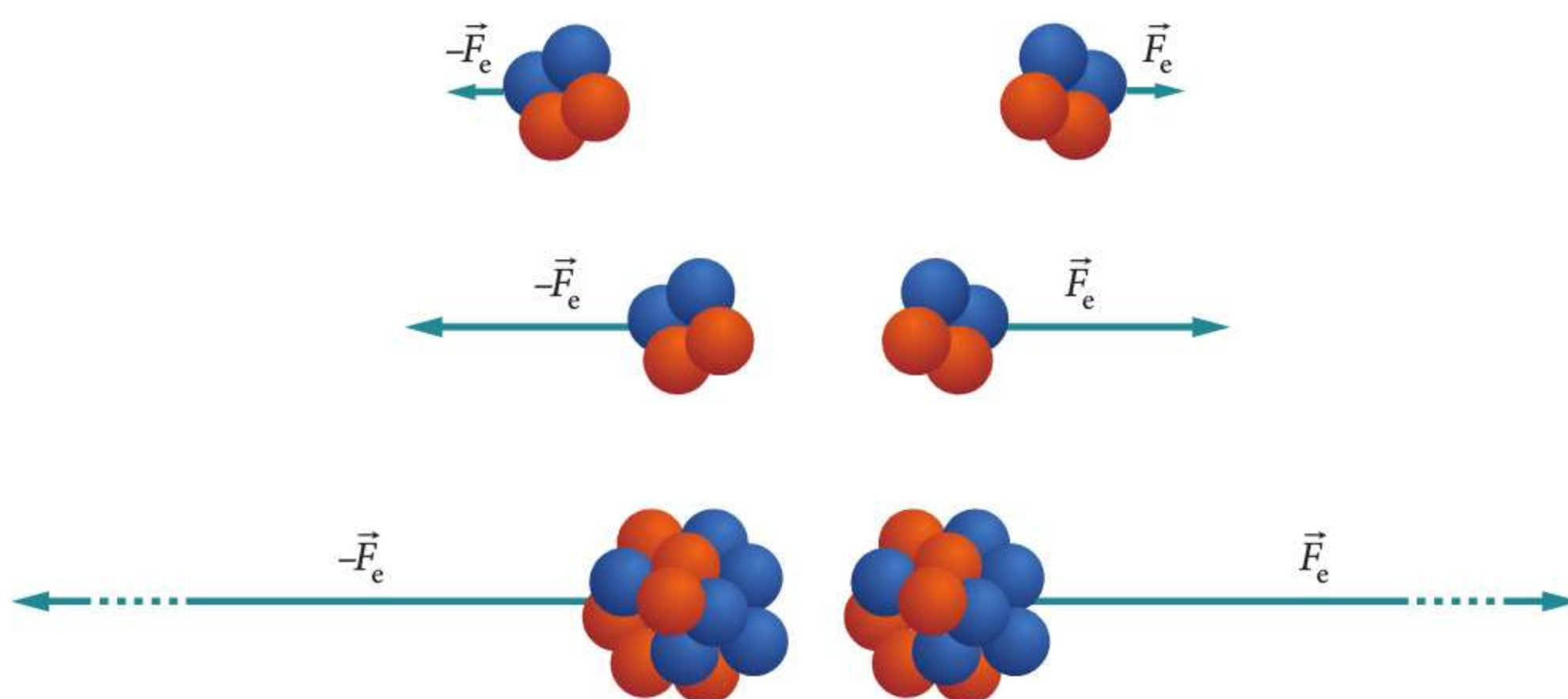
Ryc. 42.4. Jądra atomowe odpychają się siłami elektrycznymi
