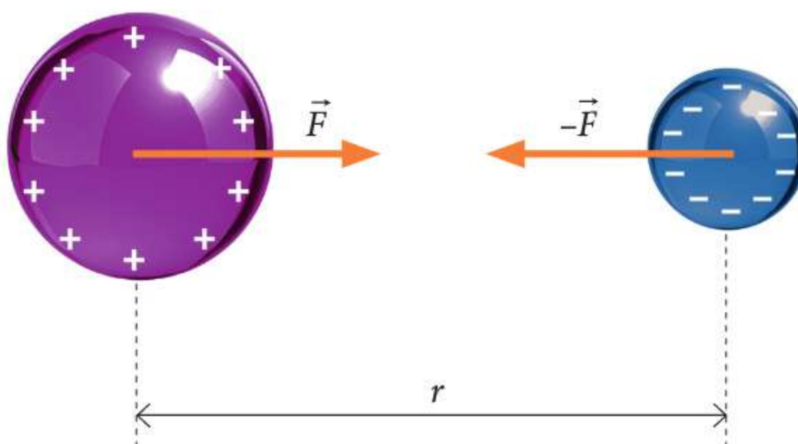
Ryc. 3.2. Siły między dwiema równomiernie naelektryzowanymi kulami
