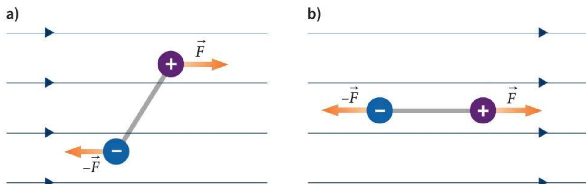
Ryc. 4.6. Dipol w polu elektrycznym ustawia się zgodnie z liniami pola, czyli zgodnie z działaniem sił elektrycznych
