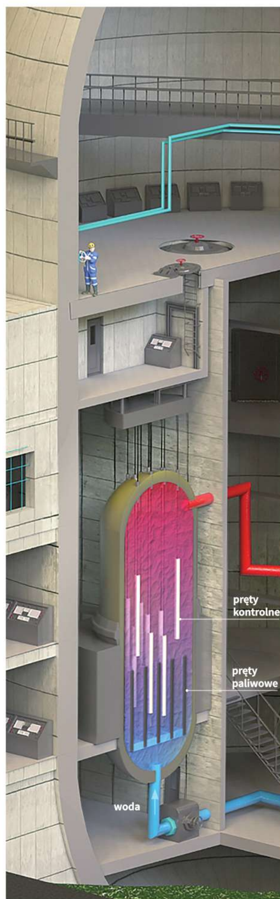
Ryc. 40.4. Schemat budowy reaktora wodnego
