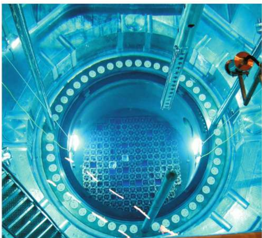
Ryc. 40.3. Reaktor wodny. Pręty paliwowe mocuje się w specjalnych stojakach, reaktor napełnia się wodą i szczelnie zamyka
