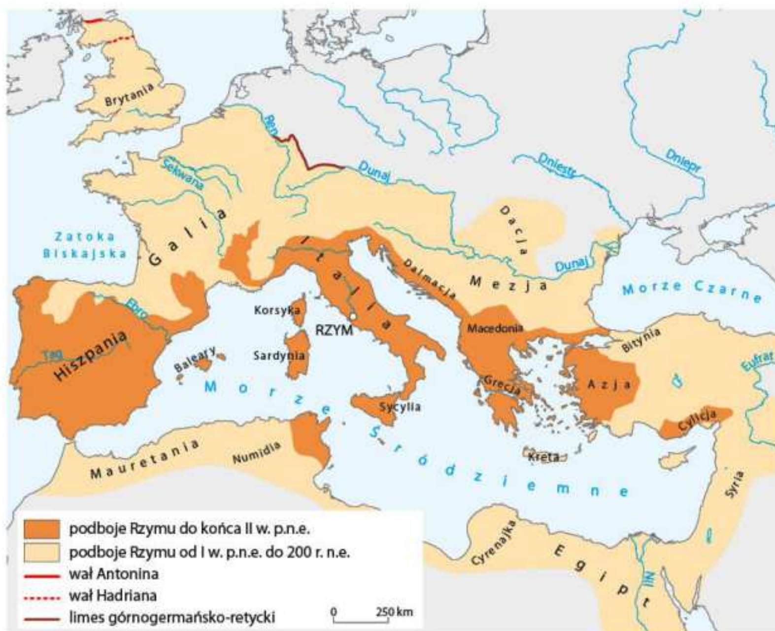
Cesarstwo Rzymskie ok. 200 r. n.e.
