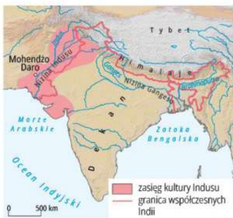
Położenie geograficzne Indii i cywilizacji doliny Indusu
