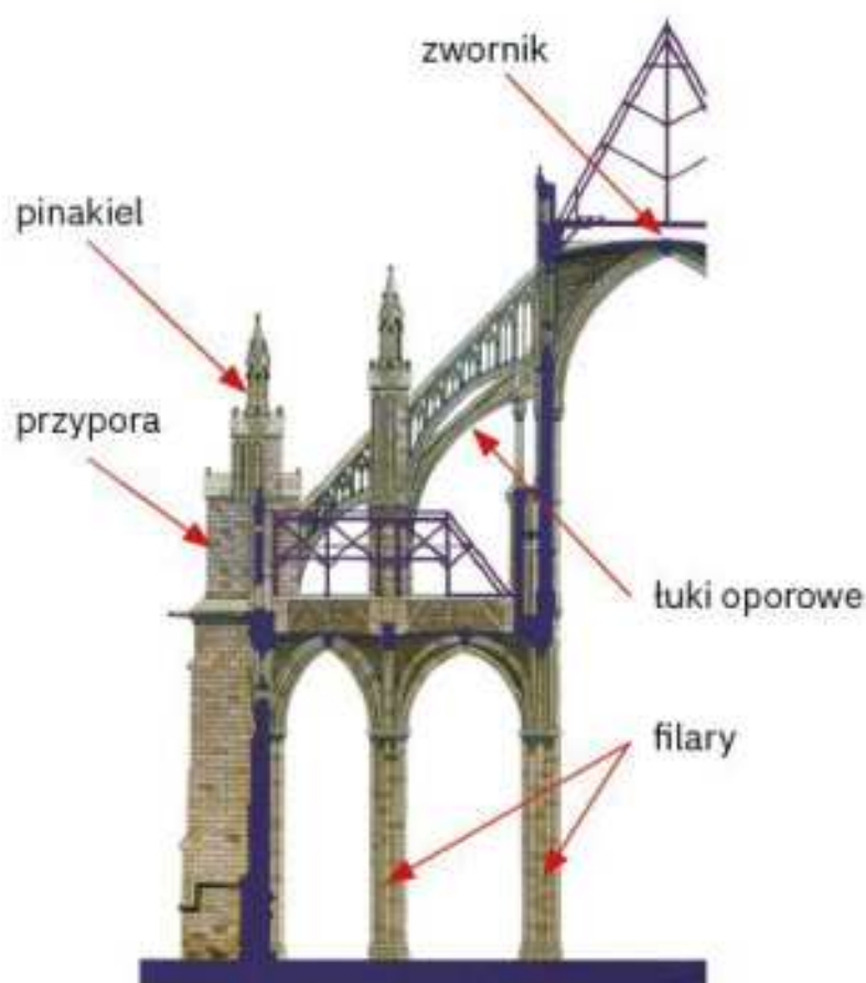
Elementy konstrukcyjne gotyckiej katedry w Amiens (czytaj: amję) we Francji, XIII w.
