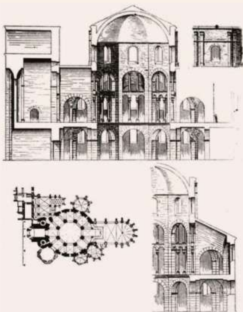
Plan i przekrój kaplicy pałacowej w Akwizgranie
