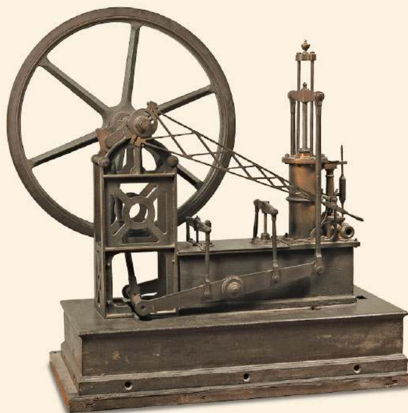
▲ Model maszyny parowej z tłokiem pionowym – konstrukcji Jamesa Watta. Zbiory Muzeum Miasta Stołecznego Warszawy.
