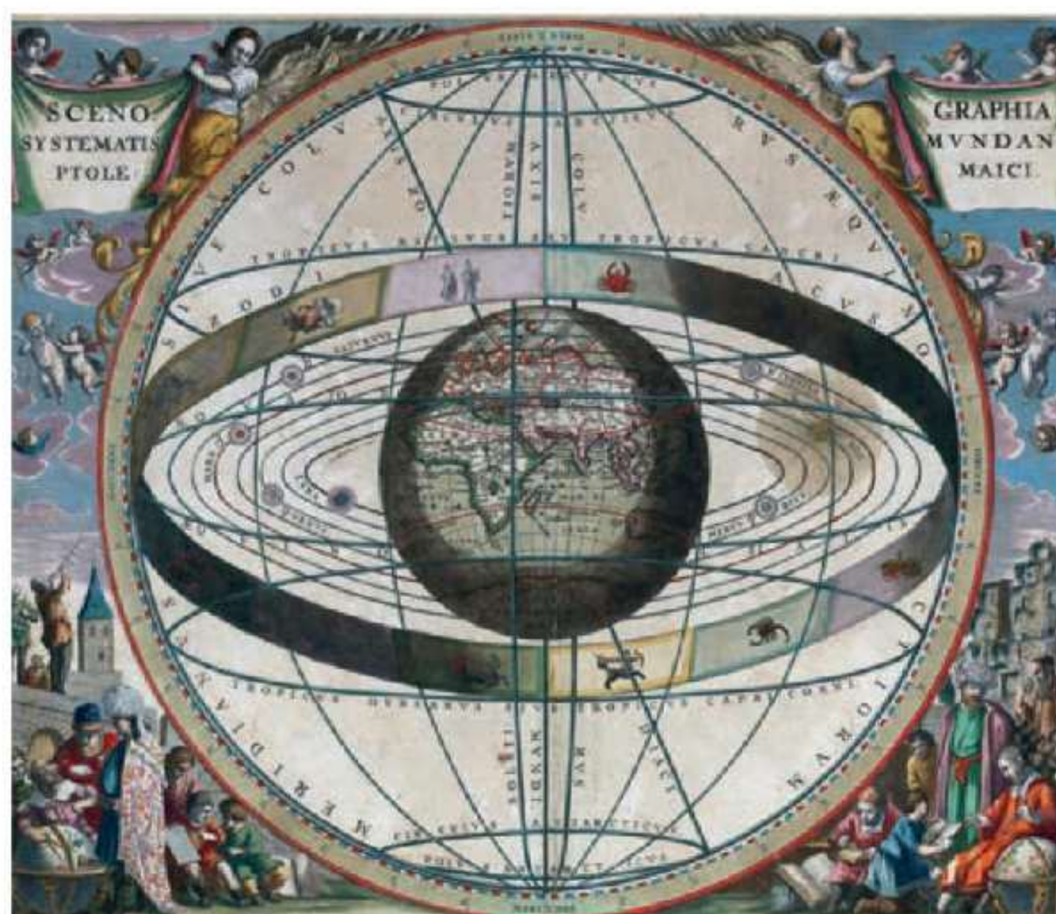
Wyobrażenie wszechświata przed odkryciem Kopernika: wokół nieruchomej Ziemi krążą Słońce, Księżyc i planety. Ilustracja z 1660 r.
