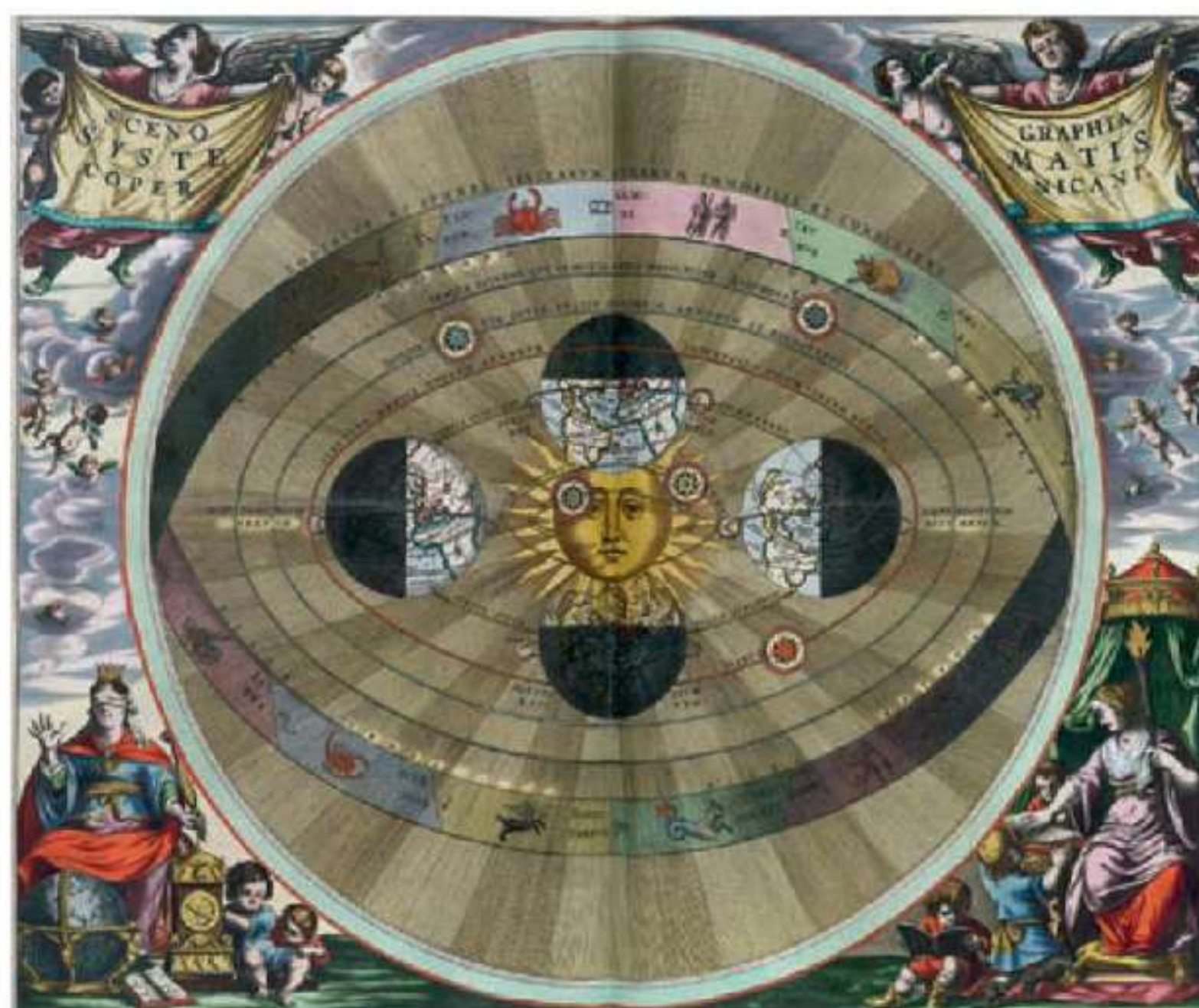
Wyobrażenie wszechświata po odkryciu Kopernika: wokół nieruchomego Słońca krążą Ziemia, Księżyc i inne planety. Ilustracja z 1660 r.
