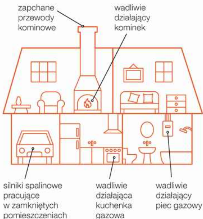
Przykłady źródeł tlenku węgla w gospodarstwie domowym.
