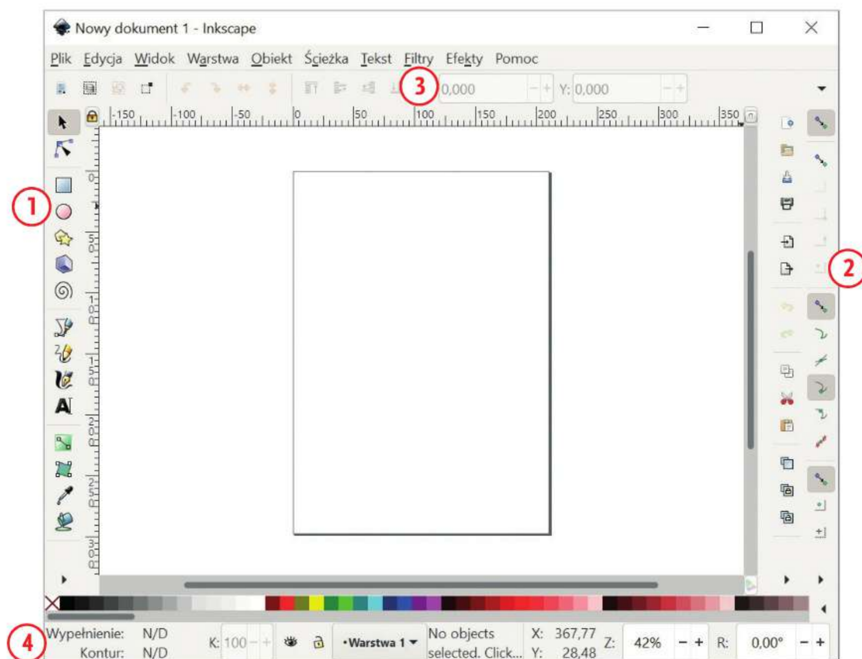
Rys. 1. Okno Inkscape'a
