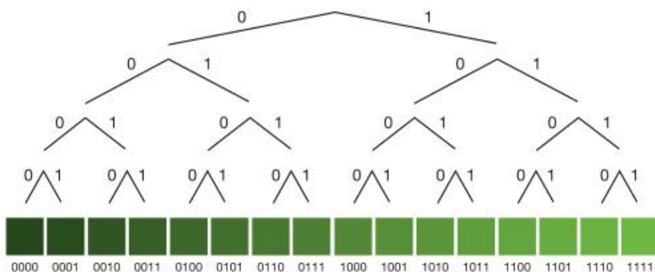
Rys. 12.8. Diagram ilustrujący tworzenie kodów odcieni w obrazie
