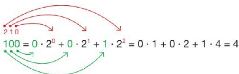
Rys. 7.9. Schemat zamiany liczby binarnej na dziesiętną
