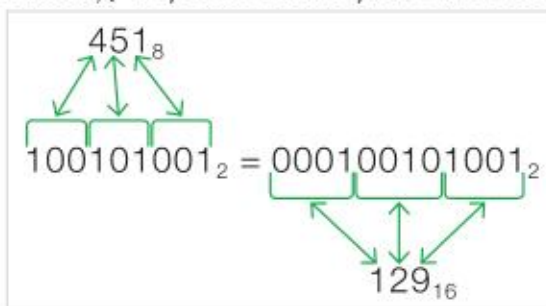
Rys. 12.3. Zamiana zapisu liczby pomiędzy systemami dwójkowym, ósemkowym i szesnastkowym
