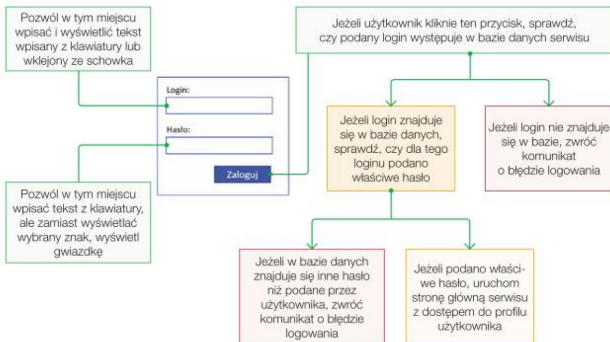
Rys. 10.1. Logowanie do serwisu internetowego – opis działania elementów
