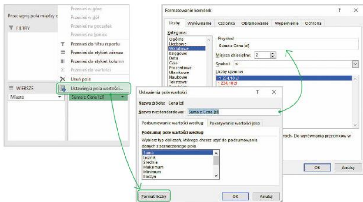
Rys. 2.18. Formatowanie liczb w tabeli przestawnej
