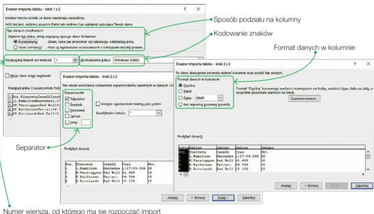
Rys. 1.11. Kreator importu danych z pliku tekstowego
