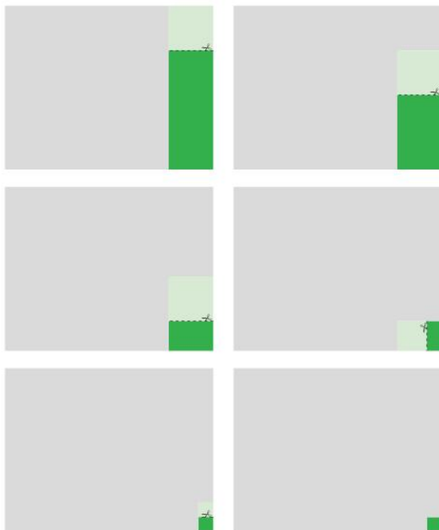
Rys. 14.4. Kolejne kroki wycinanki Euklidesa
