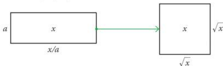
Rys. 5.2. Interpretacja geometryczna szukania przybliżenia liczby \sqrt{x}
