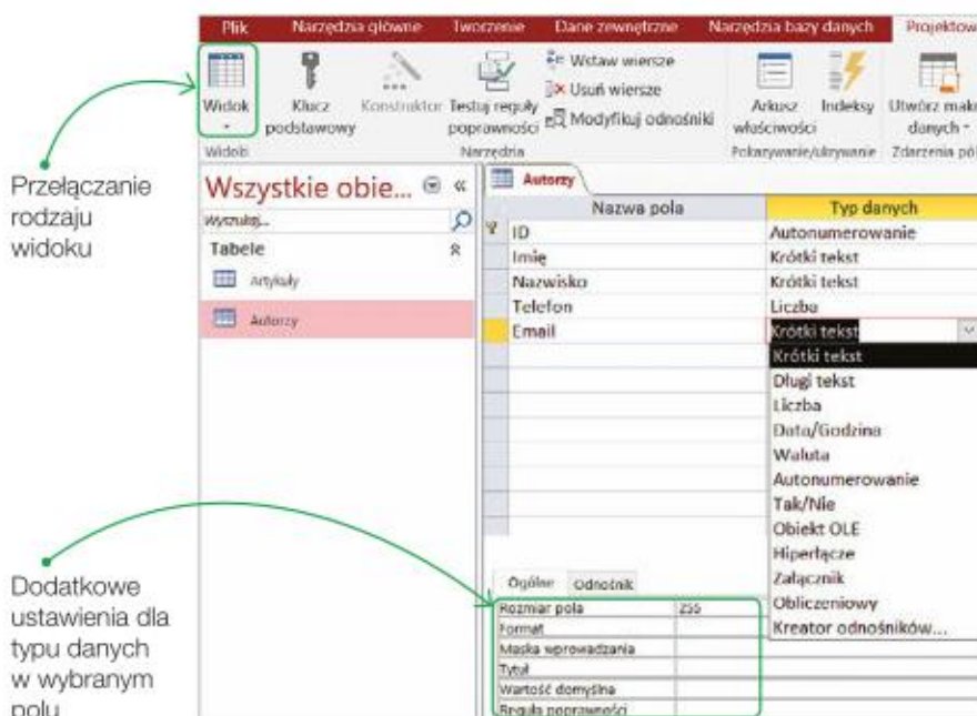
Rys. 4.6. Zarządzanie tabelą w Widoku projektu
