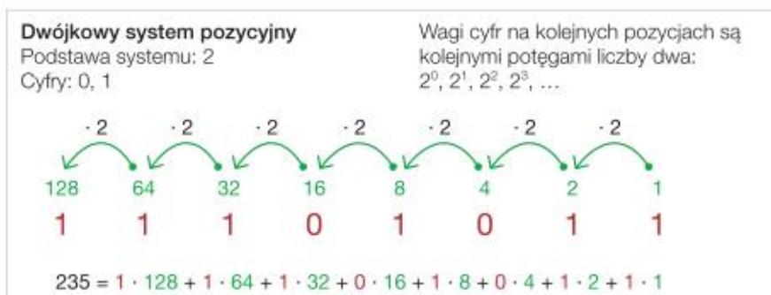
Rys. 7.2. Zapis dwójkowy liczby 235
