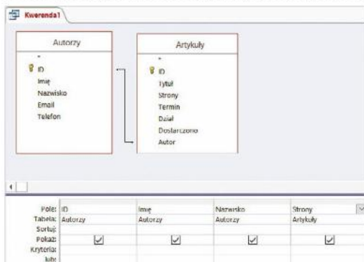
Rys. 4.16. Dodawanie tabel i wybieranie z nich pól tworzących kwerendę
