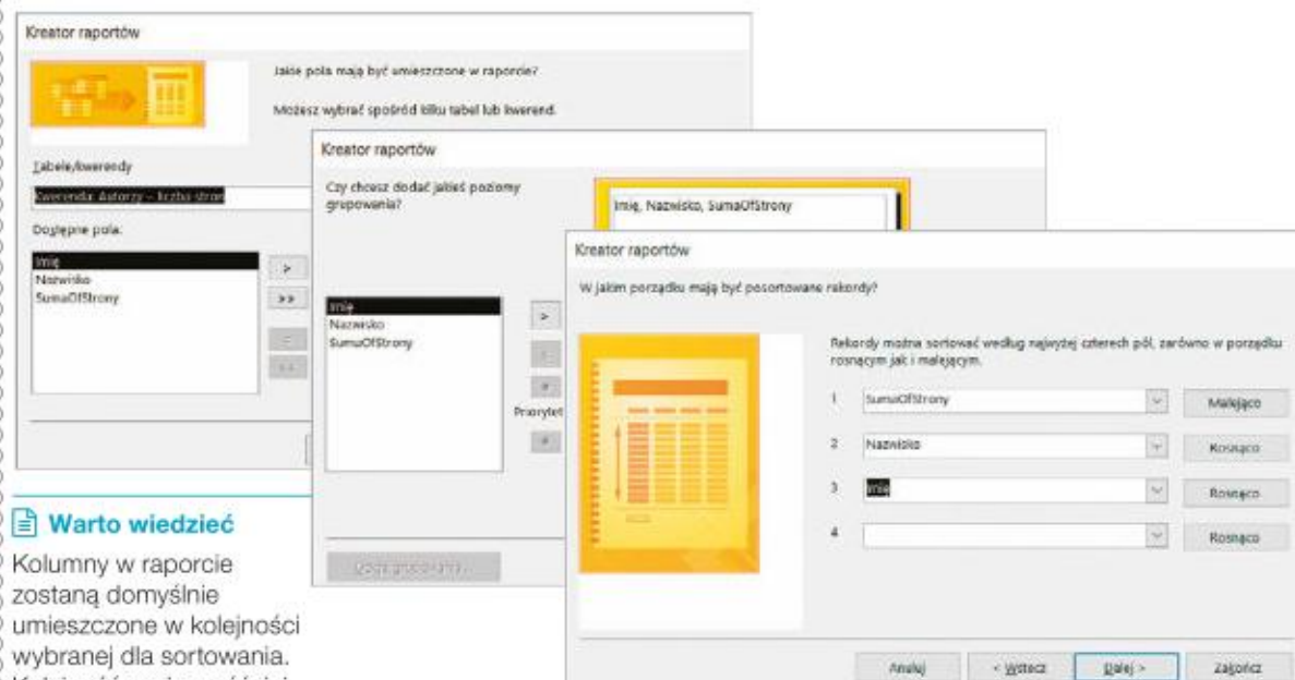
Rys. 4.19. Początkowe etapy tworzenia raportu z wykorzystaniem Kreatora raportów
