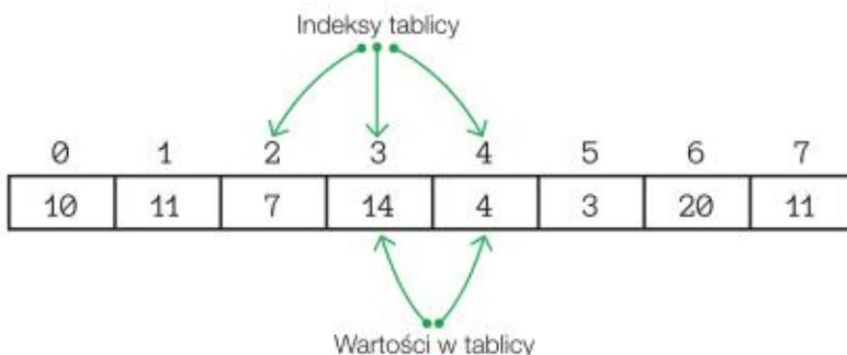
Rys. 7.10. Interpretacja graficzna tablicy 8-elementowej
