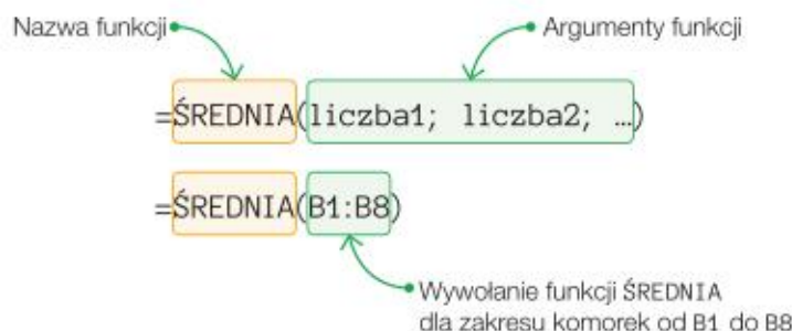
Rys. 1.4. Budowa funkcji ŚREDNIA
