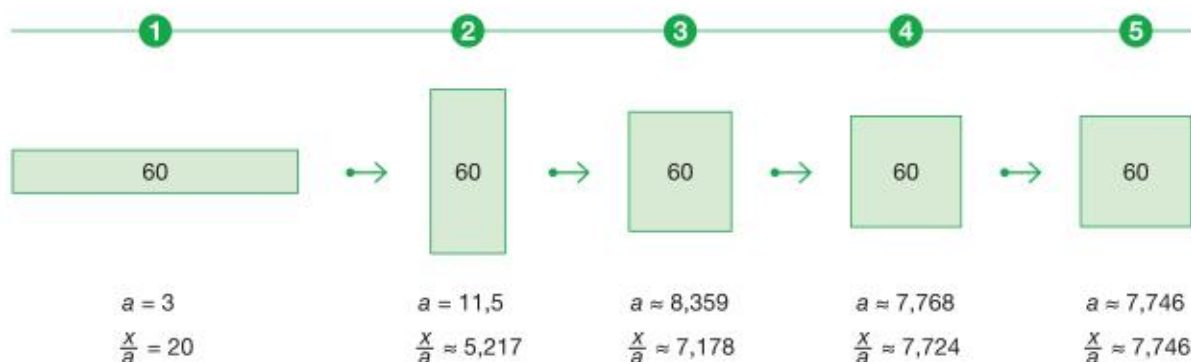
Rys. 5.3. Zastosowanie algorytmu Herona dla x = 60
