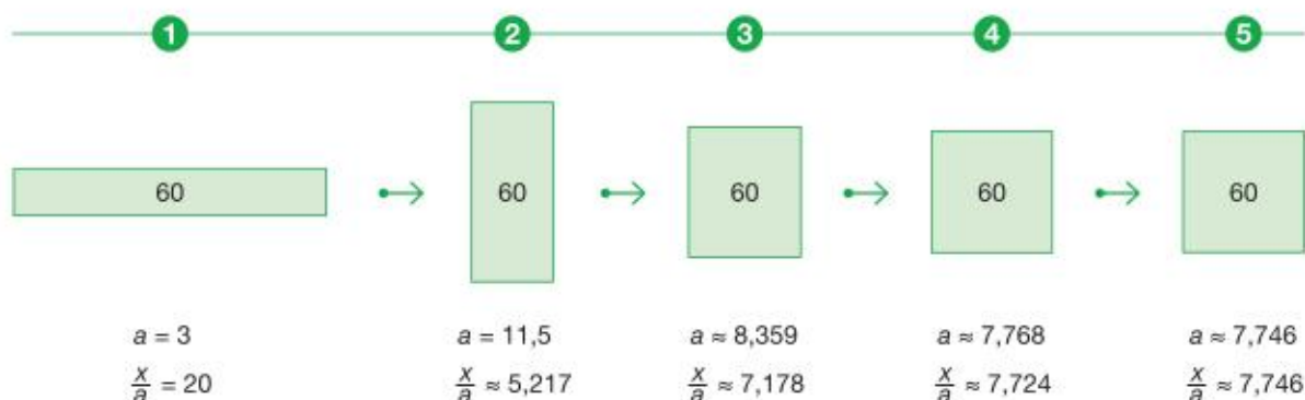
Rys. 10.3. Zastosowanie algorytmu Herona dla x = 60
