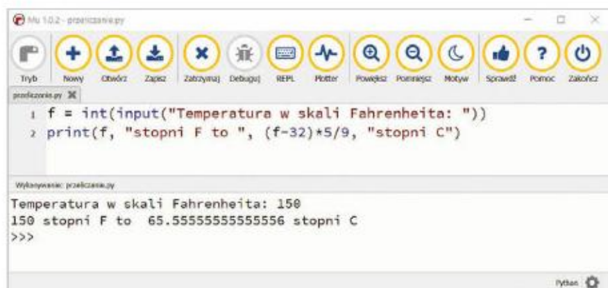
Rys. 10.7. Wywołanie programu Przeliczanie temperatury
