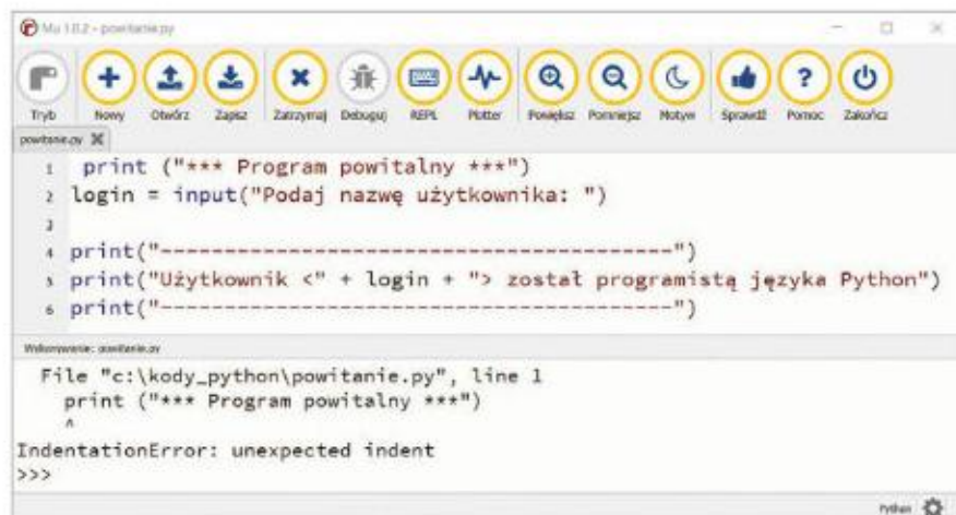
Rys. 10.5. Komunikat o błędzie składniowym – zbędna spacja przed instrukcją print
