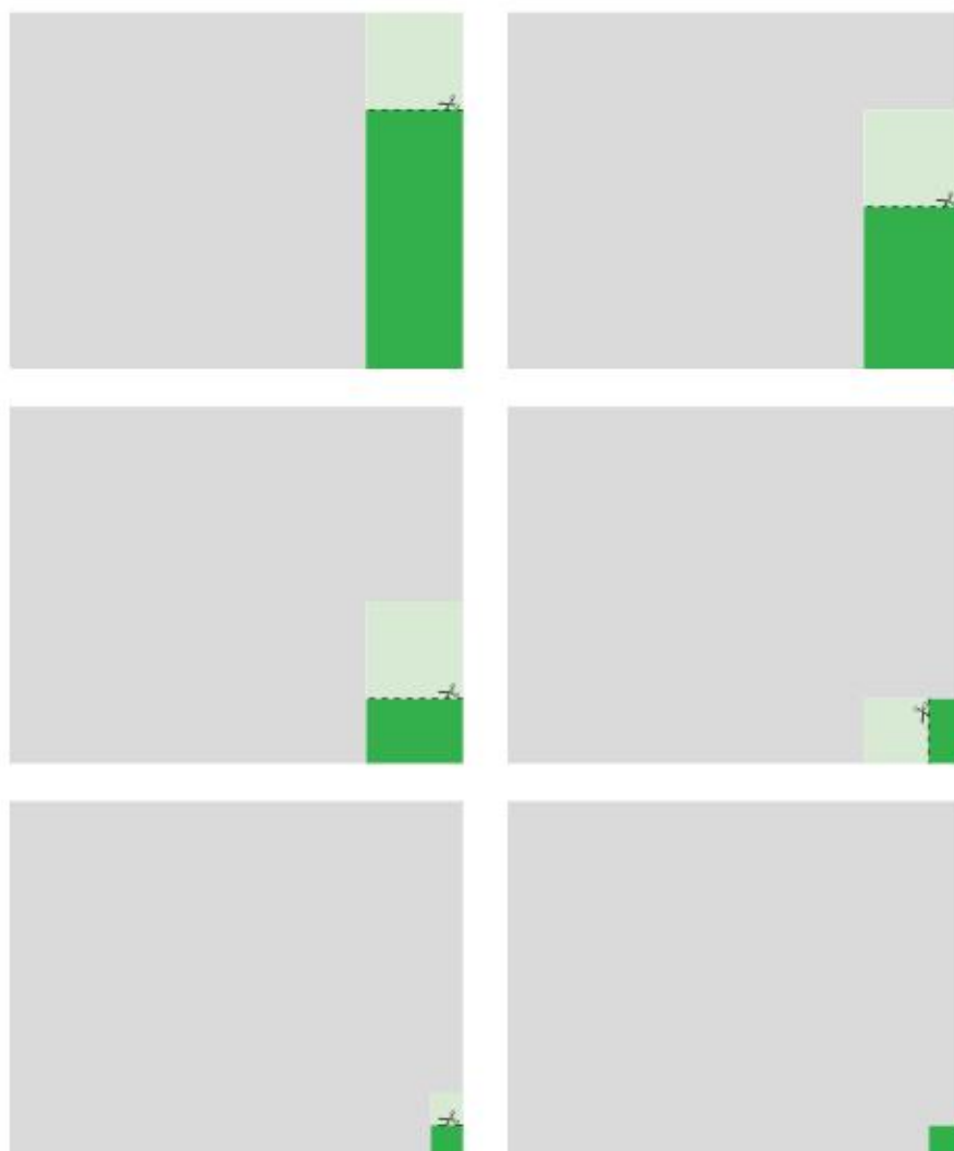
Rys. 9.4. Kolejne kroki wycinanki Euklidesa
