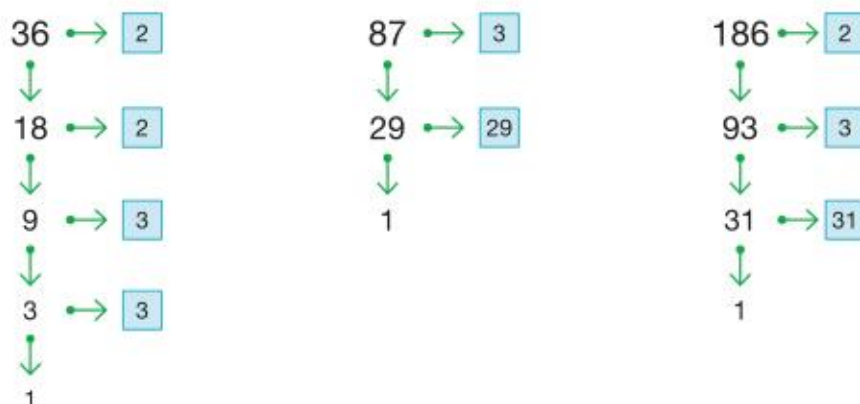
Rys. 13.2. Rozkład liczb 36, 87 i 186 na czynniki pierwsze
