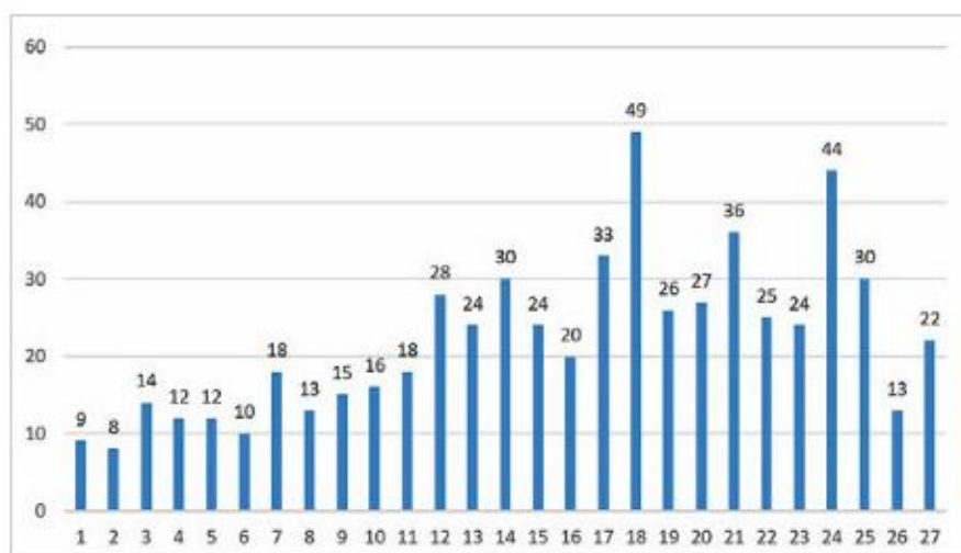
Rys. 1.21. Wykres rozkładu częstotliwości występowania liczb od 1 do 27 dla 100 losowań
