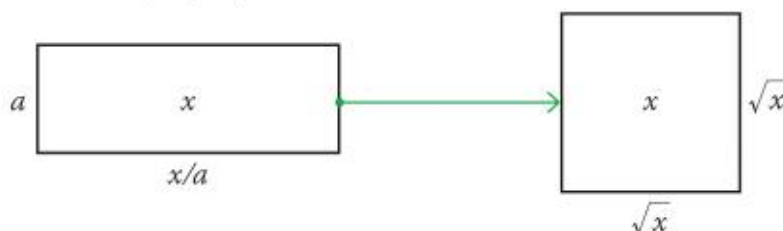
Rys. 10.2. Interpretacja geometryczna szukania przybliżenia liczby \sqrt{x}
