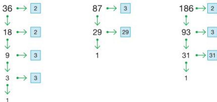
Rys. 8.2. Rozkład liczb 36, 87 i 186 na czynniki pierwsze
