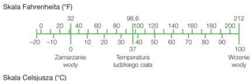
Rys. 10.6. Porównanie skali Fahrenheita ze skalą Celsjusza
