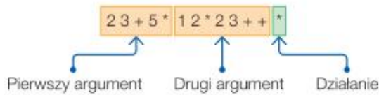
Rys. 1.5. Podział wyrażenia na argumenty wyznaczane rekurencyjnie
