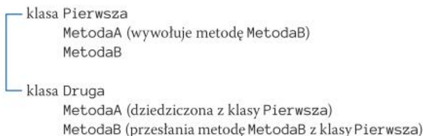
Rys. 13.4. Przykładowa hierarchia klas
