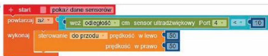
Rys. 19.13. Kod źródłowy programu Zatrzymanie przed przeszkodą
