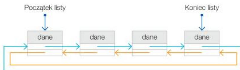
Rys. 3.4. Przykład listy dwukierunkowej cyklicznej złożonej z czterech elementów
