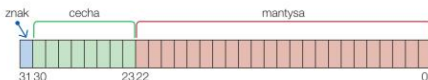
Rys. 5.4. Reprezentacja liczby zmiennoprzecinkowej pojedynczej precyzji
