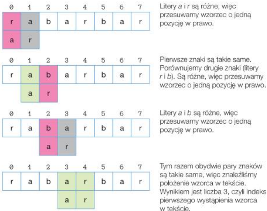
Rys. 11.1. Naiwne wyszukiwanie wzorca w tekście
