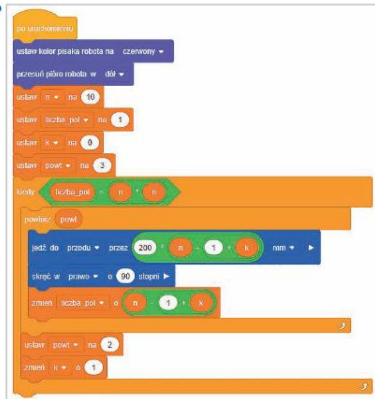
Rys. 19.25. Kod źródłowy programu Wszystkie pola planszy
