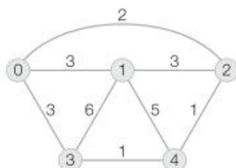
Rys. 4.2. Przykład grafu ważonego
