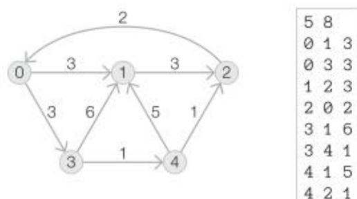
Rys. 4.11. Przykład skierowanego grafu ważonego i jego opis w pliku tekstowym
