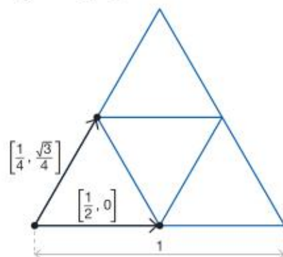
Rys. 10.17. Wektory przesunięcia w trójkącie Sierpińskiego
