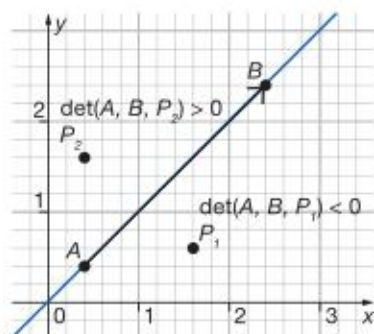
Rys. 9.8. Położenie punktów P_1 i P_2 względem prostej zawierającej wektor \overrightarrow{AB}
