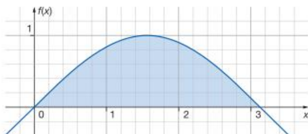
Rys. 8.4. Obszar zamknięty ograniczony wykresem funkcji f(x) = \sin x i osią OX w przedziale [0; \pi]
