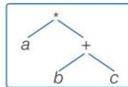
Rys. 1.2. Drzewo wyrażenia algebraicznego a b c + *
