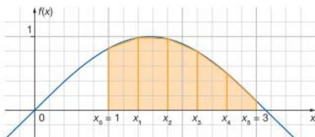
Rys. 8.7. Szukanie metodą trapezów przybliżenia pola obszaru ograniczonego funkcją f(x) = \sin x i osią OX w przedziale [1; 3] dla n = 5
