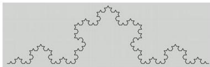
Rys. 10.9. Efekt działania skryptu rysującego krzywą Kocha stopnia 4
