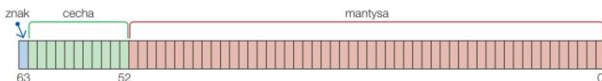
Rys. 5.5. Reprezentacja liczby zmiennoprzecinkowej podwójnej precyzji
