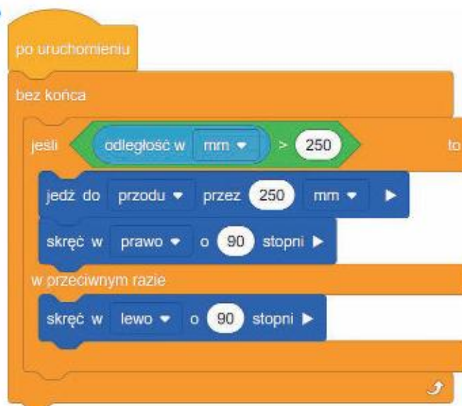
Rys. 19.27. Kod źródłowy programu Wyjście z labiryntu
