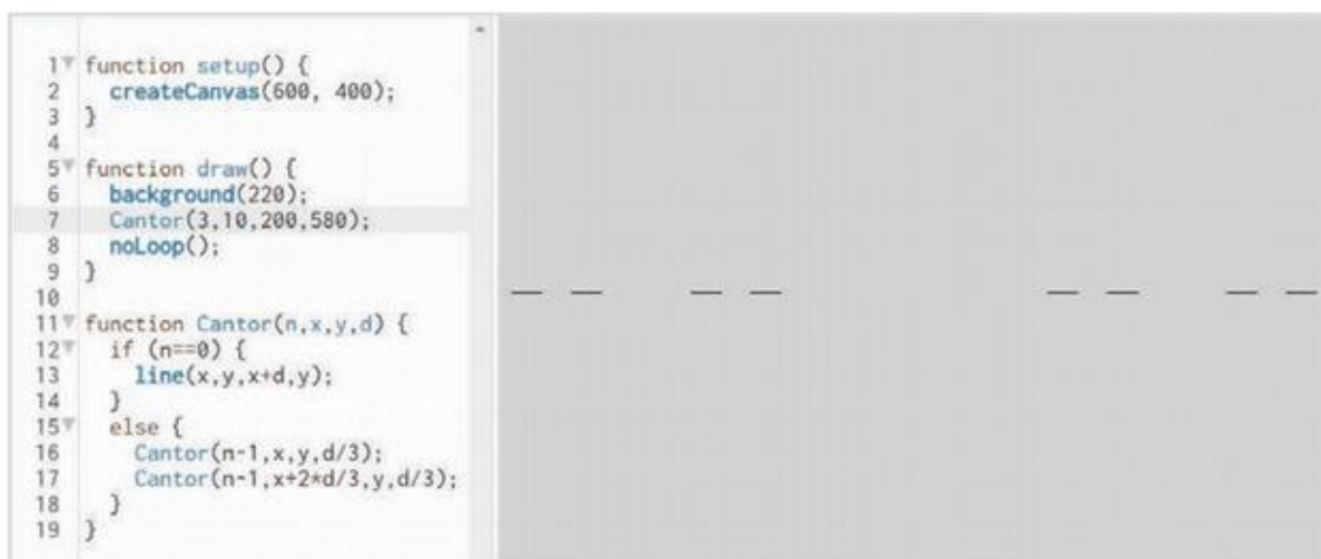
Rys. 10.3. Fragment okna edytora na stronie https://p5js.org z wywołaniem funkcji Cantor dla zbioru Cantora stopnia 3
