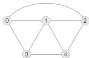
Rys. 4.1. Przykład grafu złożonego z pięciu wierzchołków i ośmiu krawędzi
