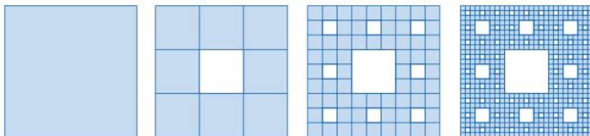
Rys. 10.14. Dywany Sierpińskiego stopni 0, 1, 2 i 3
