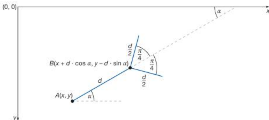
Rys. 10.13. Współrzędne punktów oraz kąty w drzewie binarnym
