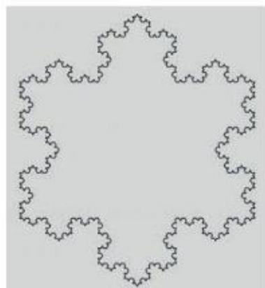
Rys. 10.11. Płatek Kocha stopnia 4
