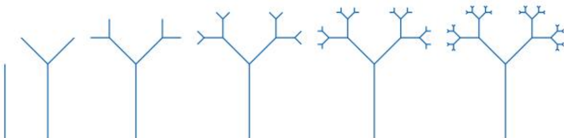
Rys. 10.12. Drzewa binarne stopni 0, 1, 2, 3, 4 i 5
