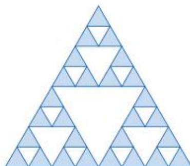
Rys. 10.16. Trójkąt Sierpińskiego stopnia 3
