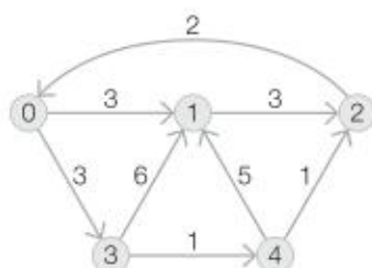
Rys. 4.3. Przykład grafu skierowanego
