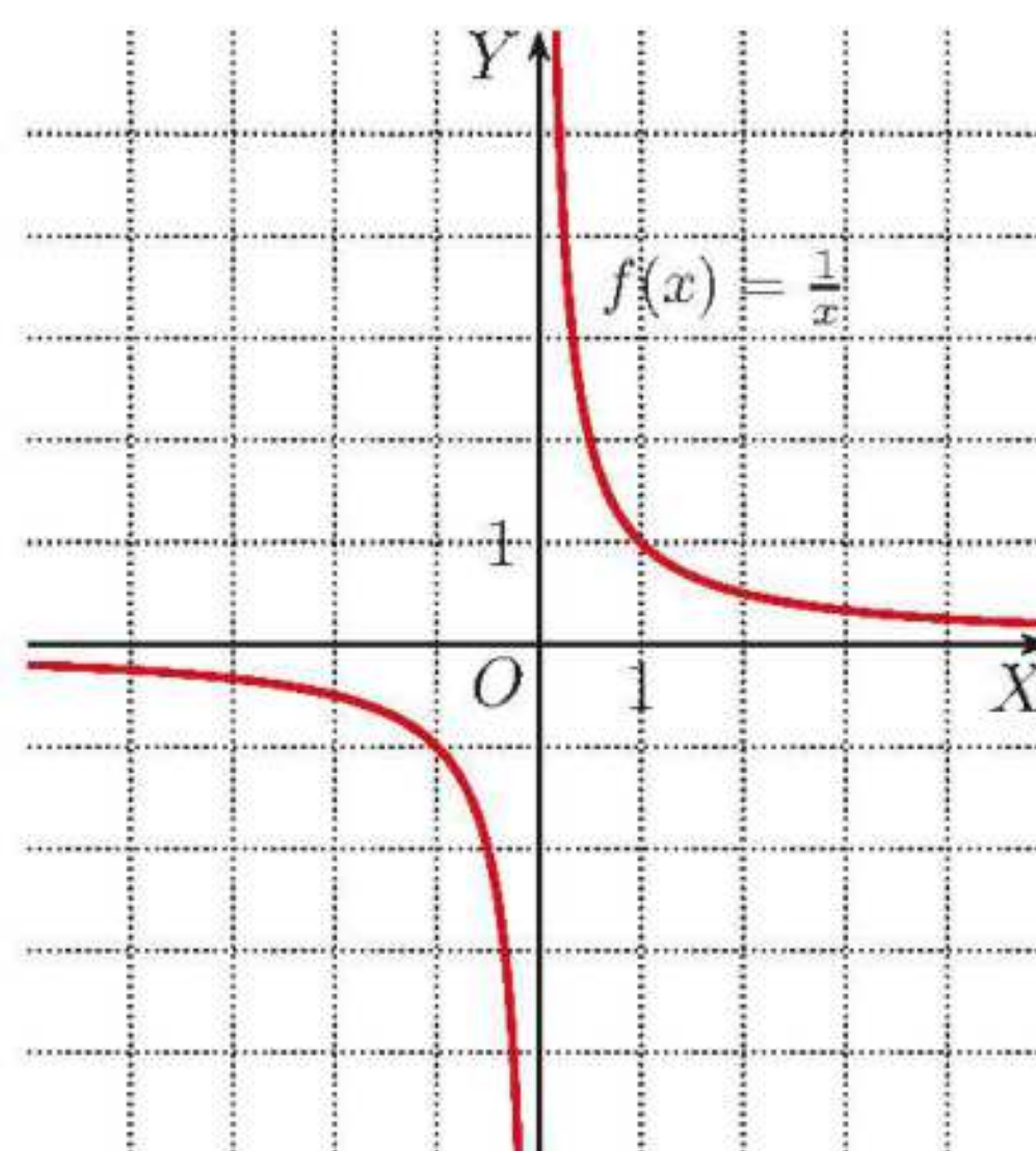
Hiperbola składa się z dwóch gałęzi.
