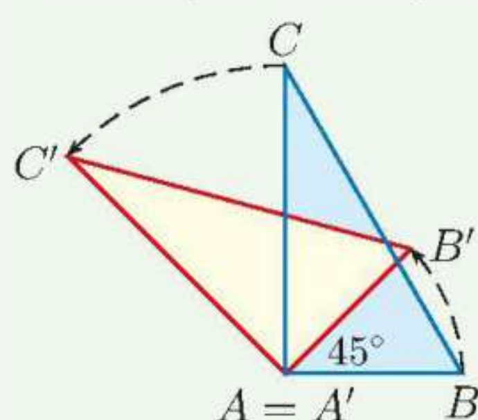
Obrót trójkąta ABC dookoła punktu A o kąt 45^\circ .
