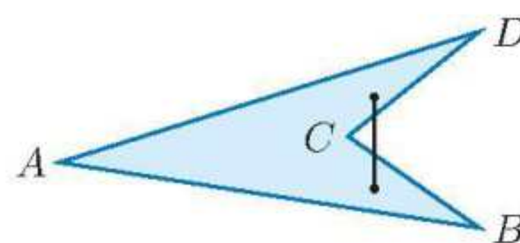
Czworokąt ABCD nie jest wypukły.
