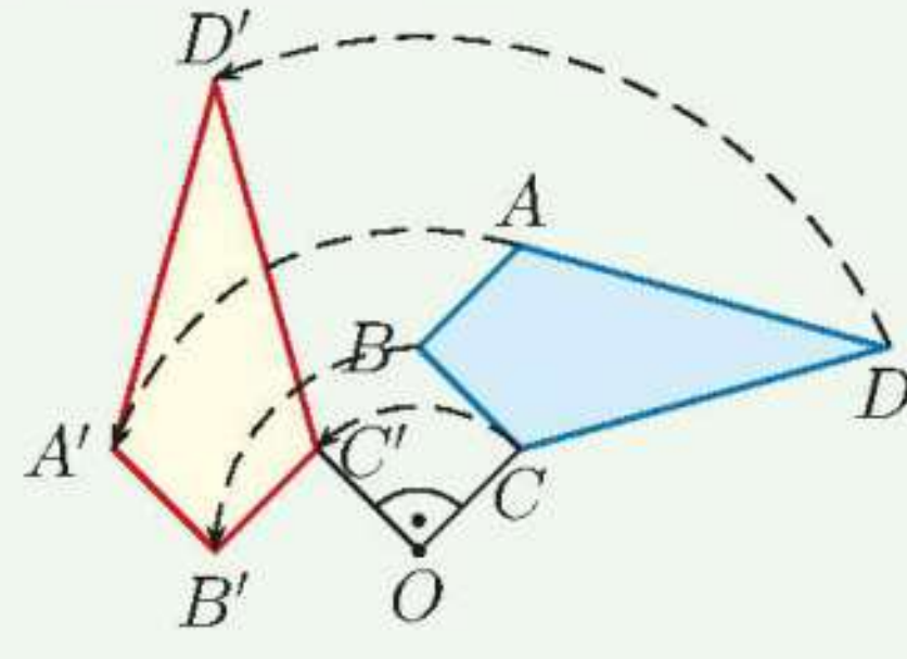
Obrót deltoidu ABCD dookoła punktu O o kąt 90^\circ .
