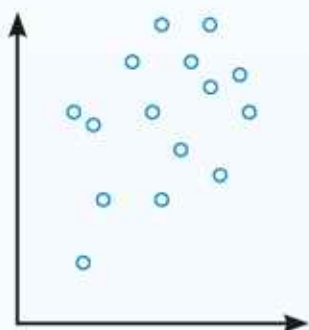
słaba korelacja dodatnia, r = 0,4
