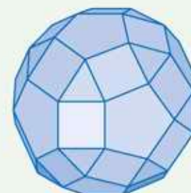
dwudziesto- -dwunastościan rombówý mały
