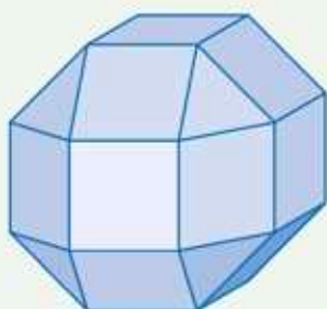
sześćcio-ośmiościan rombówý mały
