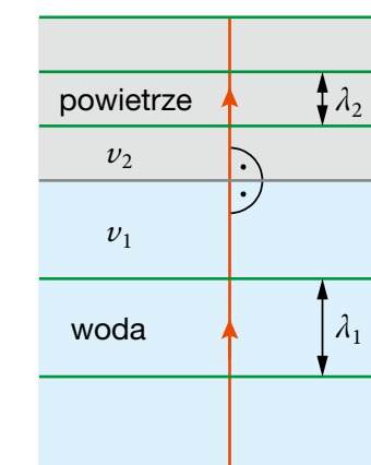
Rys. 12.13. Przejęcie fali dźwiękowej z wody do powietrza
