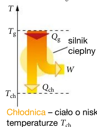
Rys. 8.19. Przepływ energii w silniku cieplnym
