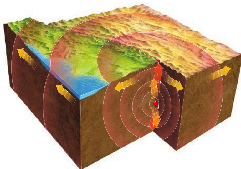
Rys. 11.10. Podłużna fala sejsmiczna porusza się z prędkością 4-8 \frac{\text{km}}{\text{s}} , a poprzeczna z prędkością 2-5 \frac{\text{km}}{\text{s}}
