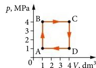
Rys. 8.20. Cykl termodynamiczny
