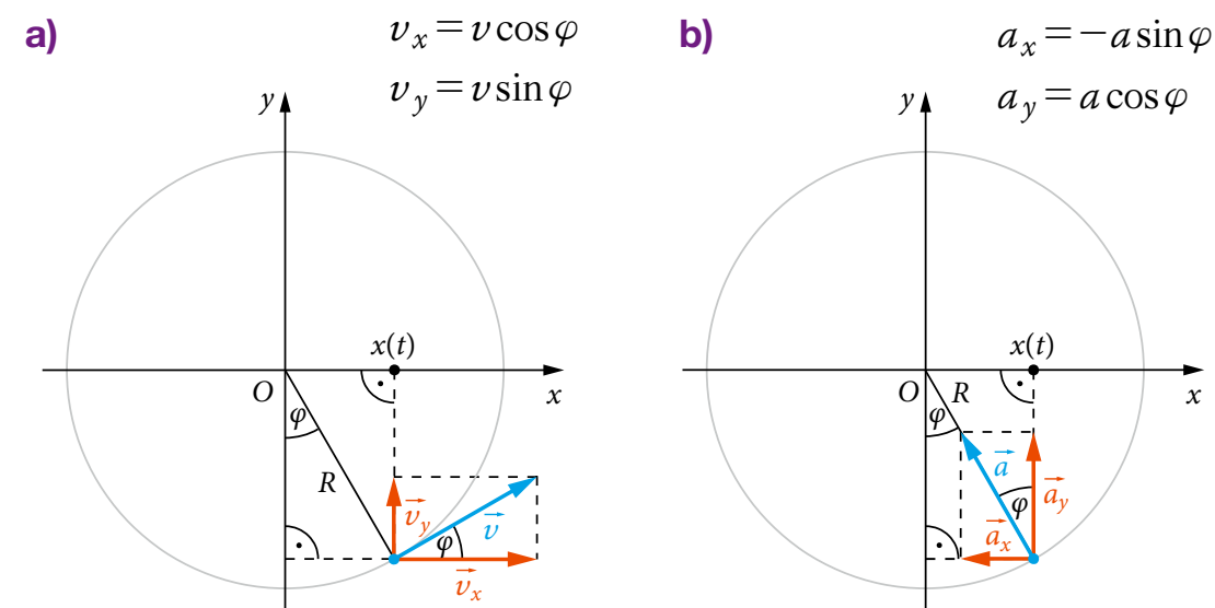
Rys. 10.13. Rozkład wektorów: prędkości liniowej (a) i przyspieszenia dośrodkowego (b) w ruchu po okręgu na składowe: równoległą do osi x i równoległą do osi y
