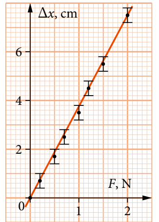
Rys. 10.5. Wykres zależności wydłużenia sprężyny od ciężaru obciążenia
