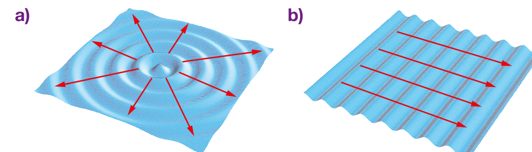
Rys. 11.22. Promienie fal rozchodzących się na powierzchni wody: a) fal kulistych, b) fal płaskich
