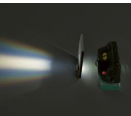
Rys. 12.34. Światło białe przechodzące przez siatkę dyfrakcyjną
