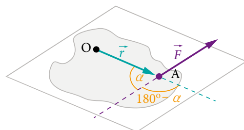
Rys. 9.15. Zaznaczamy kąty między promieniem wodzącym i siłą
