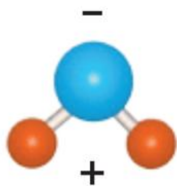
model cząsteczki wody
