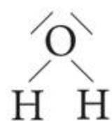
wzór elektronowy kreskowy
